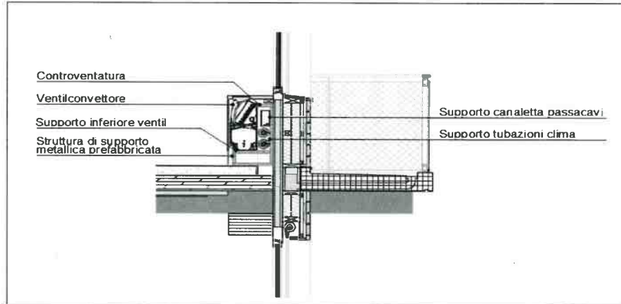
SUPPORTO VENTILCONVETTORE TIPO 1.2
