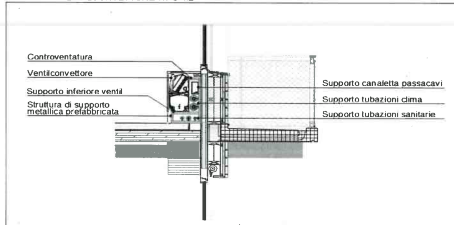
SUPPORTO VENTILCONVETTORE TIPO 1.2
