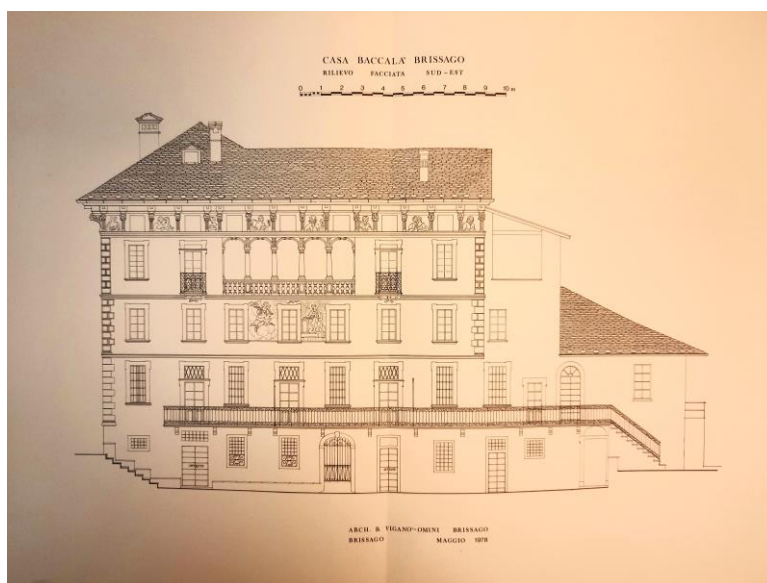
Brissago, casa Baccalà, rilievo architetto Bruno Viganò-Omini, 1978
