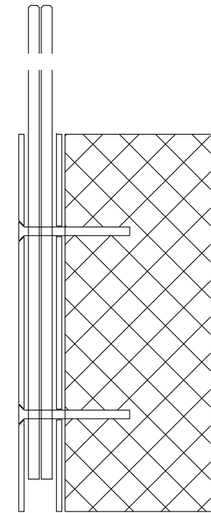
SEZIONE TIPO 1:5
