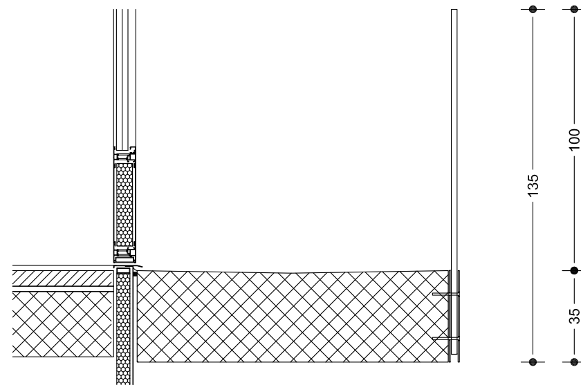
SEZIONE 1-1 1:20
