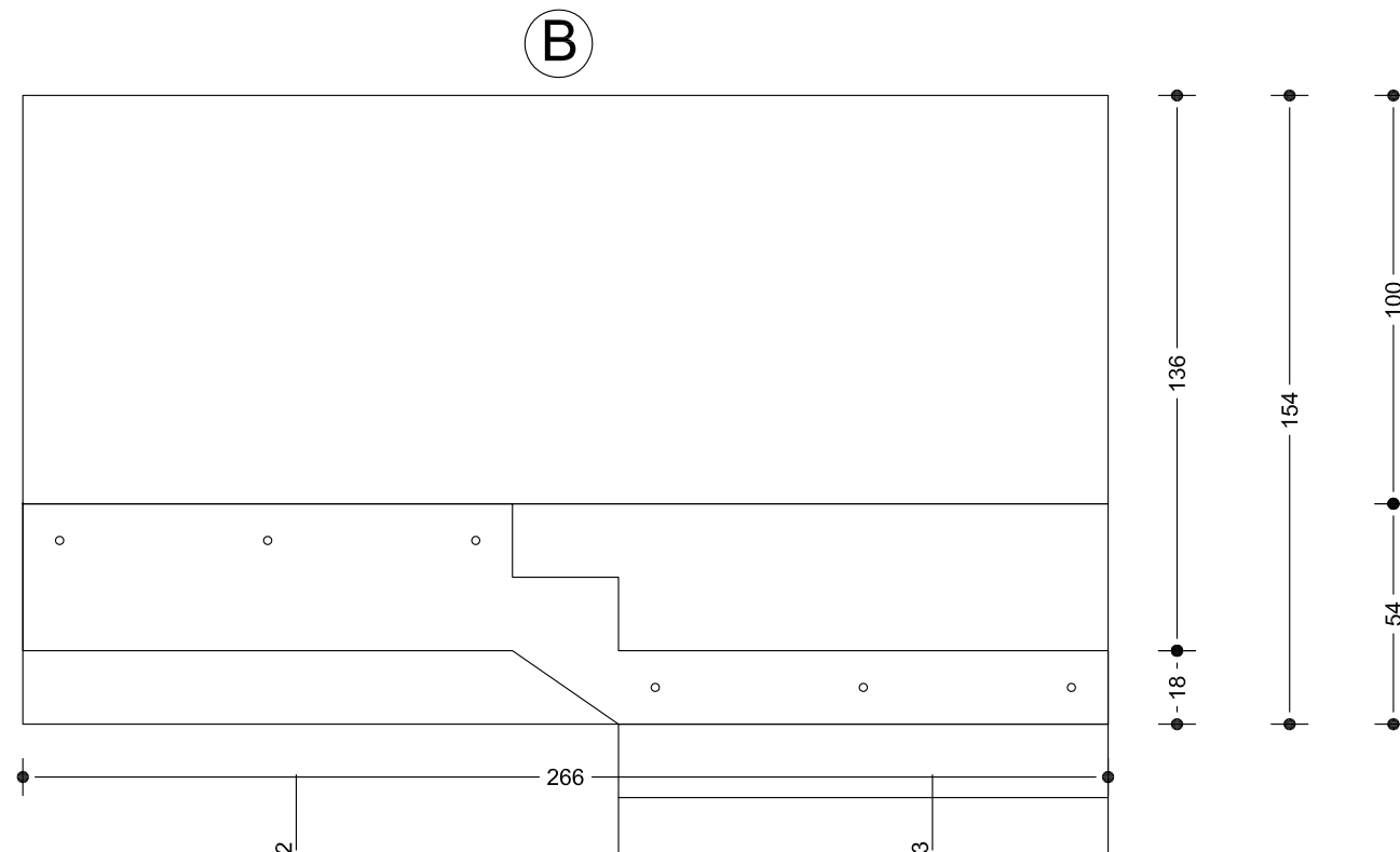
SEZIONE 3-3 1:20
