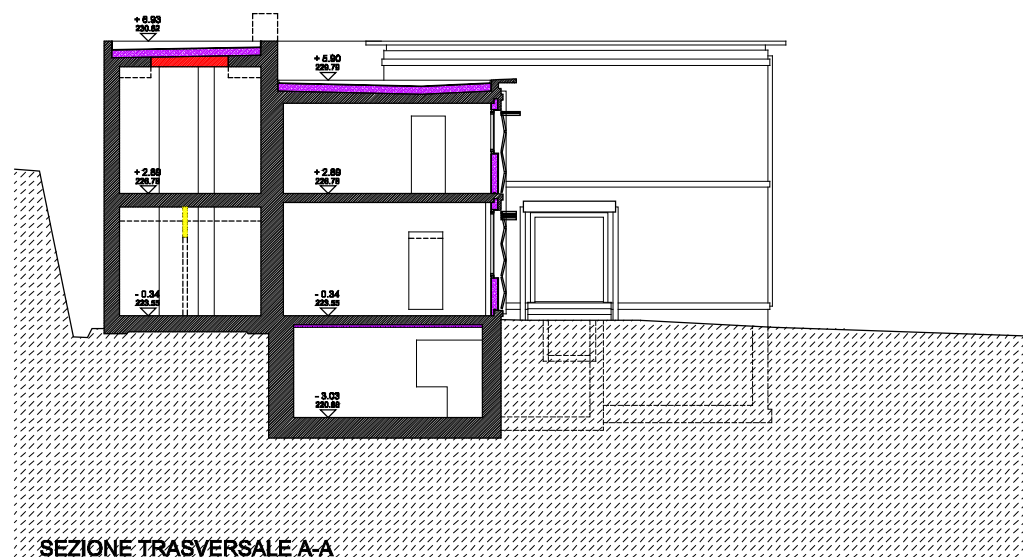
SEZIONE TRASVERSALE A-A
