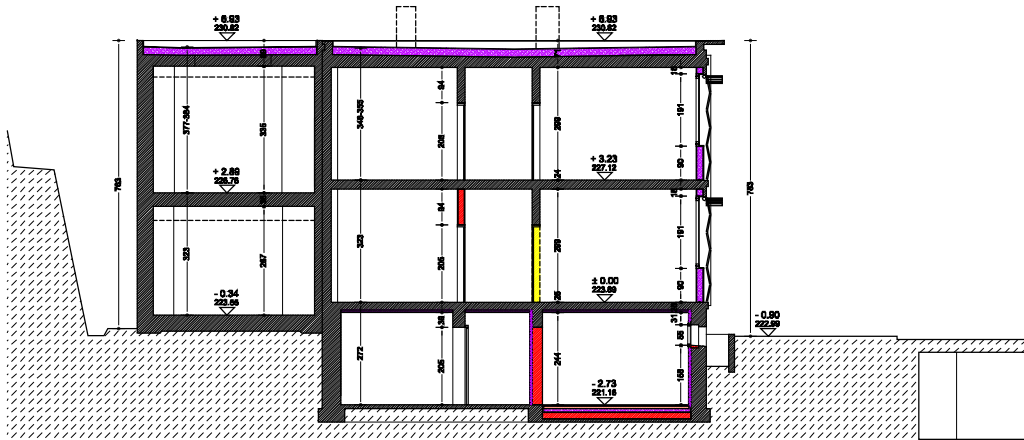
SEZIONE TRASVERSALE D-D
