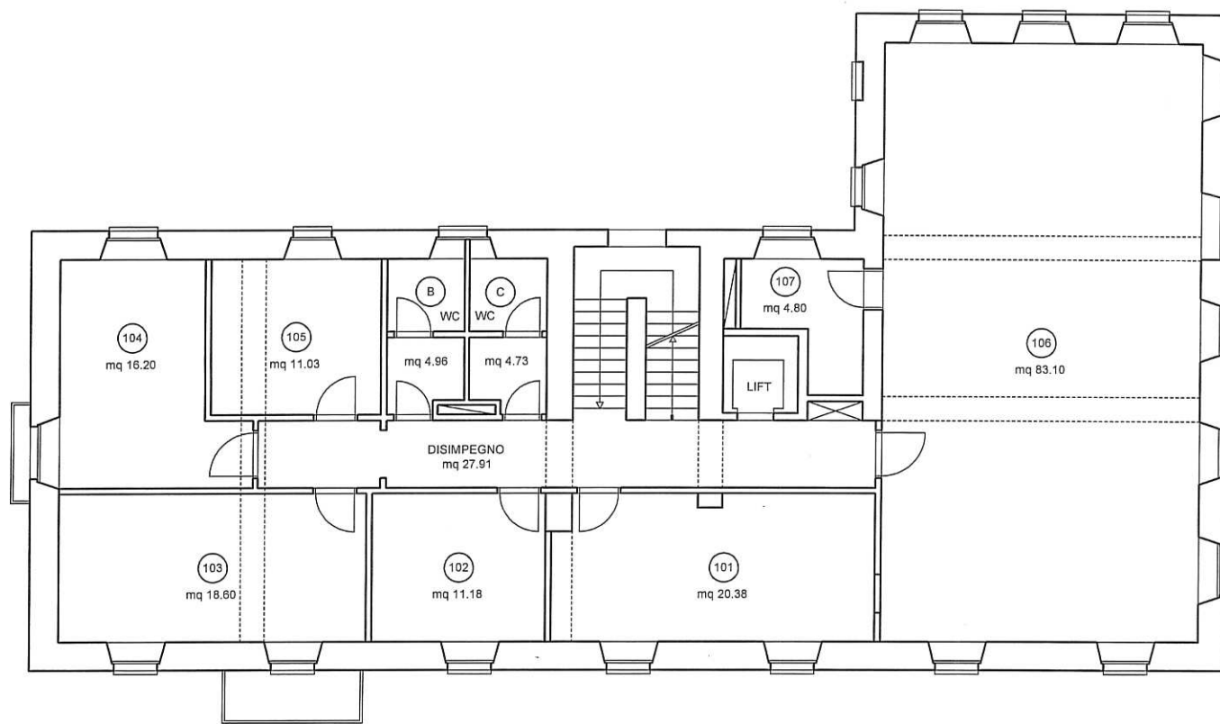
PIANTA PRIMO PIANO
