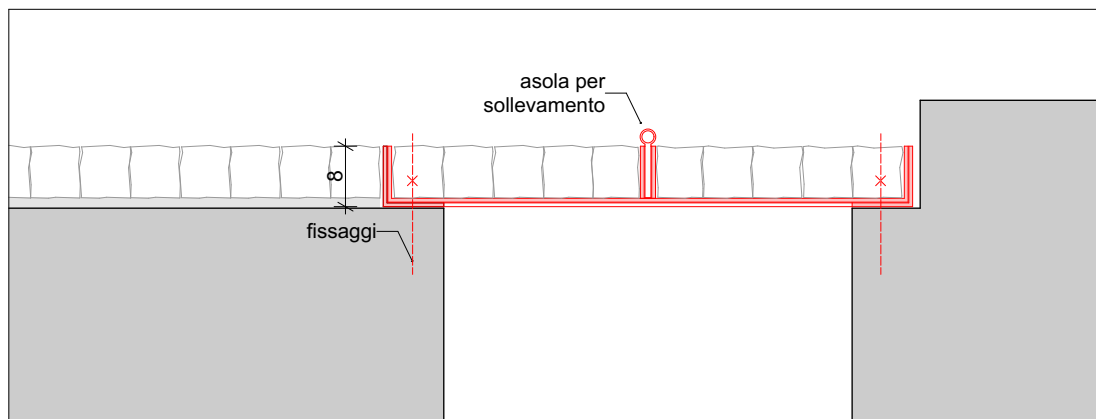
SEZIONE 1
