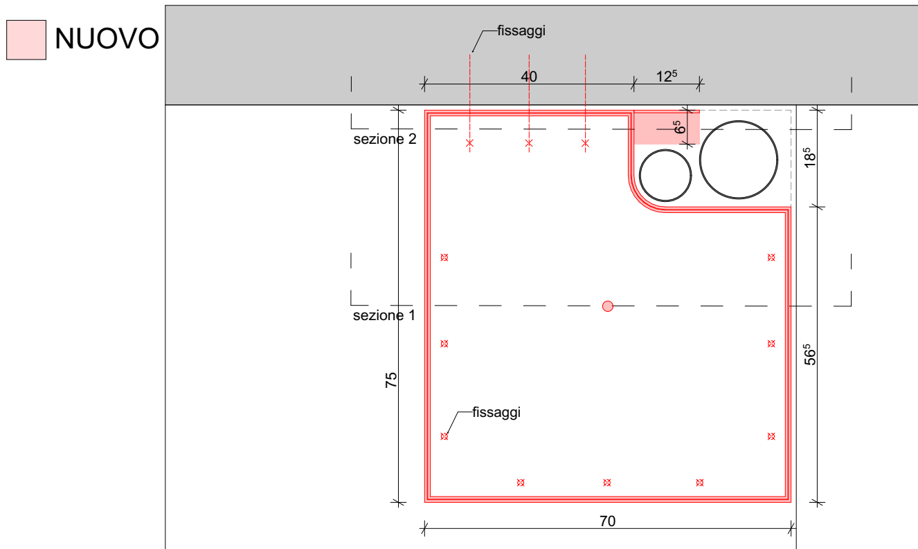
PIANTA
