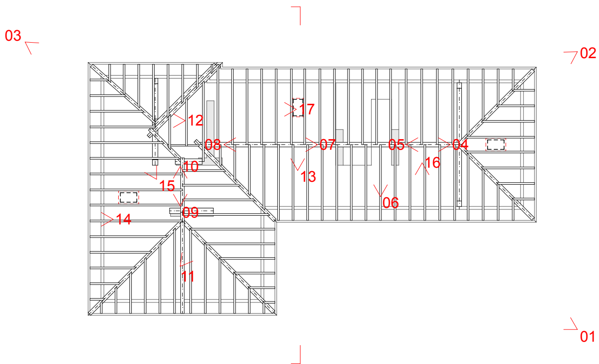
Pianta sottotetto 1:200 (con in evidenza i punti di scatto)
