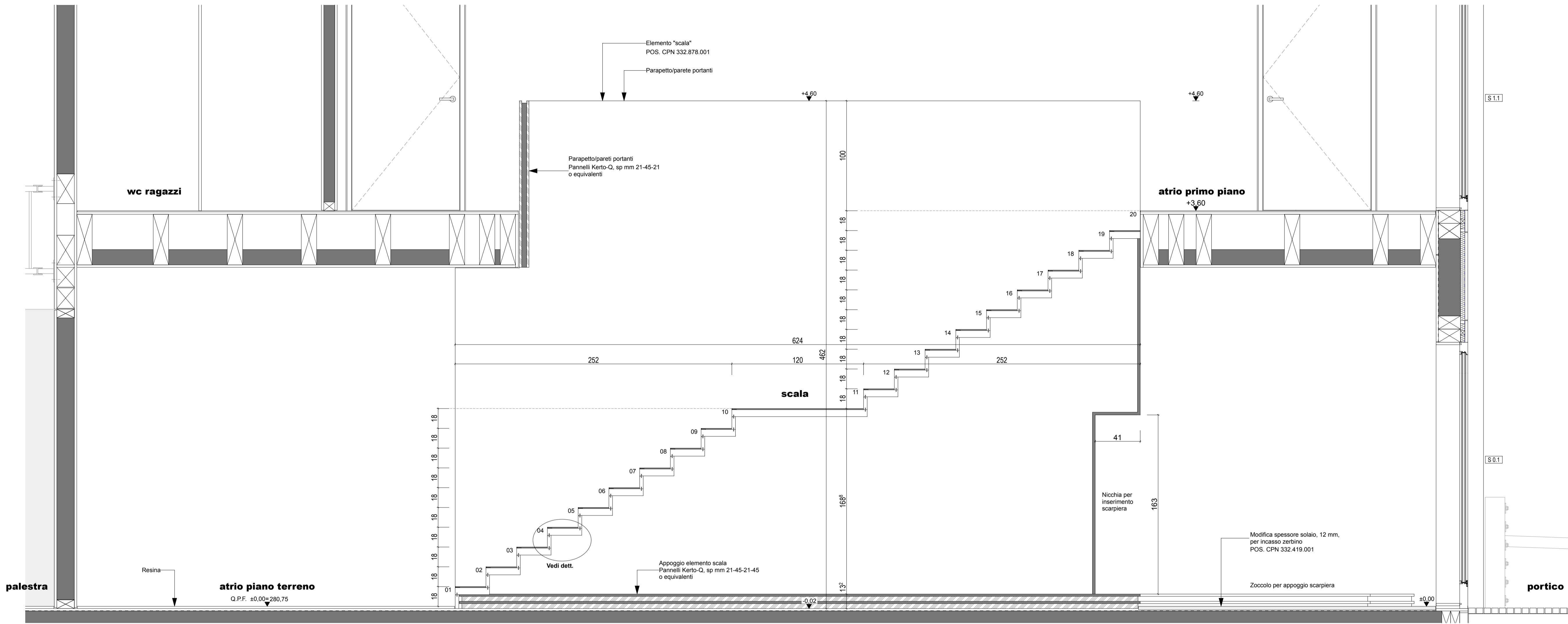
ELEMENTO SCALA - SEZIONE
