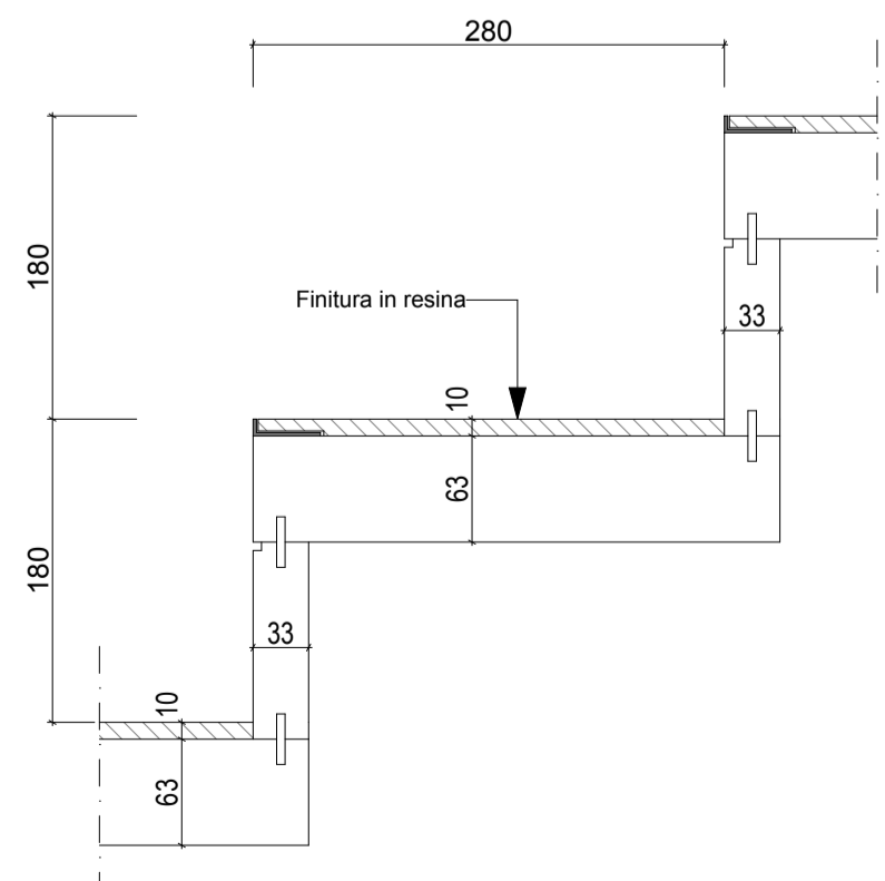
DETTAGLIO GRADINO - SEZIONE 1 : 5
