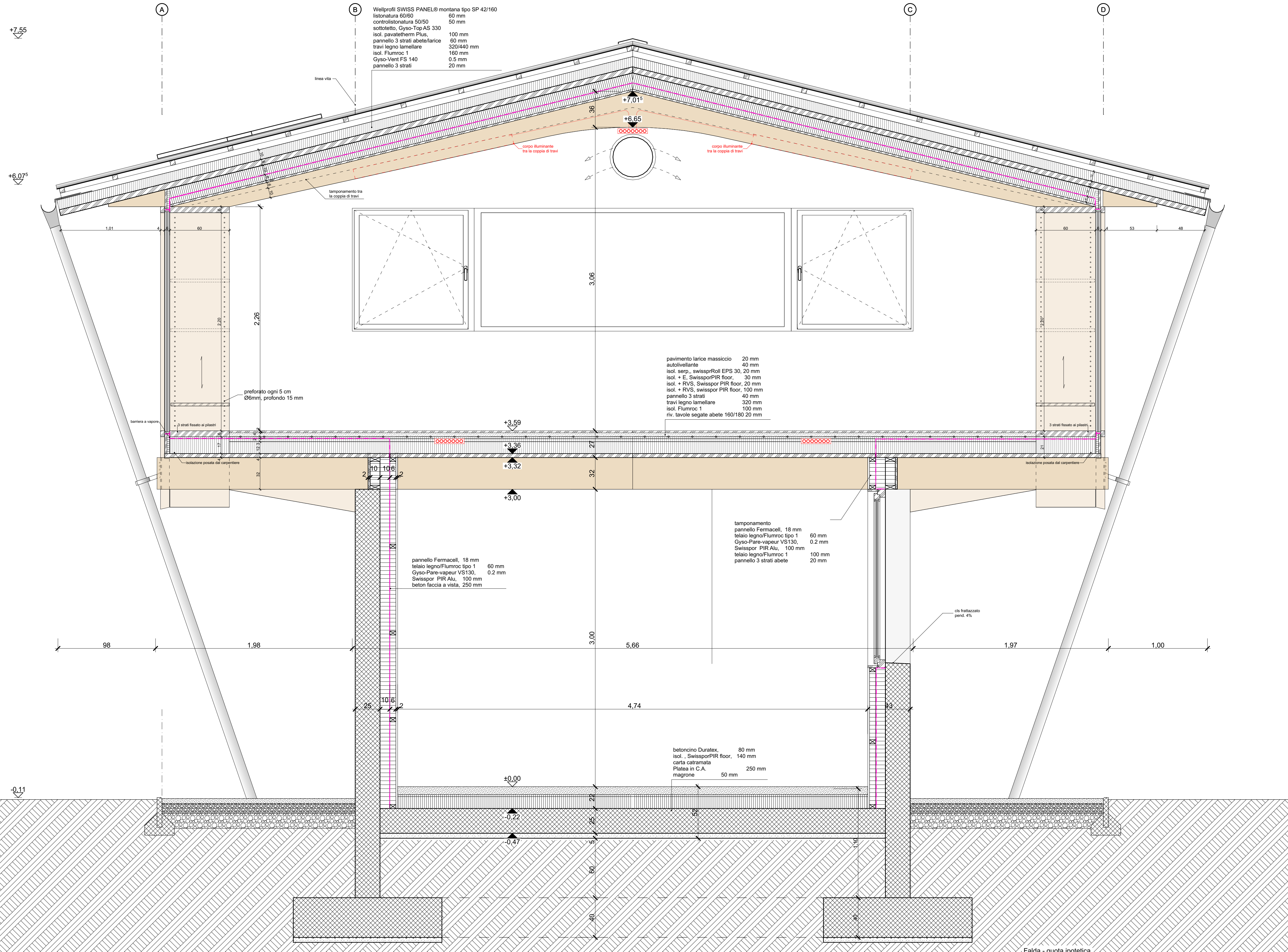
SEZIONE SALA 1:20
