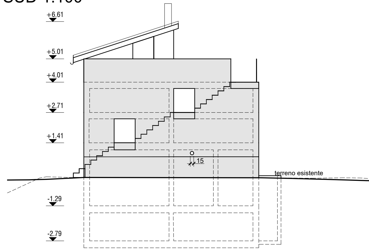
VISTA SUD 1:100
