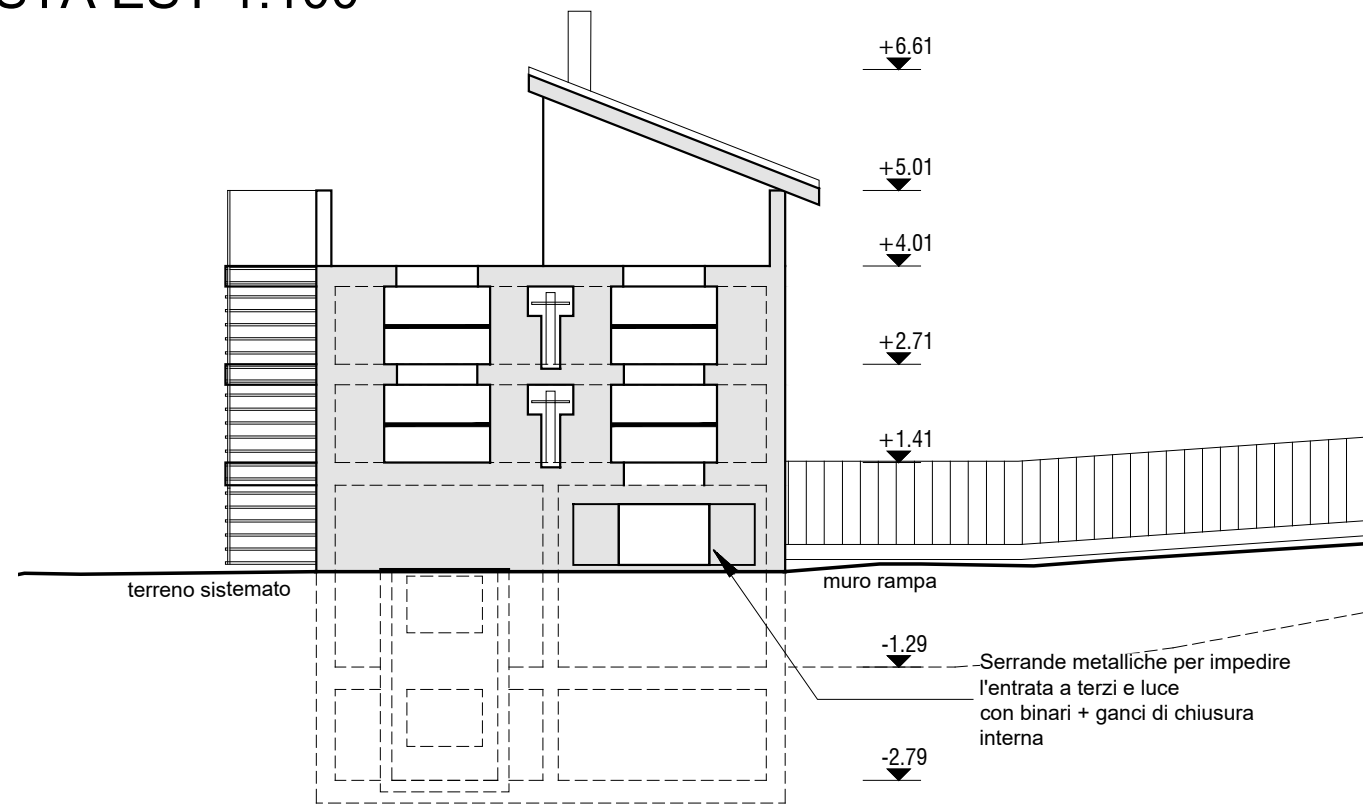
VISTA EST 1:100
