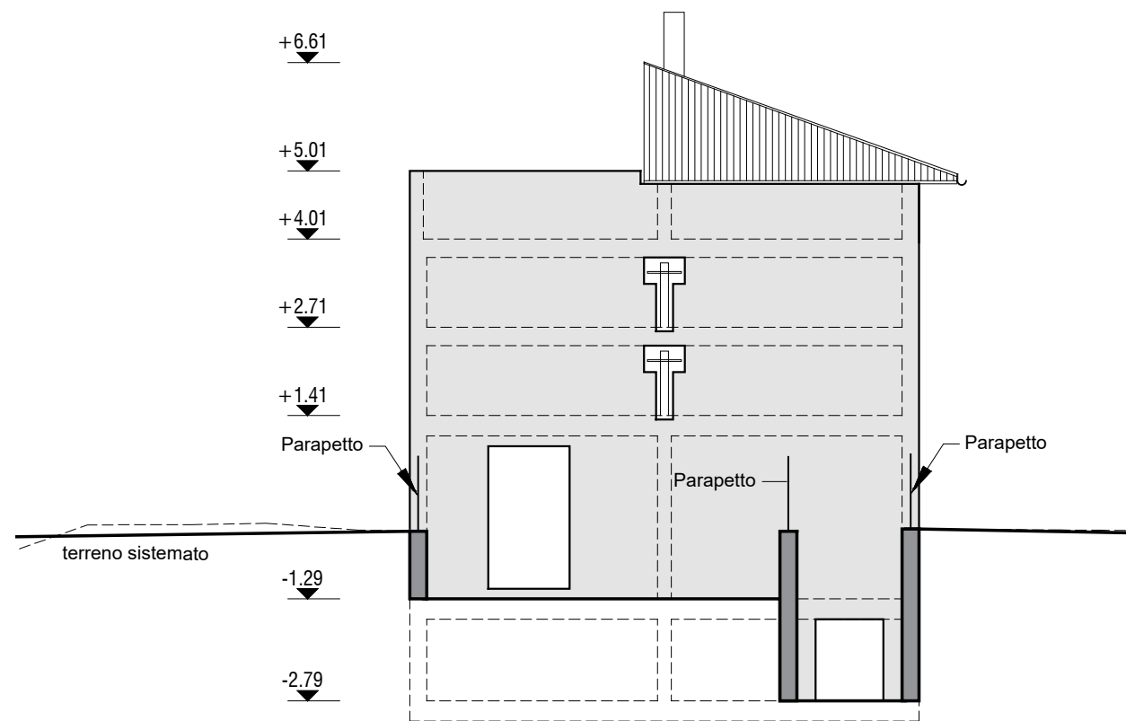
VISTA NORD 1:100
