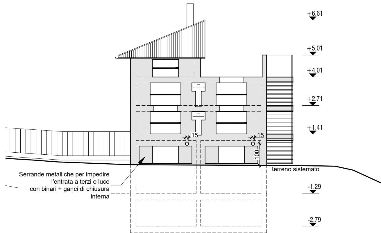
VISTA OVEST 1:100
