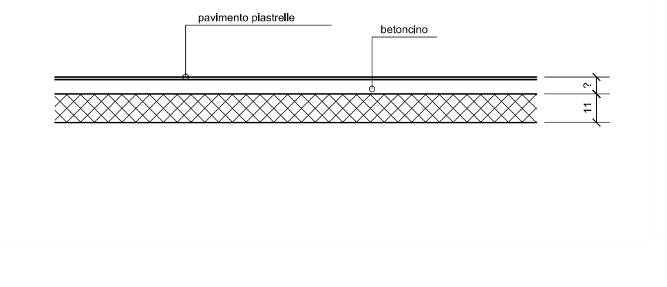
SONDAGGIO 10 Sezione soletta 1:20
