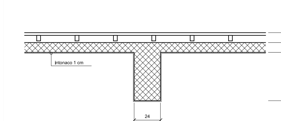
SONDAGGIO 8 Sezione trave/soletta 1:20
