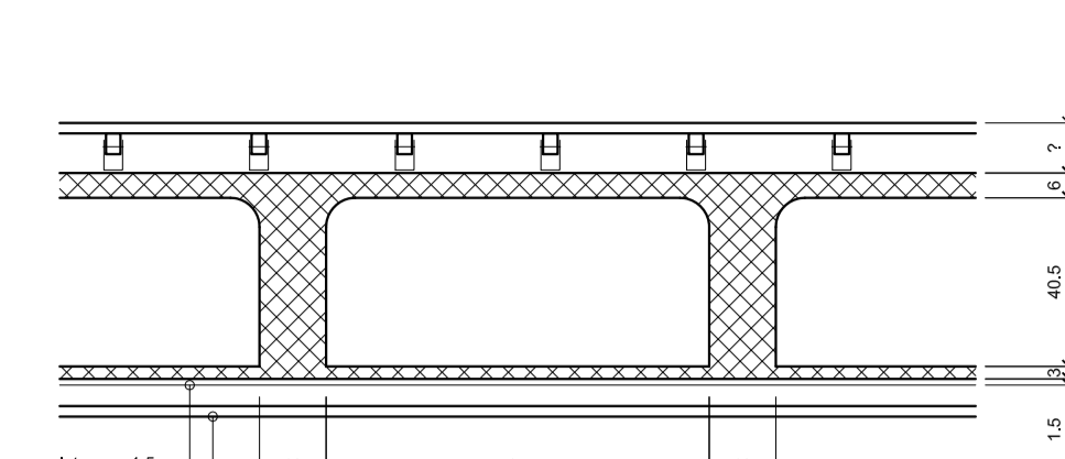
SONDAGGI 5 + 1 Sezione trave/soletta 1:20
