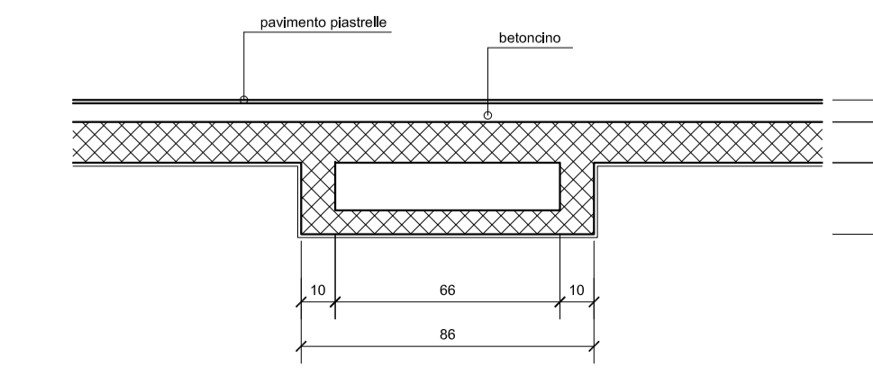
SONDAGGIO 12 Sezione trave/soletta 1:20
