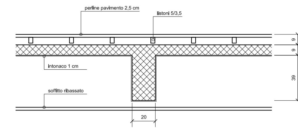
SONDAGGIO 3 / 3 Sezione trave/soletta 1:20
