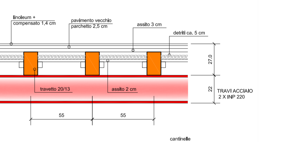
SONDAGGIO 4 Sezione soletta 1:20
