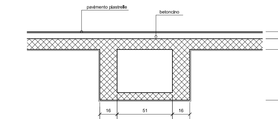
SONDAGGIO 13 Sezione trave/soletta 1:20
