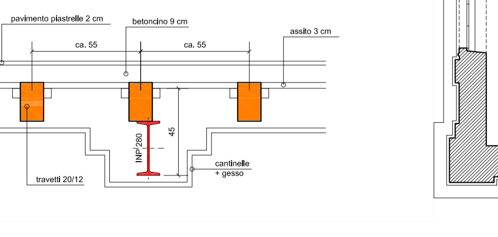
SONDAGGIO 7 Sezione soletta 1:20
