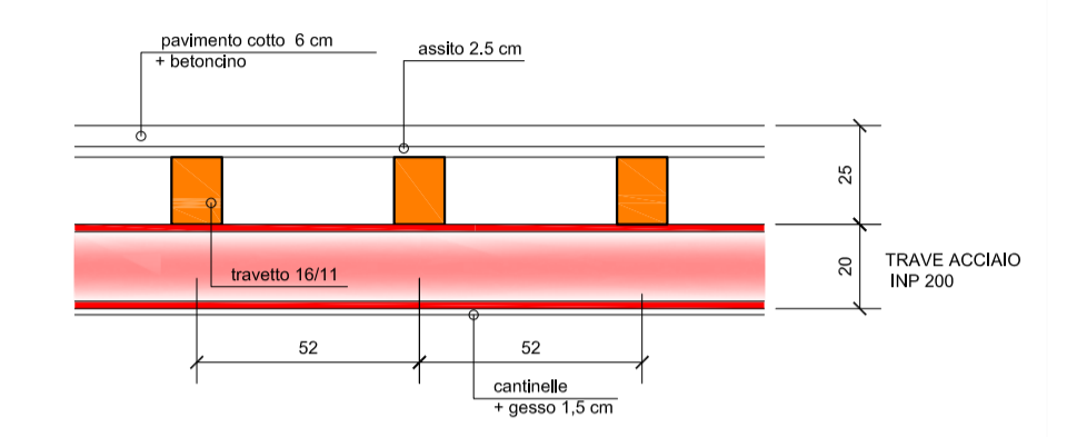
SONDAGGIO 43 Sezione soletta 1:20
