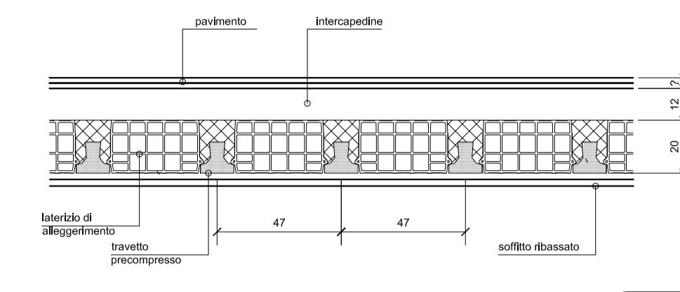
SONDAGGIO 5 / 6 Sezione soletta 1:20
