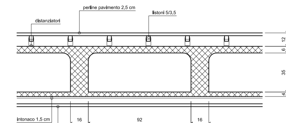
SONDAGGIO 4 / 4 + 11 Sezione trave/soletta 1:20
