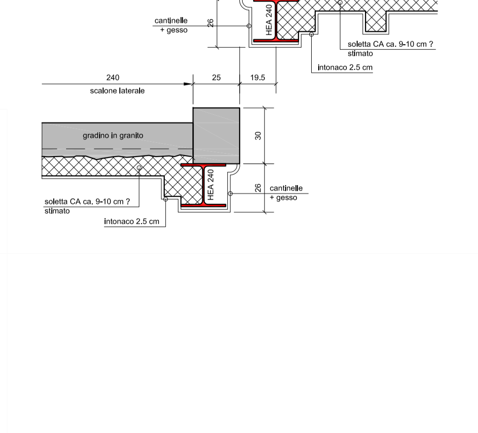
SONDAGGIO 8 Sezione scala 1:20
