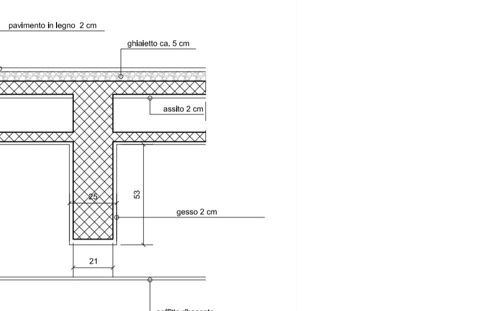
SONDAGGIO 3 Sezione trave 1:20
