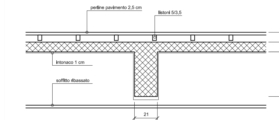
SONDAGGIO 1.1 Sezione trave/soletta 1:20
