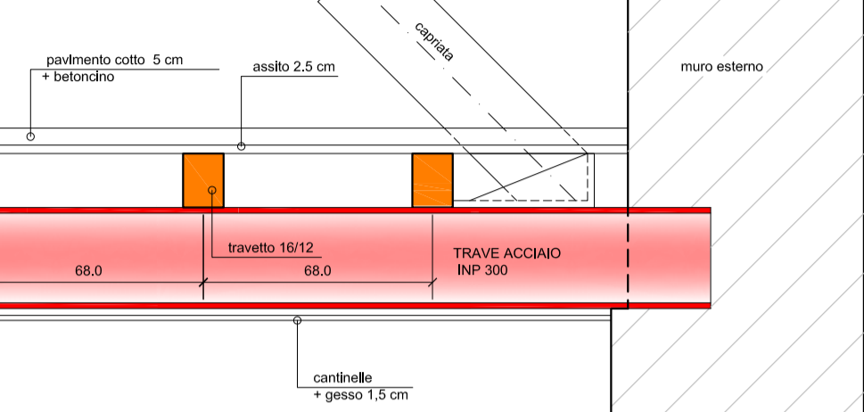
SONDAGGIO 5 Sezione soletta 1:20
