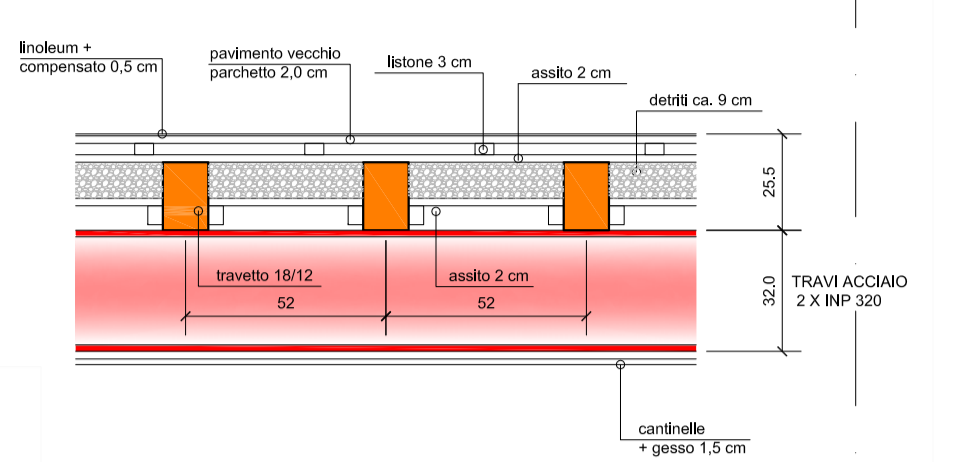
SONDAGGIO 3 Sezione soletta 1:20
