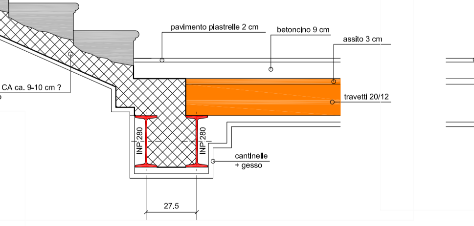
SONDAGGIO 6 Sezione trave 1:20
