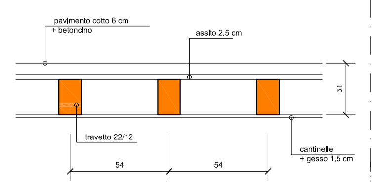
SONDAGGIO 42 Sezione soletta 1:20
