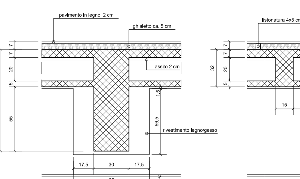
SONDAGGIO 2 Sezione trave 1:20
