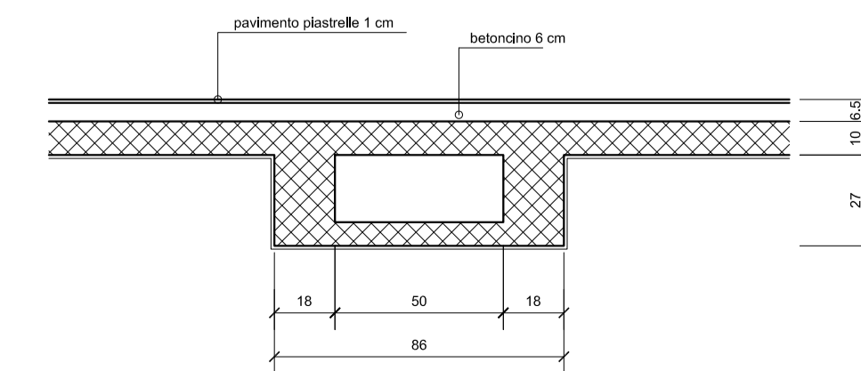
SONDAGGIO 1 / 9 Sezione trave/soletta 1:20
