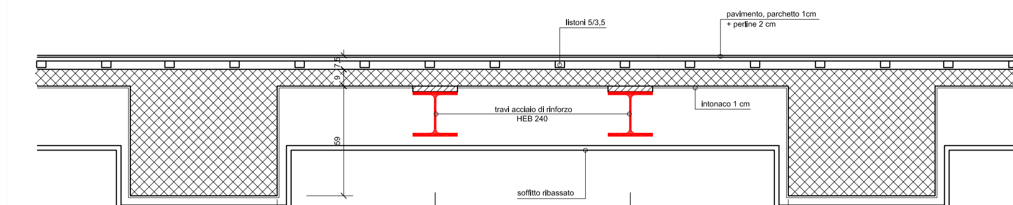
SONDAGGIO 6 / 7 Sezione trave/soletta 1:20
