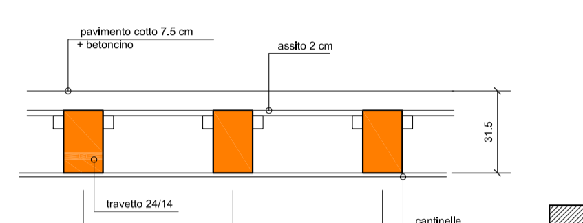
SONDAGGIO 32 Sezione soletta 1:20
