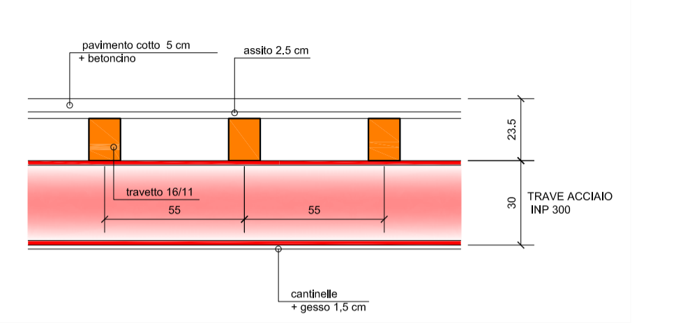
SONDAGGIO 33 Sezione soletta 1:20
