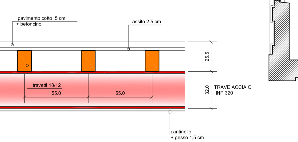
SONDAGGIO 6 Sezione soletta 1:20
