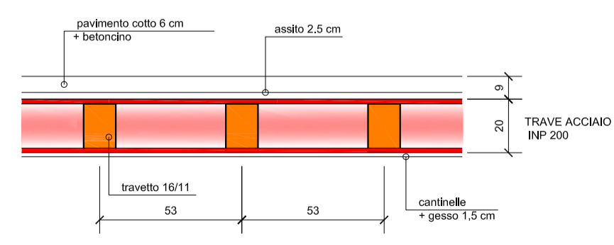
SONDAGGIO 41 Sezione soletta 1:20
