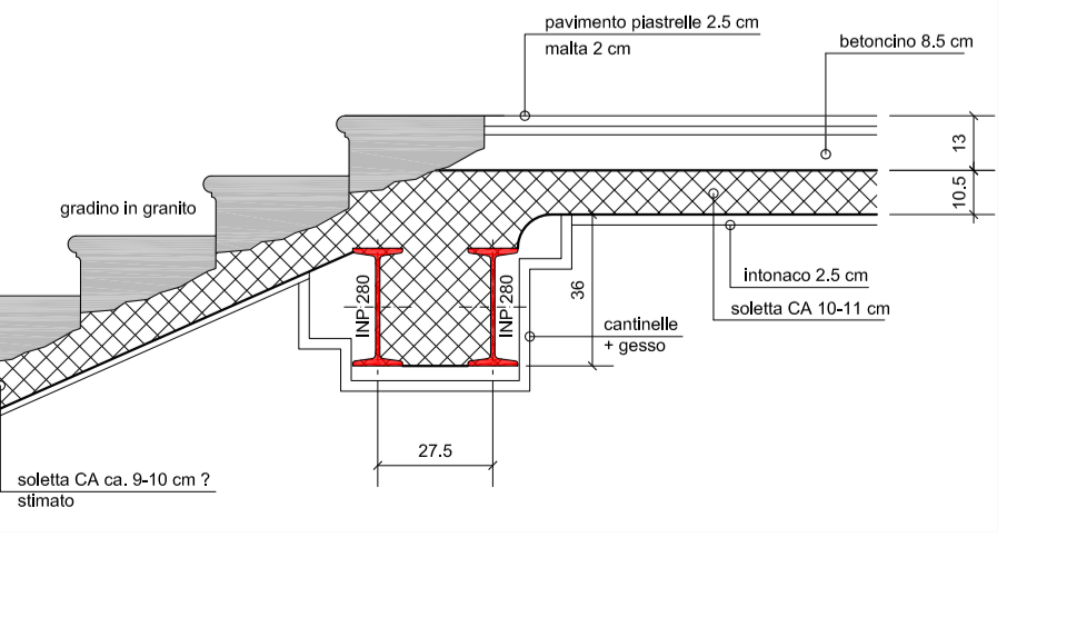
SONDAGGIO 5 Sezione trave 1:20
