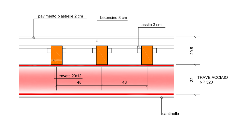
SONDAGGIO 2 Sezione soletta 1:20
