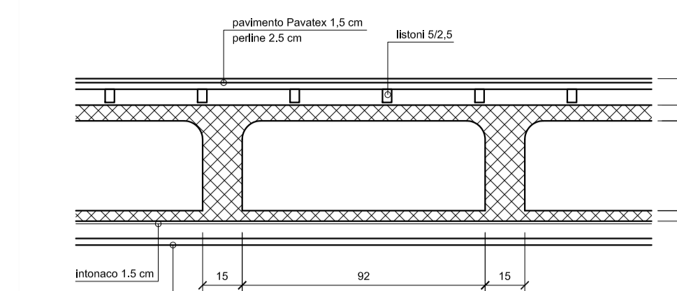
SONDAGGI 7 / 15 + 14 Sezione trave/soletta 1:20
