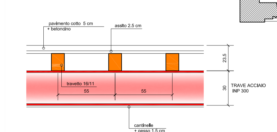
SONDAGGIO 31 Sezione soletta 1:20
