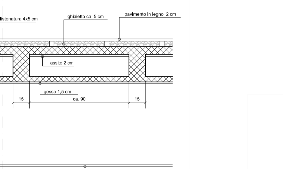
SONDAGGIO 2a Sezione soletta 1:20
