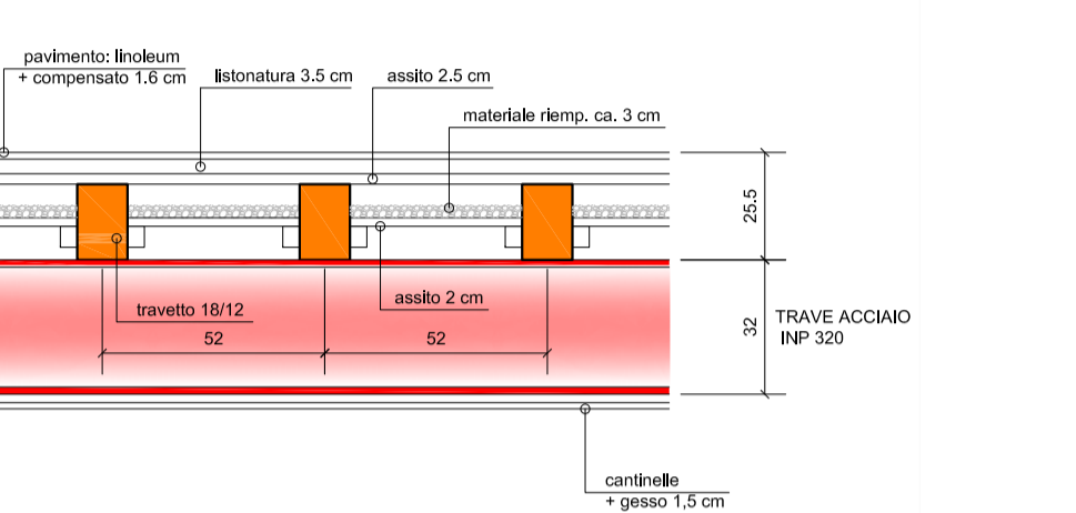
SONDAGGIO 1 Sezione soletta 1:20
