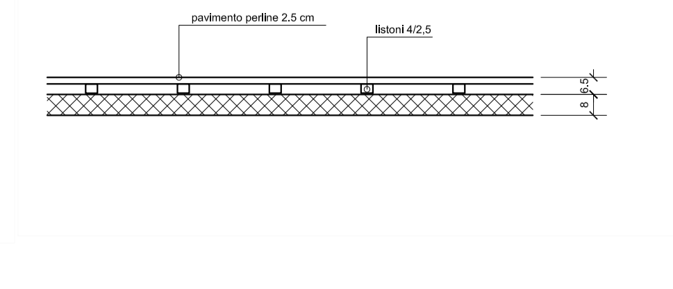
SONDAGGIO 8 Sezione soletta 1:20
