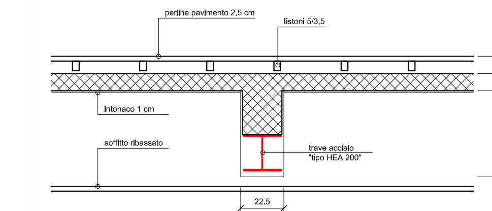
SONDAGGIO 2 / 1 Sezione trave/soletta 1:20
