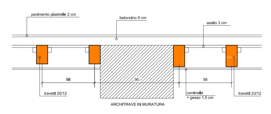
SONDAGGIO 3 Sezione soletta 1:20
