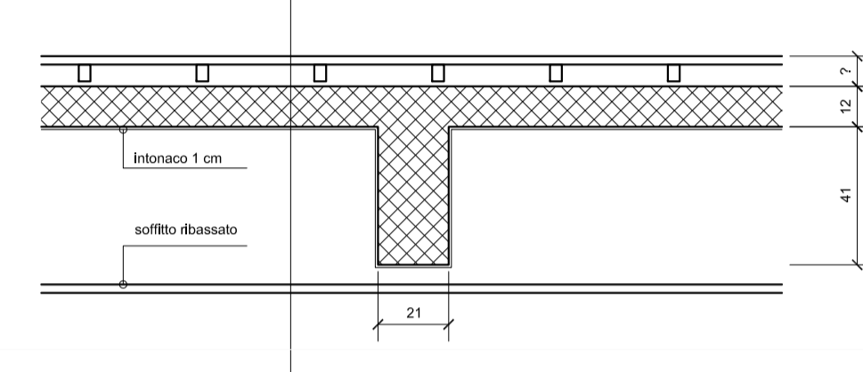
SONDAGGIO 2 Sezione trave/soletta 1:20
