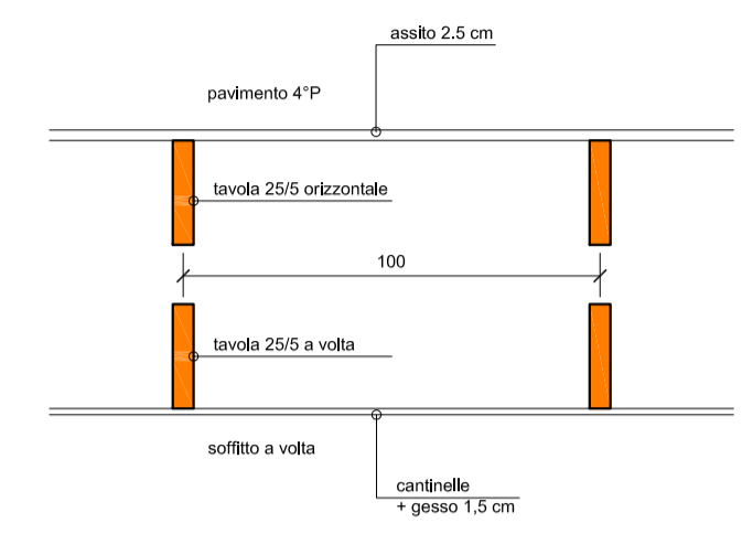
SONDAGGIO 1 Sezione soletta 1:20
