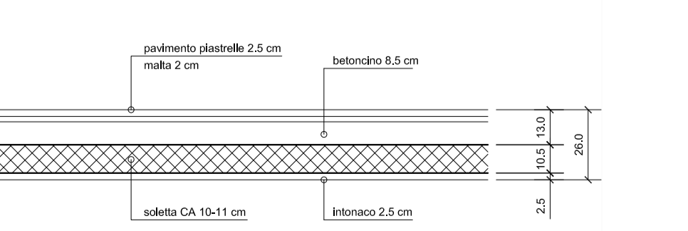
SONDAGGIO 7 Sezione soletta 1:20
