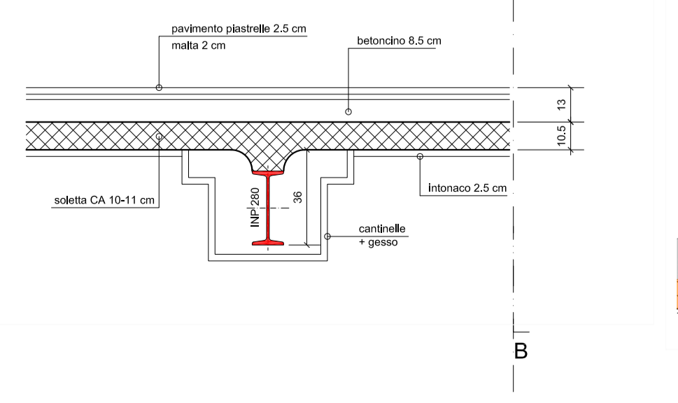
SONDAGGIO 4 Sezione trave/soletta 1:20
