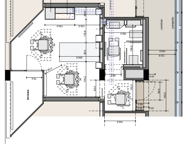
pianta camera tipo 1:50
