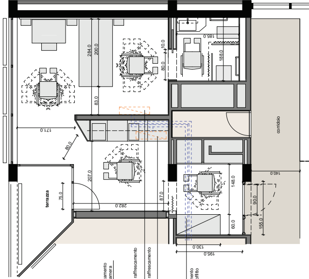
pianta camera ad angolo 1:50
