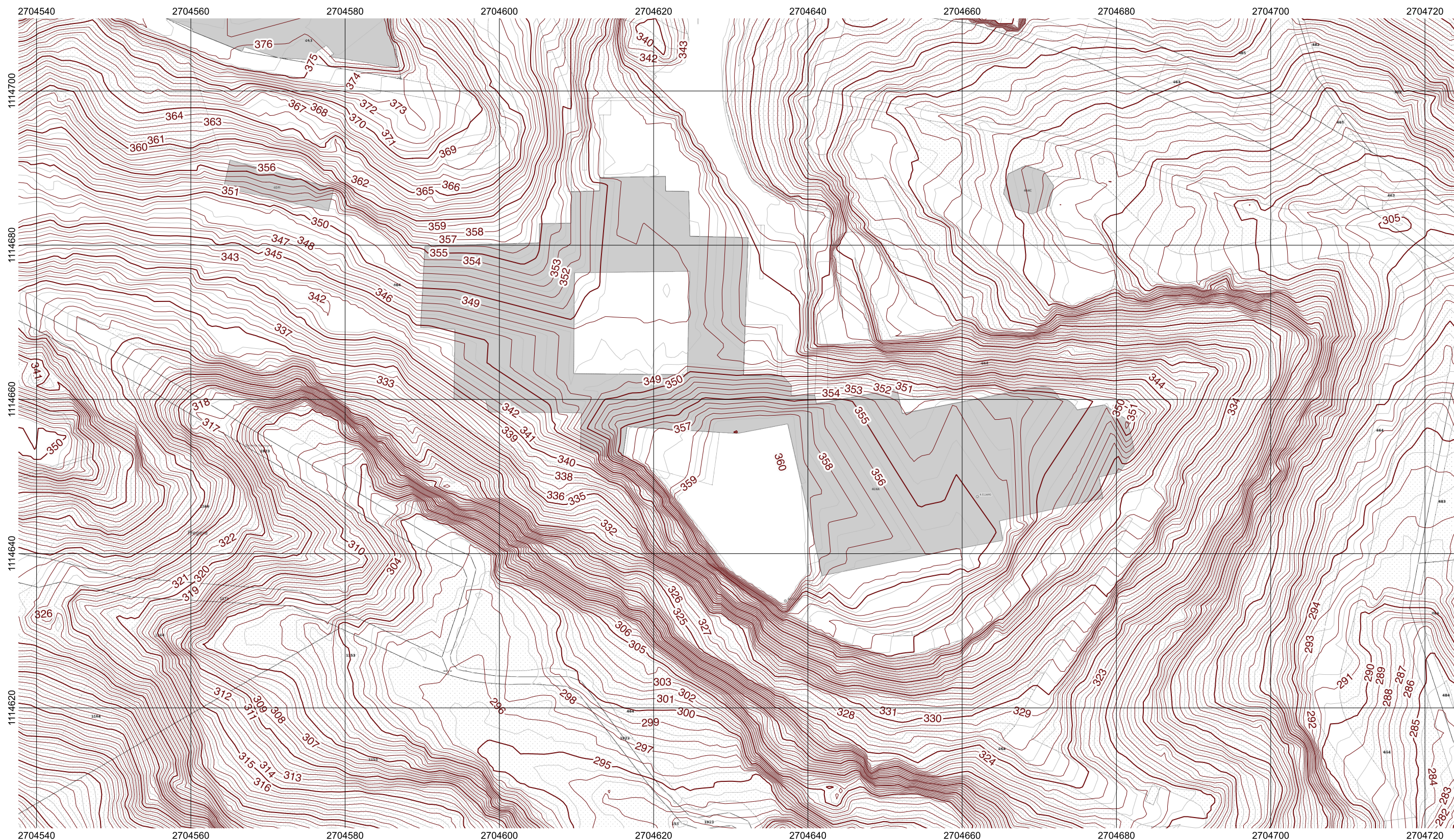
Planimetria 1:500
