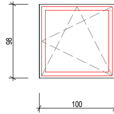
PT 07 - N° 2 pz Finestra con apertura ad anta e ribalta. Vetro camera triplo.
