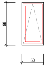
PT 06 - N° 3 pz Finestra con apertura ad anta e ribalta. Vetro camera triplo. Pellicola satinata.
