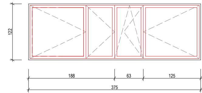
PT 12 - N° 1 pz Finestra con apertura ad anta e ribalta. Vetro camera triplo con lastra interna stratificata di sicurezza.
