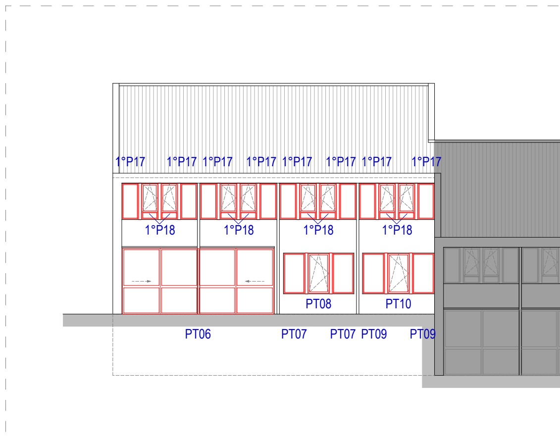
FACCIATA SUD-EST
