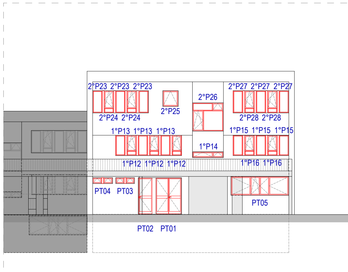
FACCIATA NORD-OVEST
