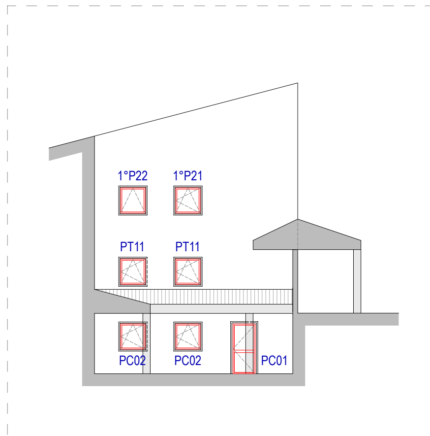
FACCIATA NORD-EST
