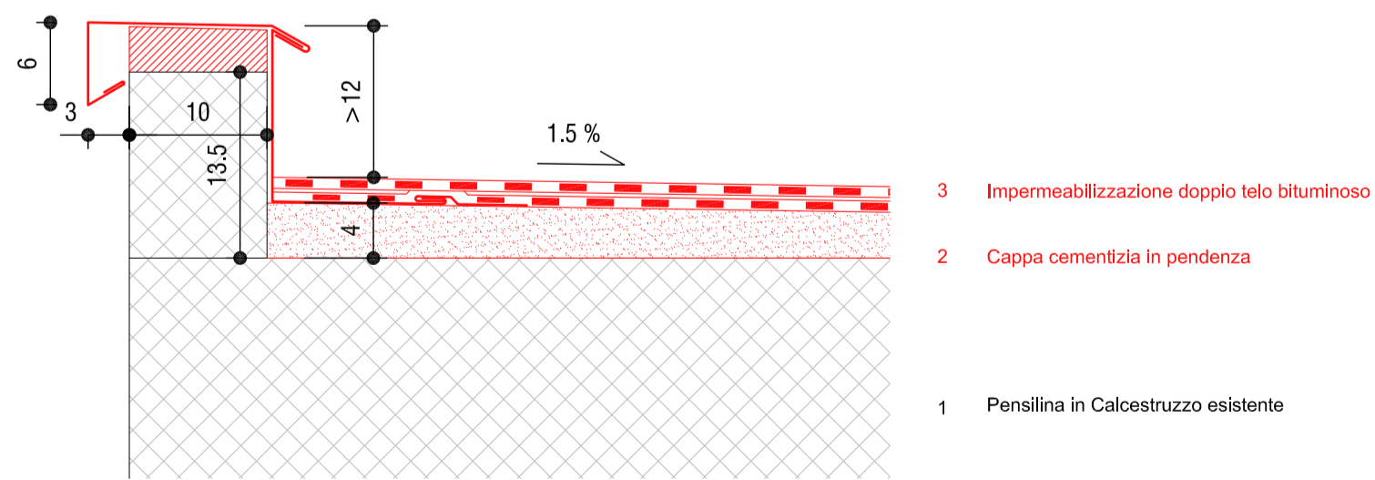
Intervento: Dettaglio tipo - pensiline 1.5
