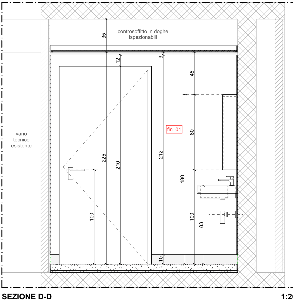
SEZIONE D-D 1:20
