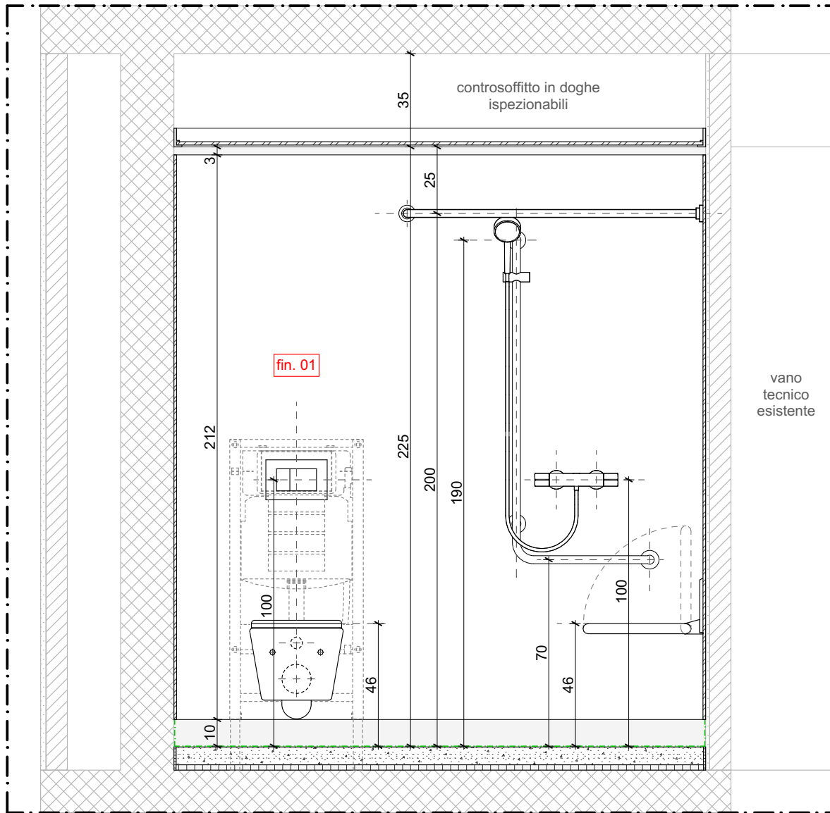
SEZIONE B-B 1:20
