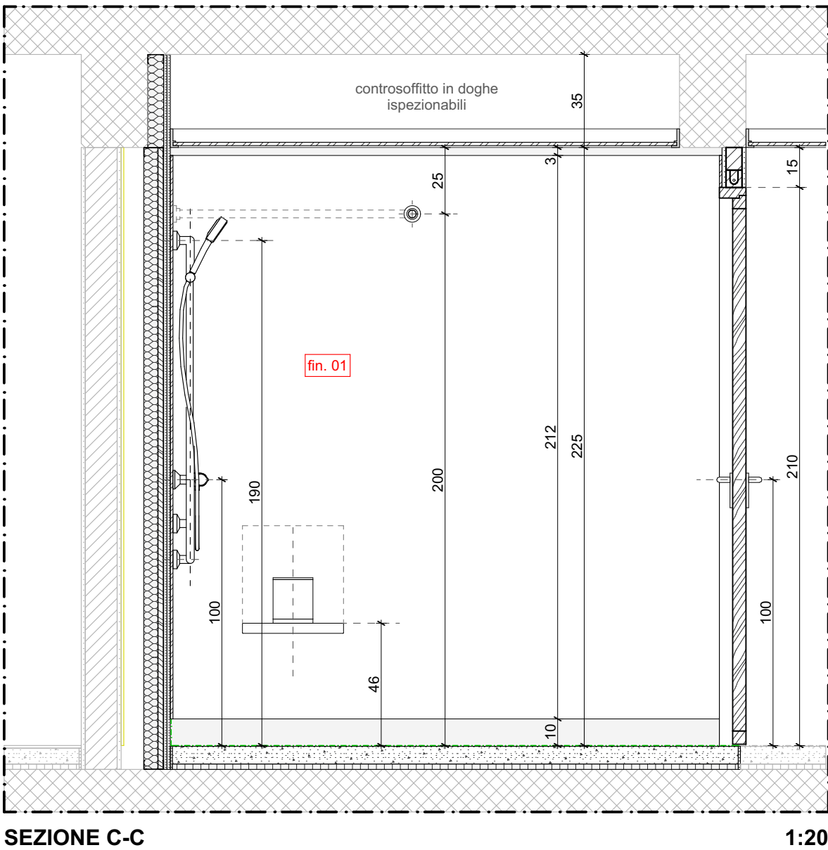
SEZIONE C-C 1:20
