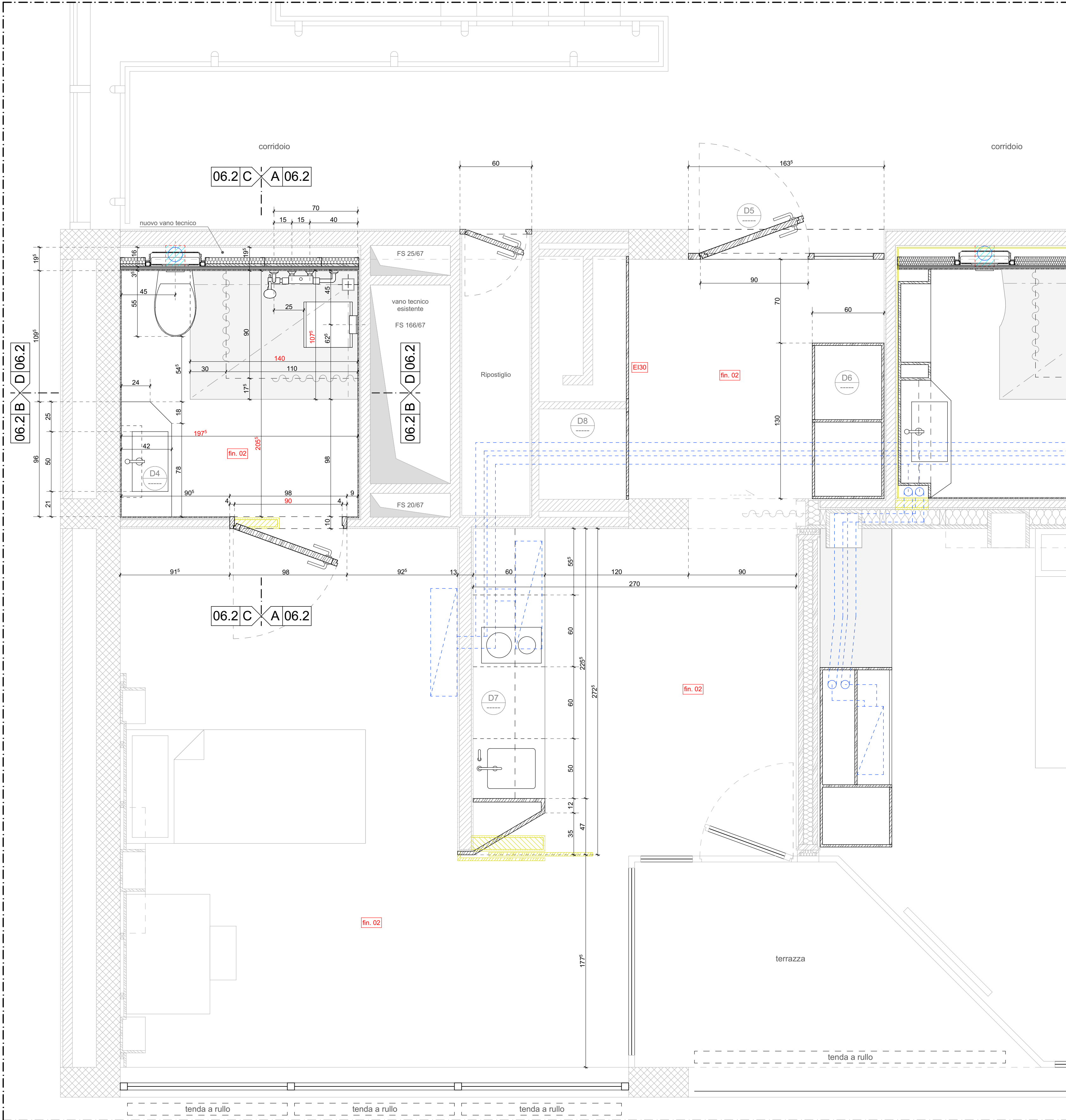
PIANTA CAMERA ANGOLO E BAGNO - STANDARD
