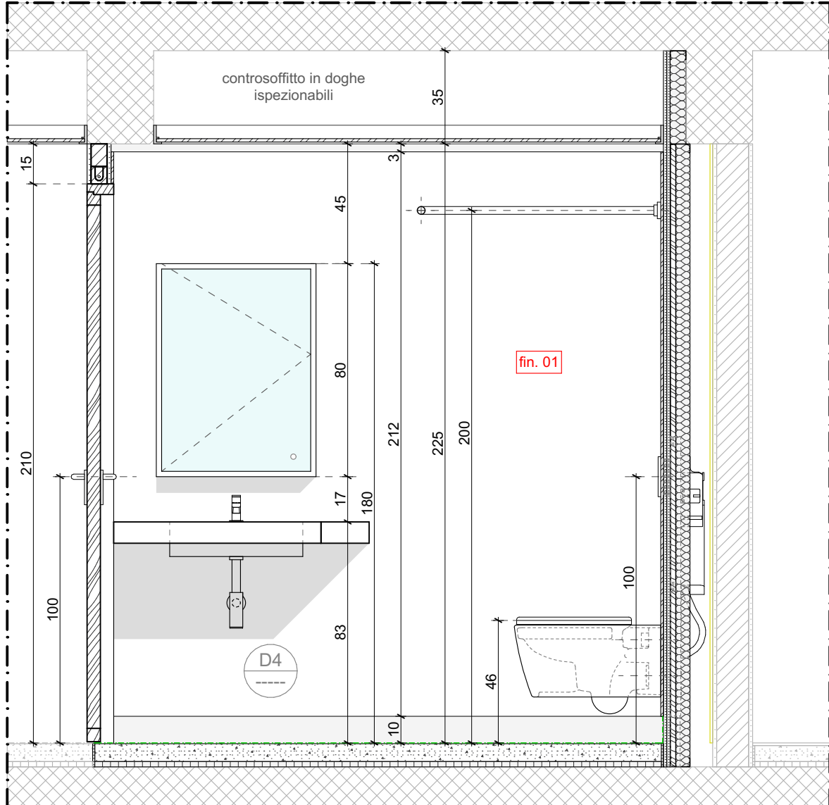
SEZIONE A-A 1:20
