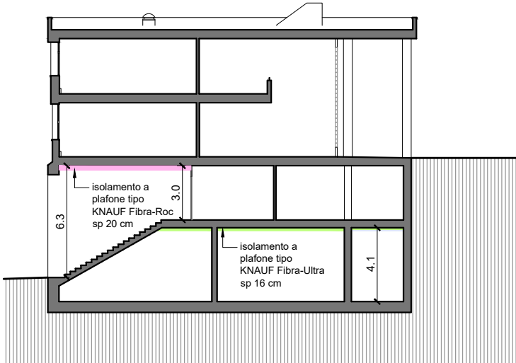
SEZIONE A-A
