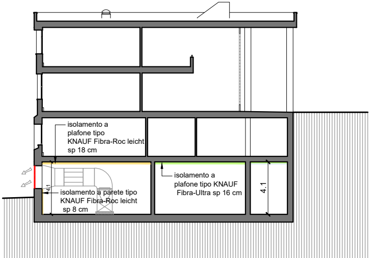
SEZIONE B-B
