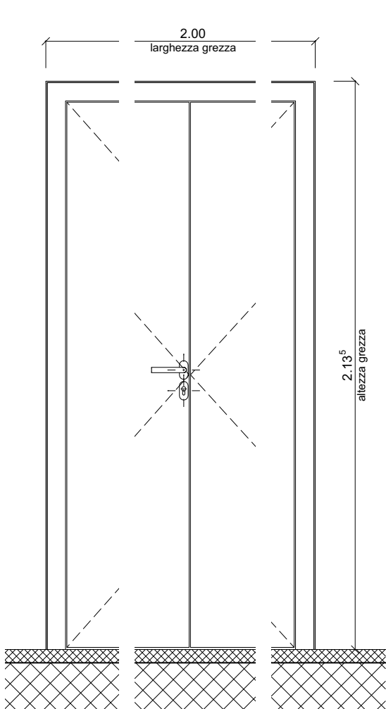
PROSPETTO INTERNO 1:20
