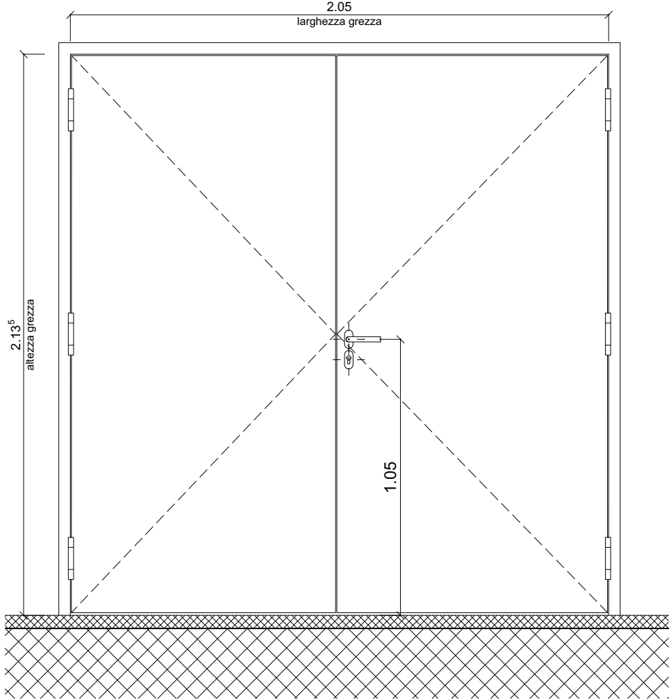
PROSPETTO ESTERNO 1:20
