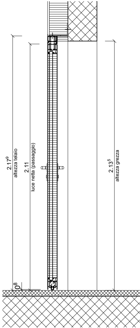
PROSPETTO INTERNO 1:20
