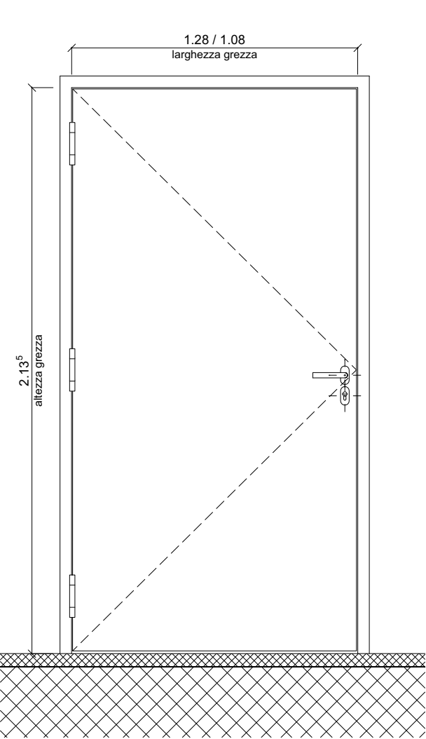
PROSPETTO ESTERNO 1:20
