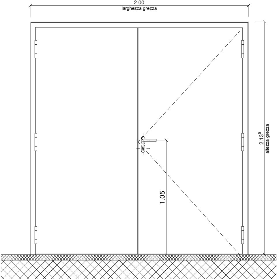
PROSPETTO ESTERNO 1:20
