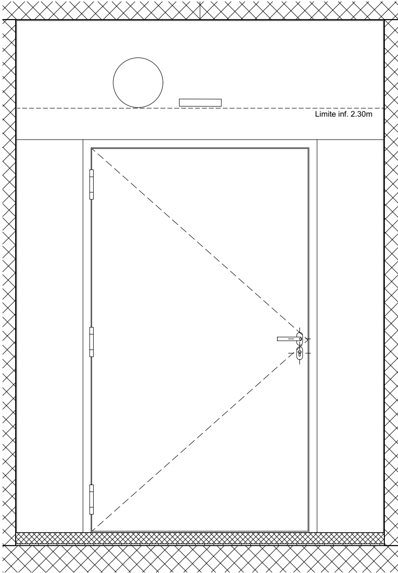
PROSPETTO INTERNO 1:20
