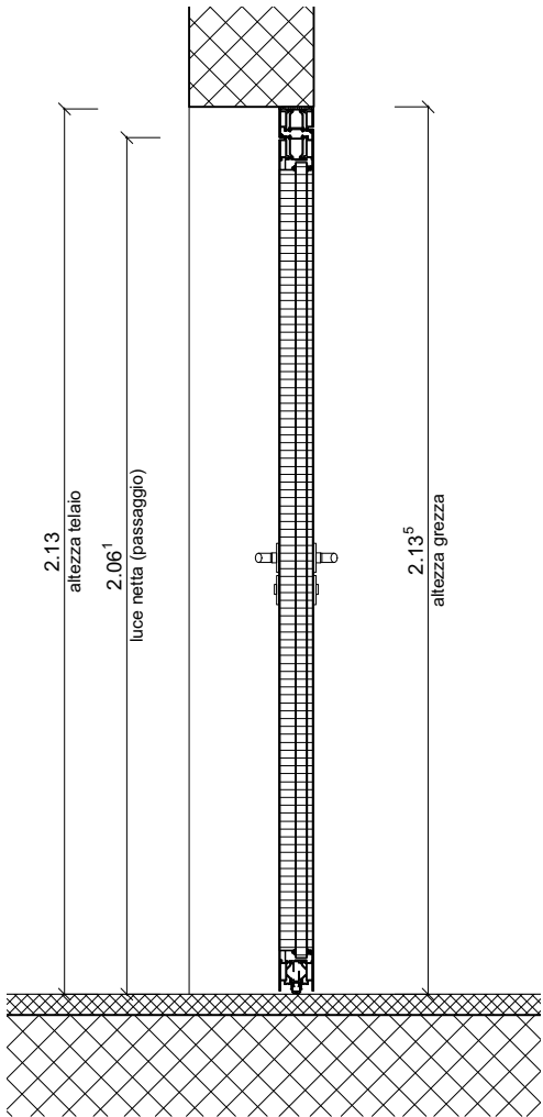
SEZIONE 1:20
