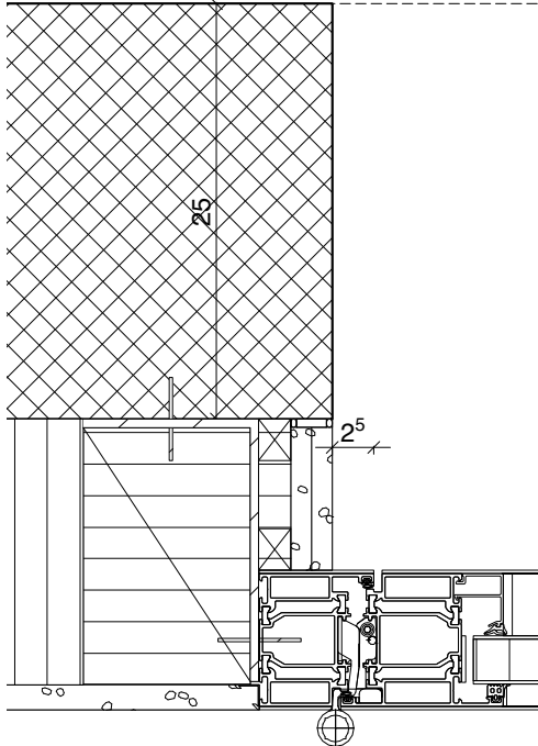
PIANTA DETTAGLIO 1:5
