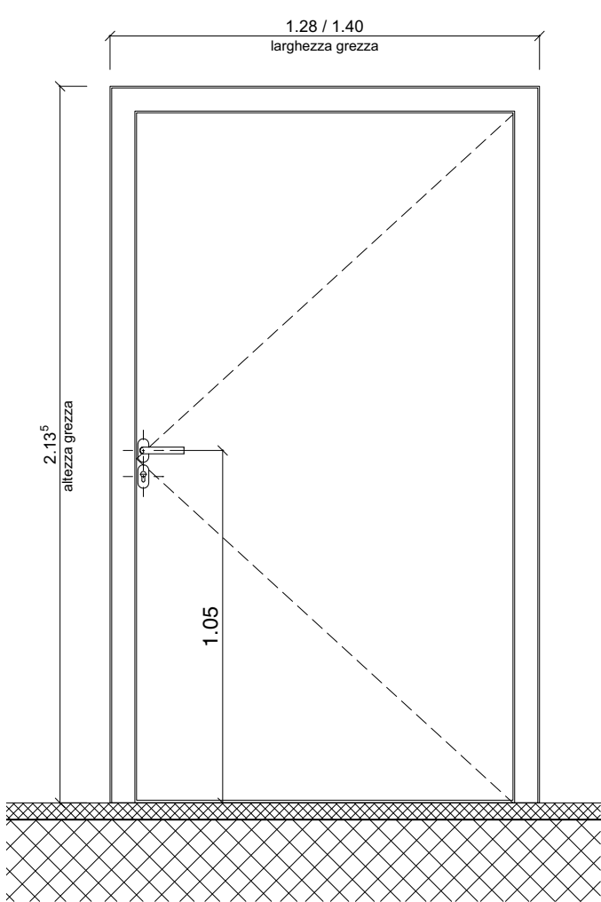
PROSPETTO INTERNO 1:20
