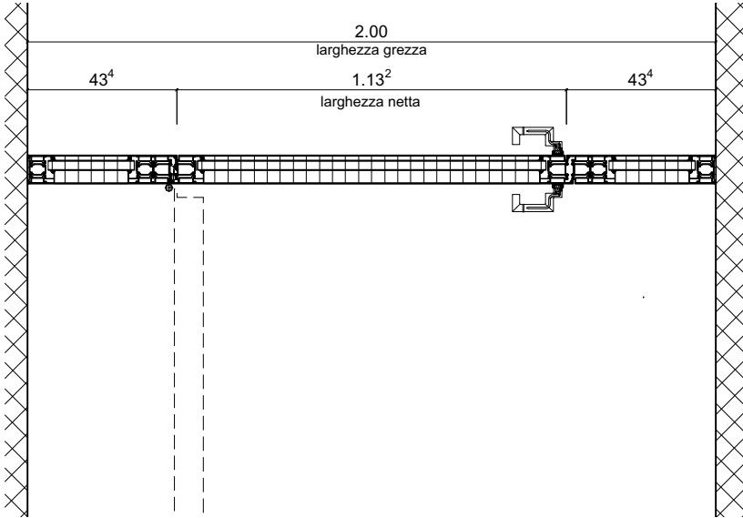
PIANTA 1:20
