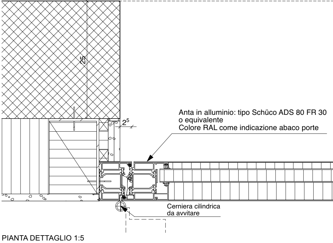
PIANTA DETTAGLIO 1:5
