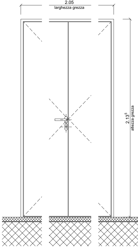
PROSPETTO INTERNO 1:20
