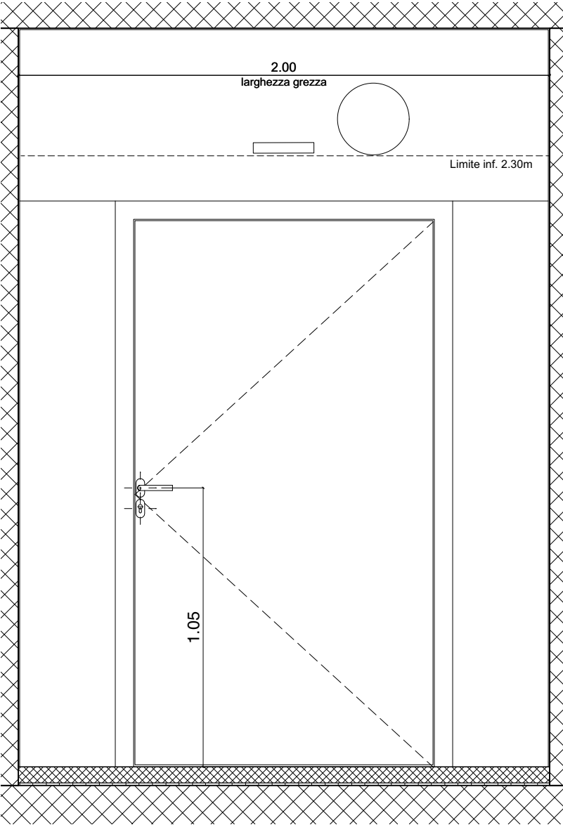
PROSPETTO ESTERNO 1:20
