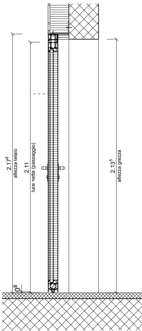
SEZIONE 1:20
