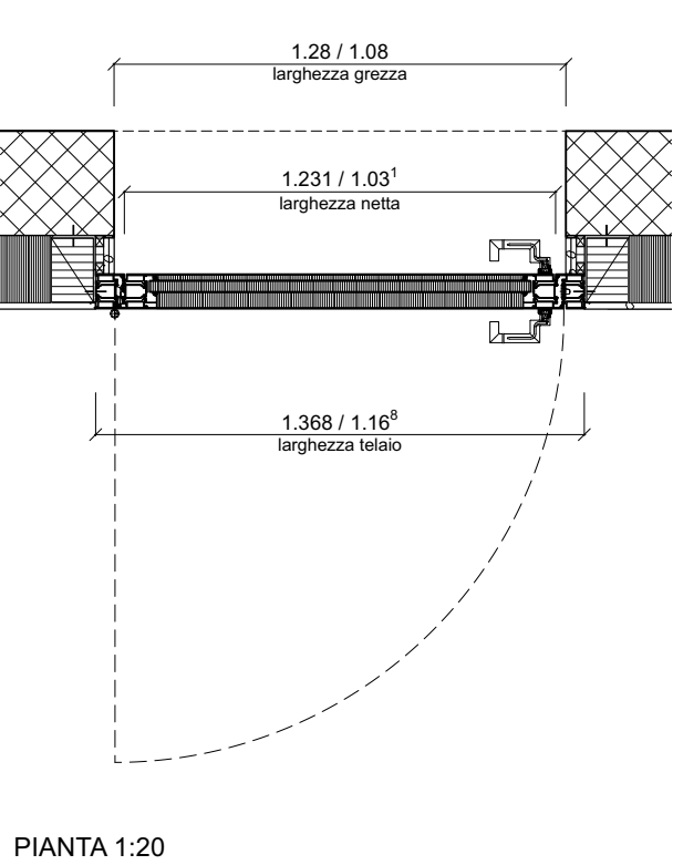
PIANTA 1:20
