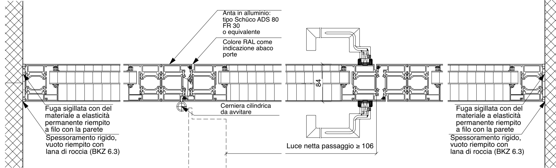
PIANTA DETTAGLIO 1:5
