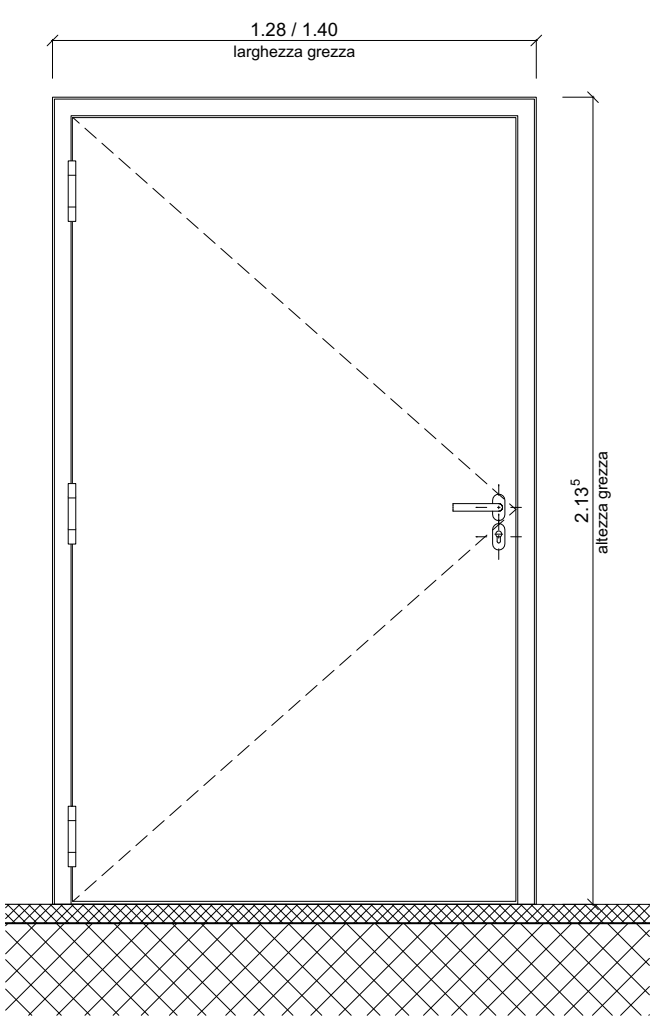
PROSPETTO ESTERNO 1:20
