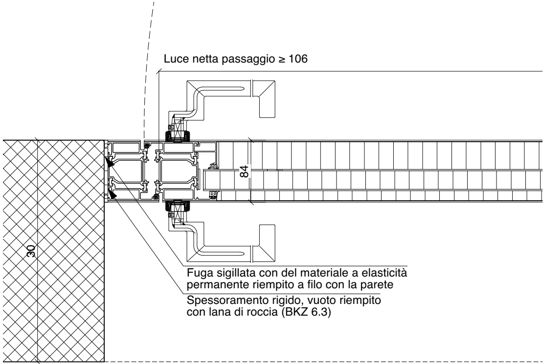
PIANTA DETTAGLIO 1:5
