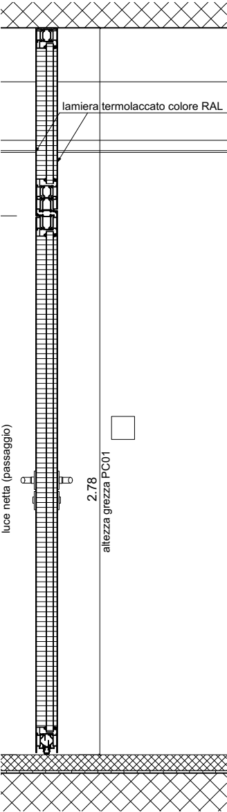
SEZIONE 1:20
