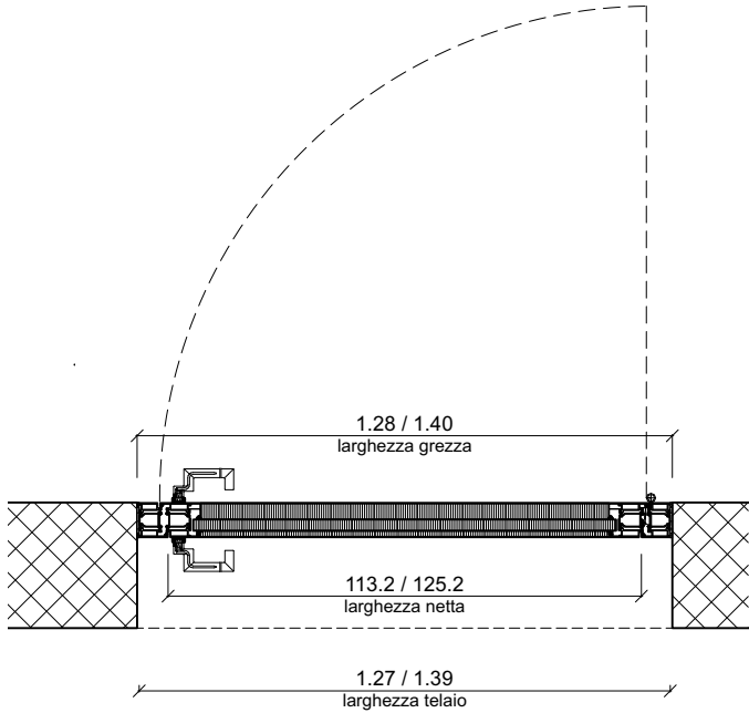
PIANTA 1:20
