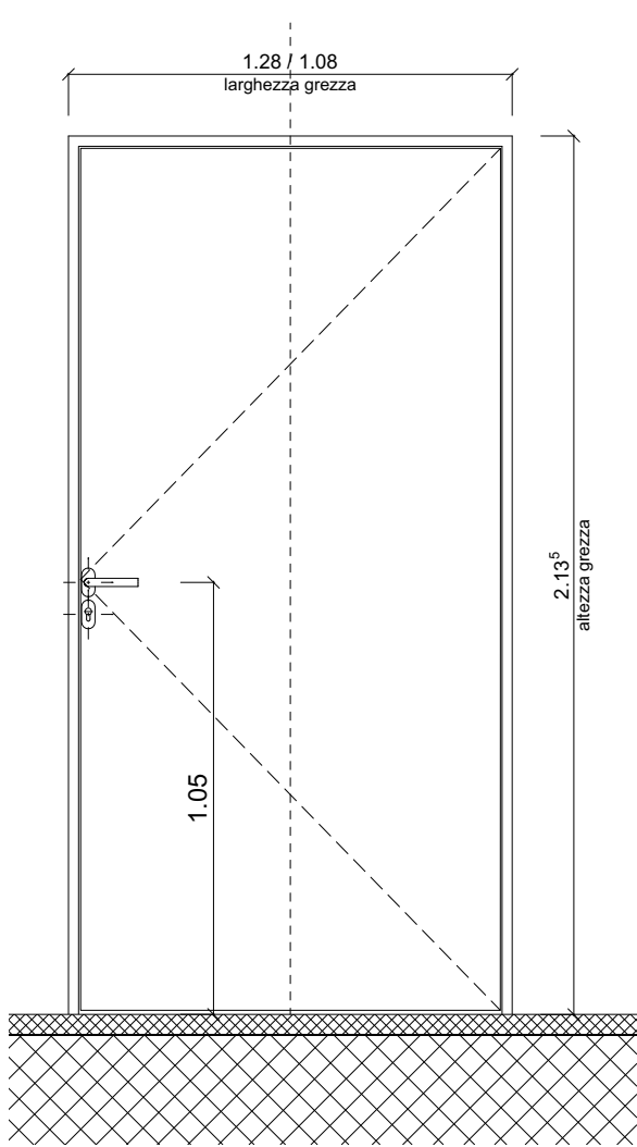
PROSPETTO INTERNO 1:20
