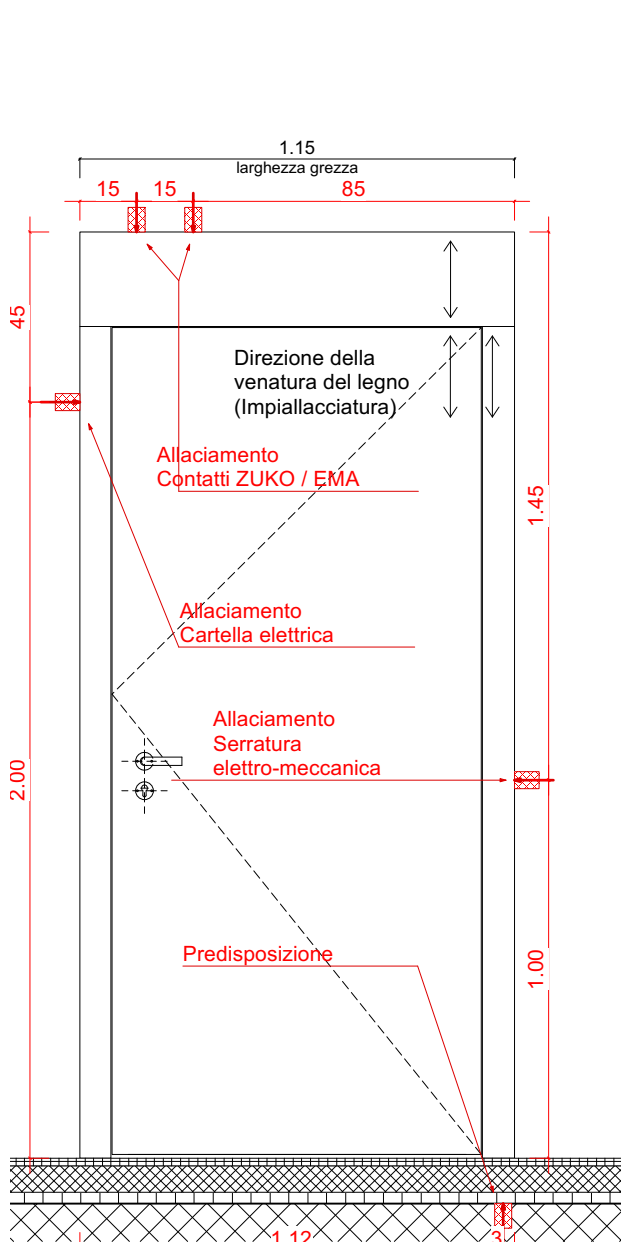
PROSPETTO INTERNO 1:20
