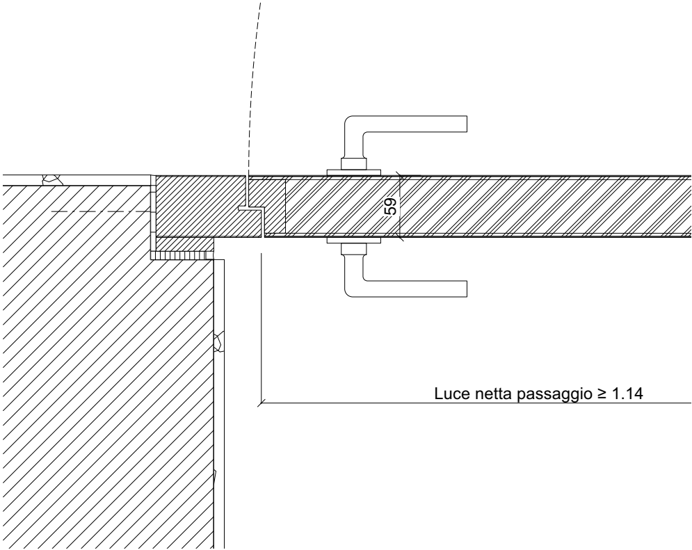
PIANTA DETTAGLIO 1:5
