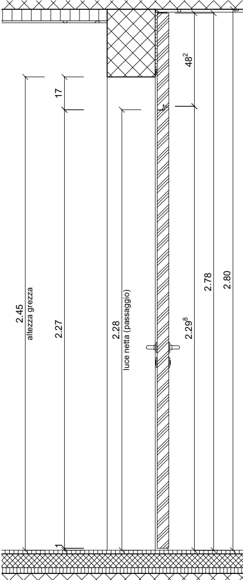
SEZIONE 1:20
