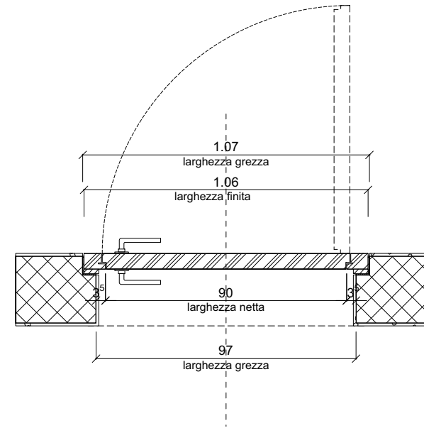
PIANTA 1:20
