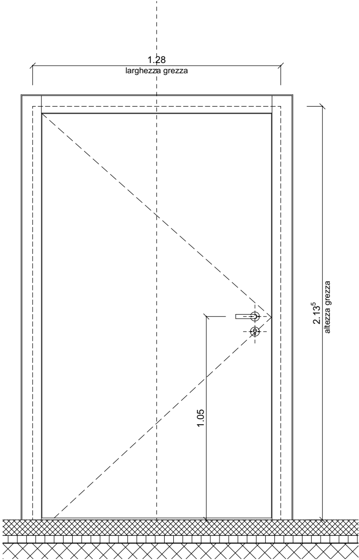
PROSPETTO INTERNO 1:20
