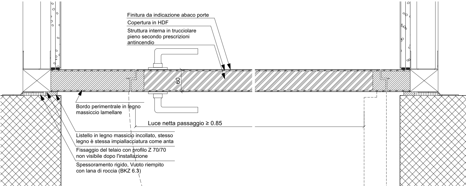
SEZIONE 1:20
