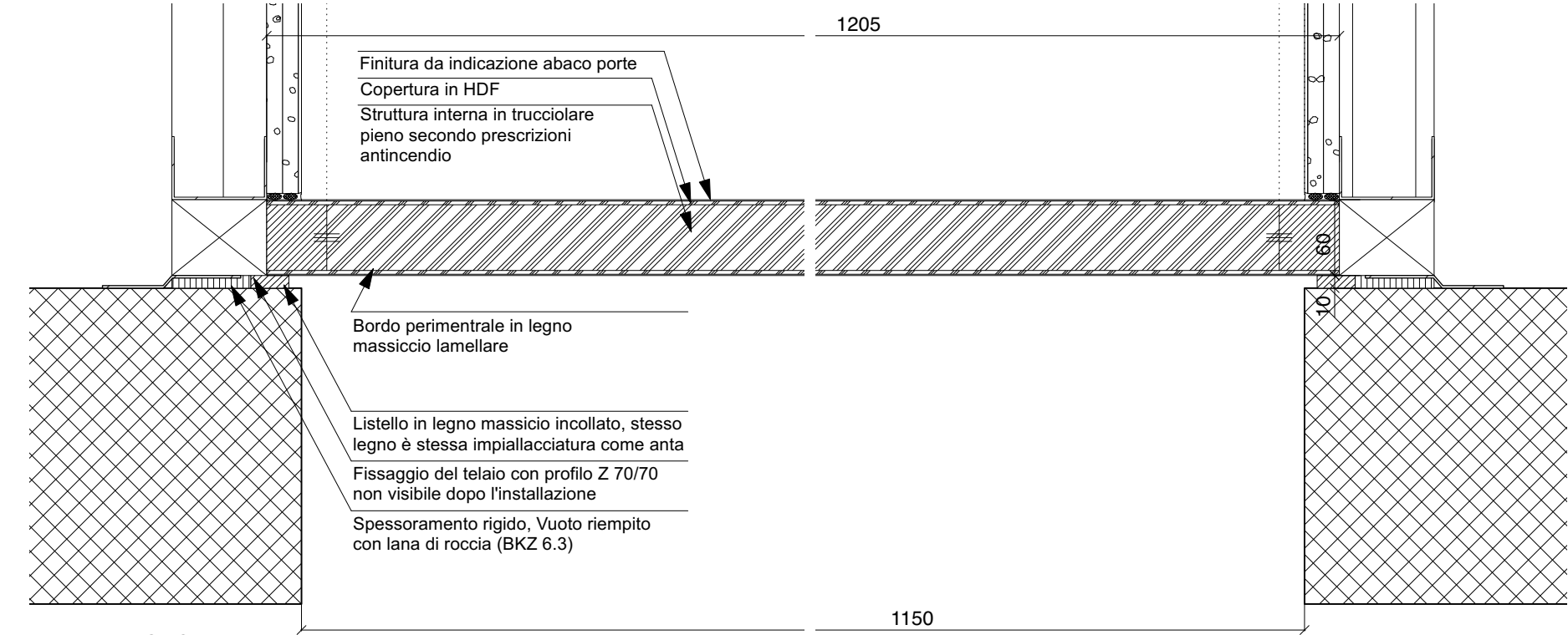
PIANTA DETTAGLIO 1:5
