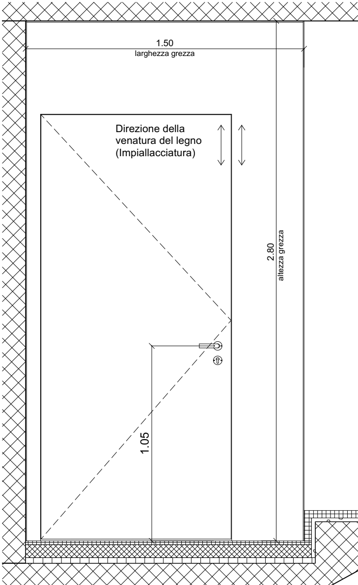
PROSPETTO ESTERNO 1:20
