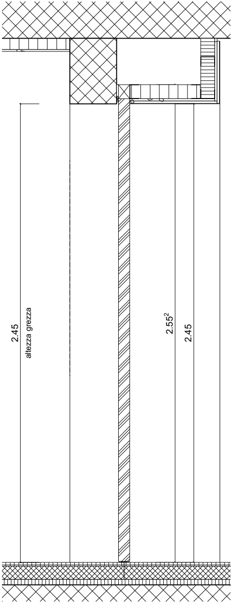
SEZIONE 1:20
