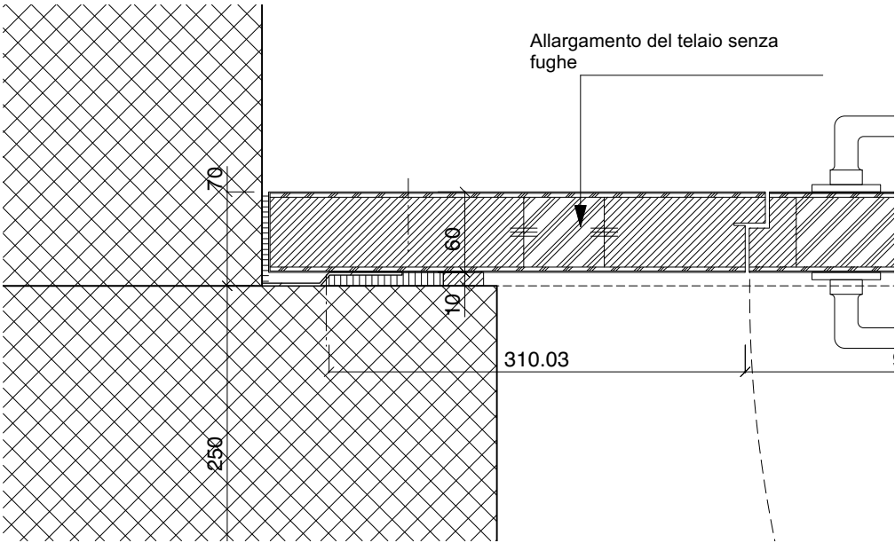
PIANTA DETTAGLIO 1:5
