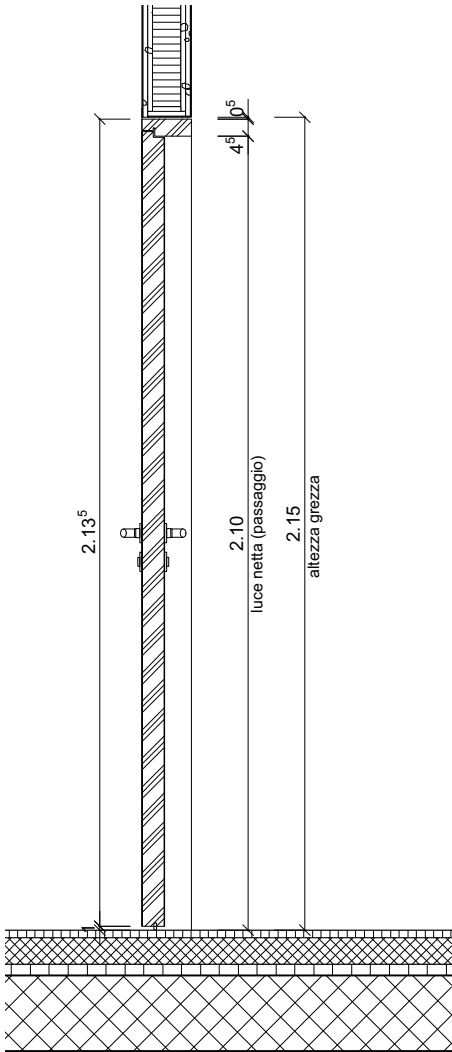
SEZIONE 1:20
