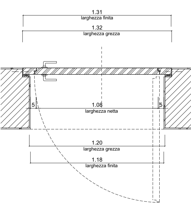
PIANTA 1:20
