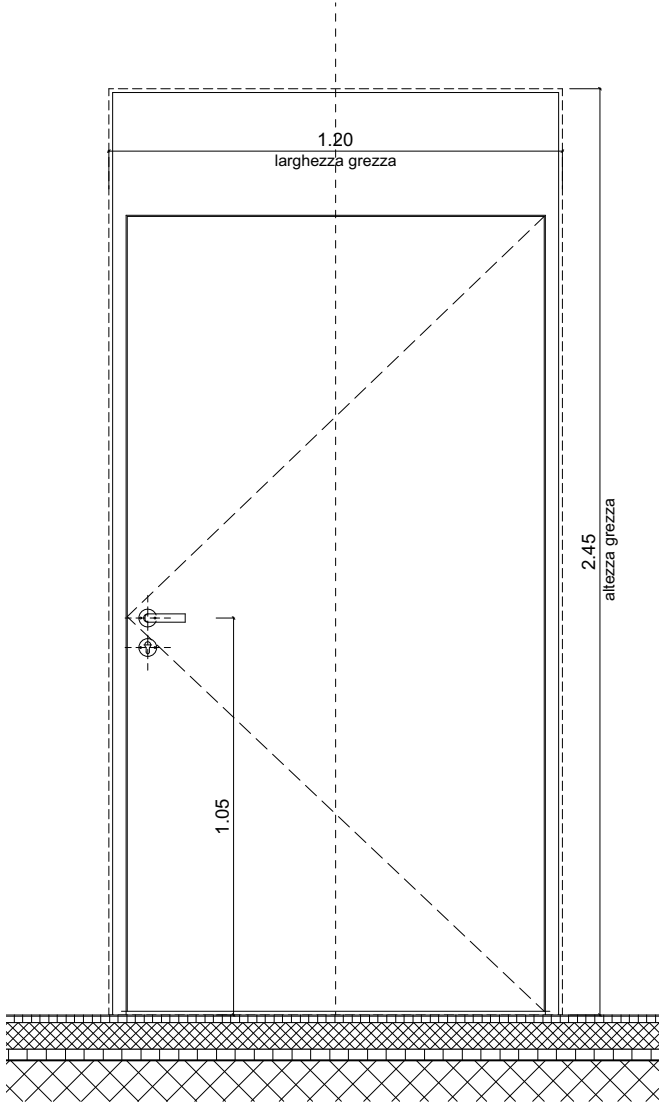
PROSPETTO ESTERNO 1:20
