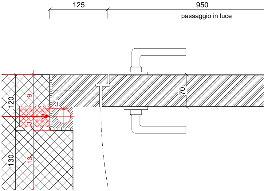
PIANTA DETTAGLIO 1:5
