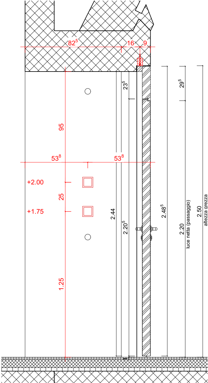
SEZIONE 1:20
