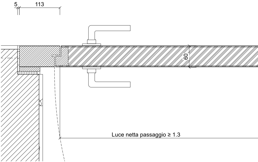
PIANTA DETTAGLIO 1:5
