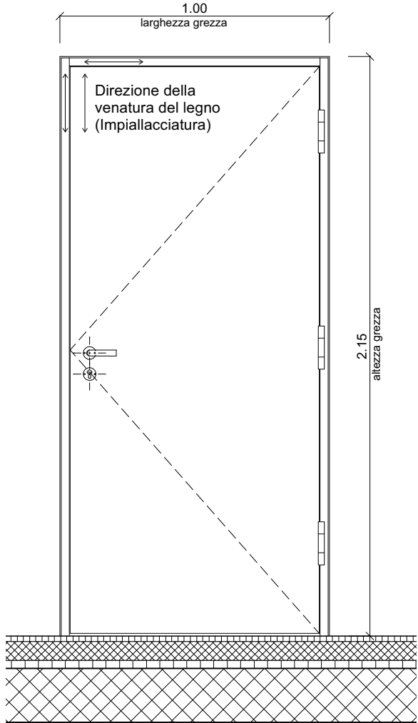
PROSPETTO ESTERNO 1:20
