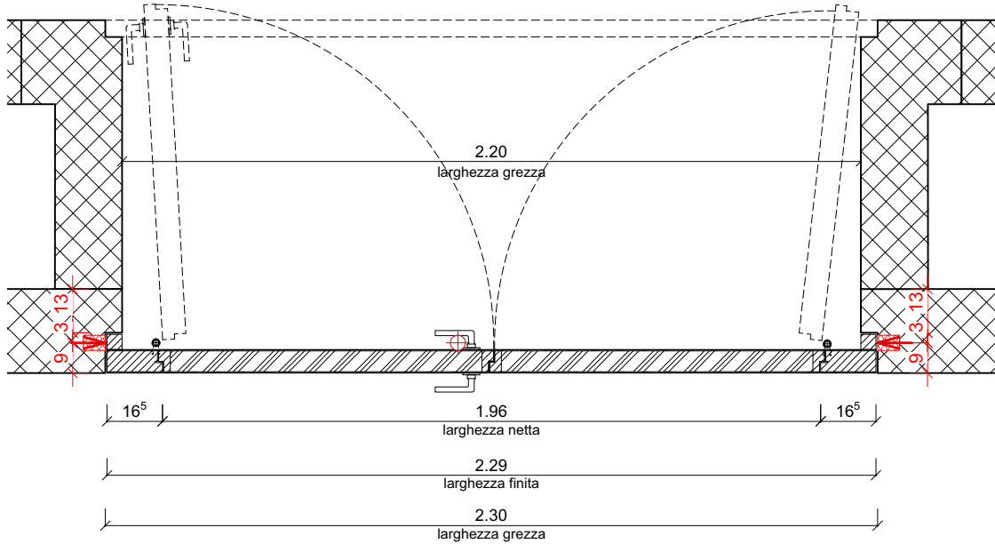
PIANTA 1:20
