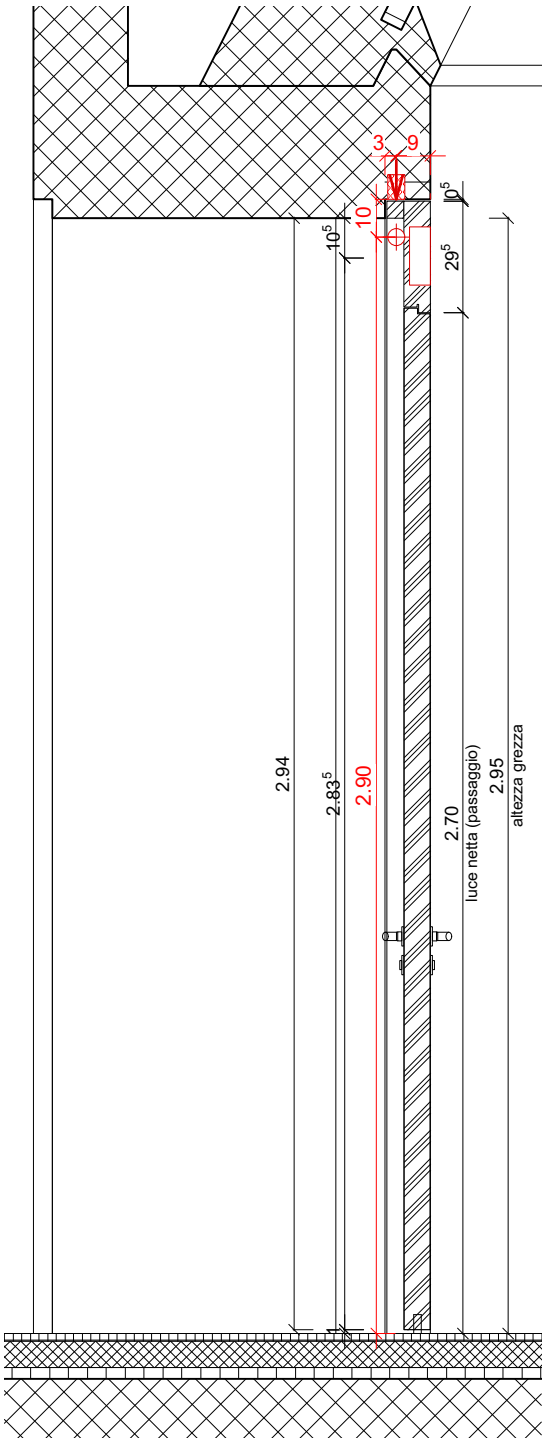
SEZIONE 1:20
