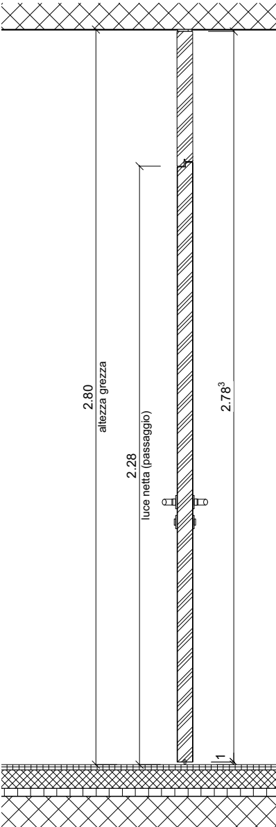
SEZIONE 1:20
