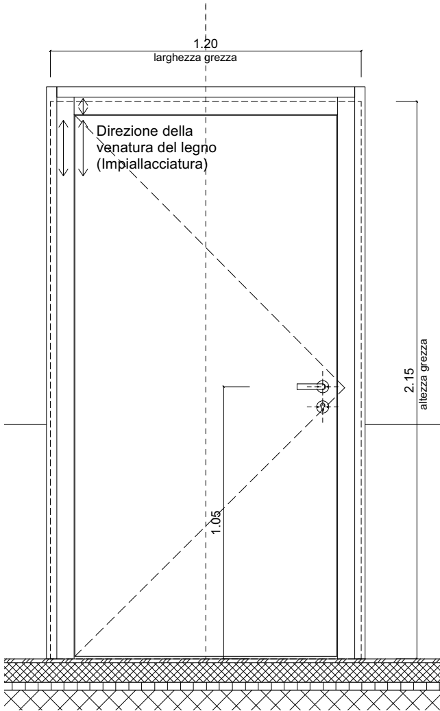
PROSPETTO INTERNO 1:20
