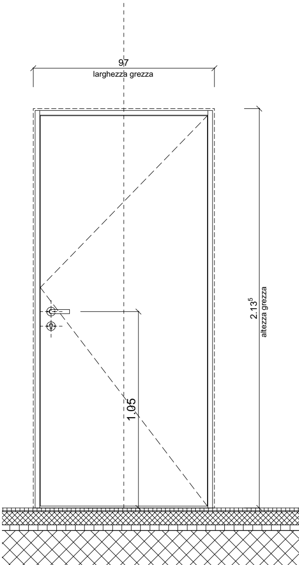
PROSPETTO INTERNO 1:20
