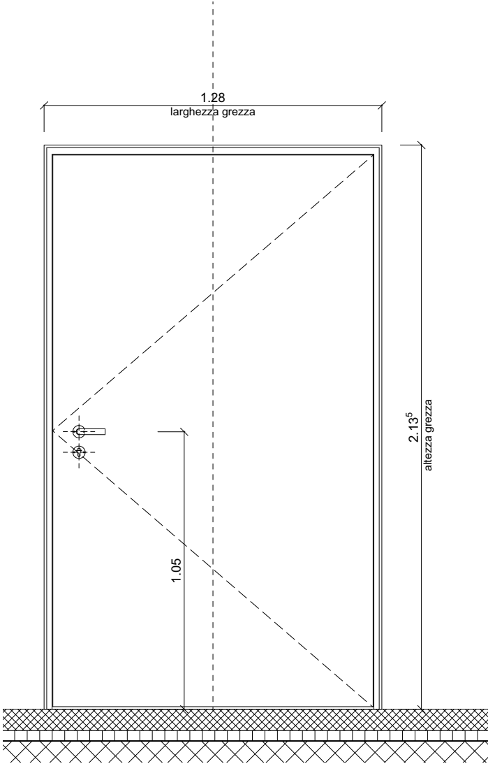
PROSPETTO ESTERNO 1:20
