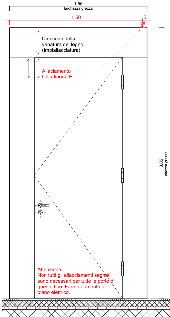
PROSPETTO INTERNO 1:20
