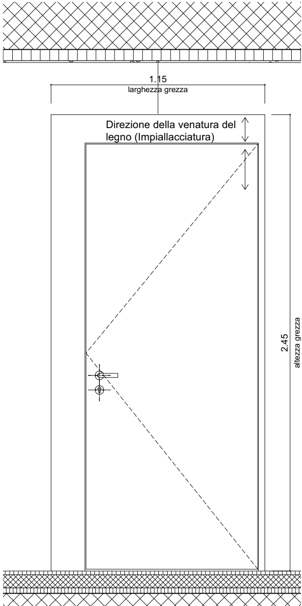
PROSPETTO INTERNO 1:20
