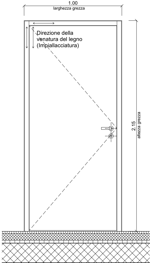
PROSPETTO INTERNO 1:20
