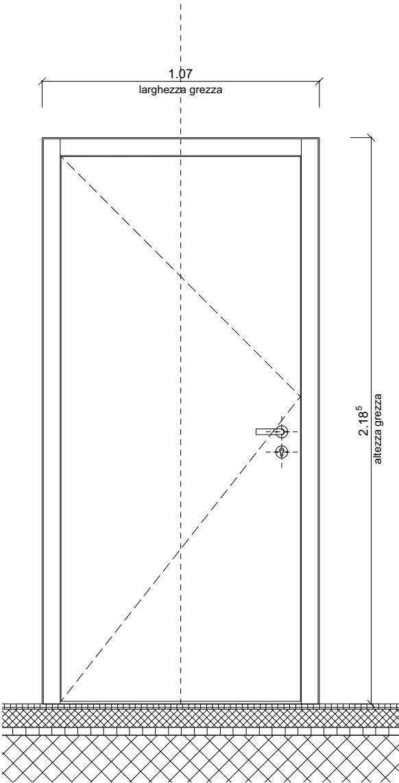
PROSPETTO ESTERNO 1:20
