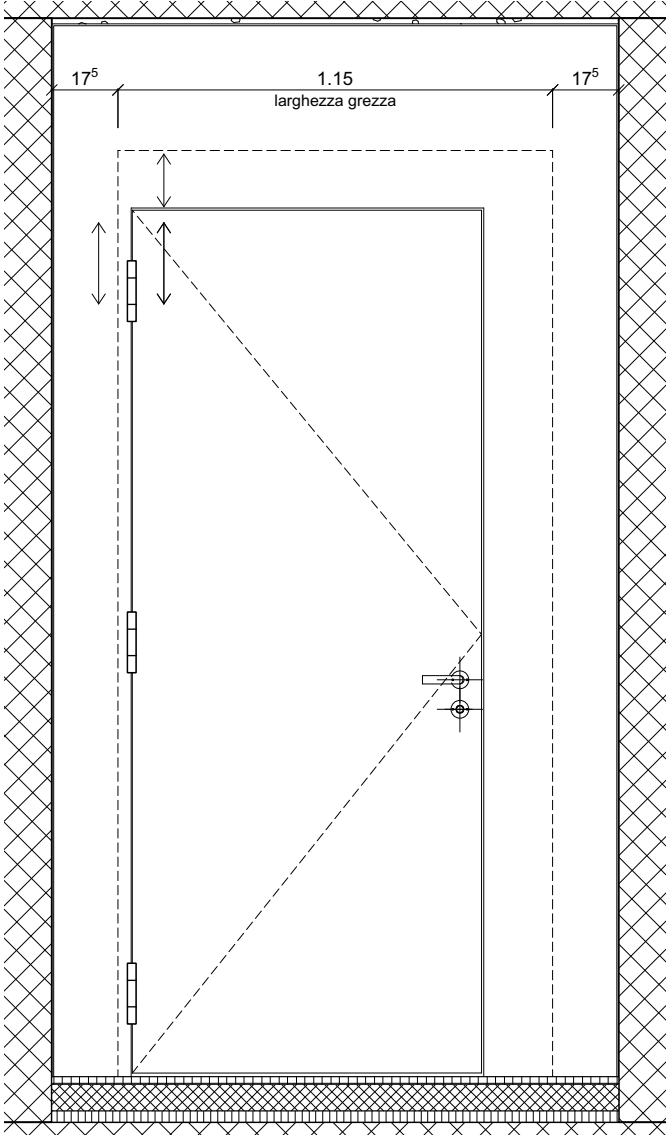
PROSPETTO ESTERNO 1:20
