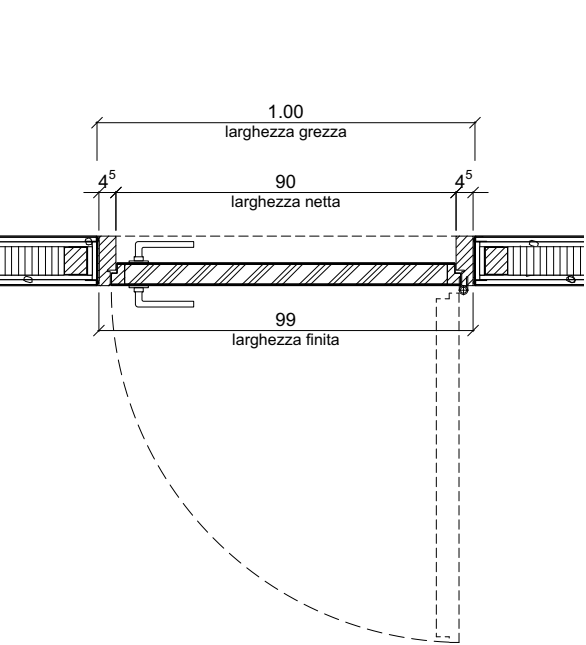
PIANTA 1:20
