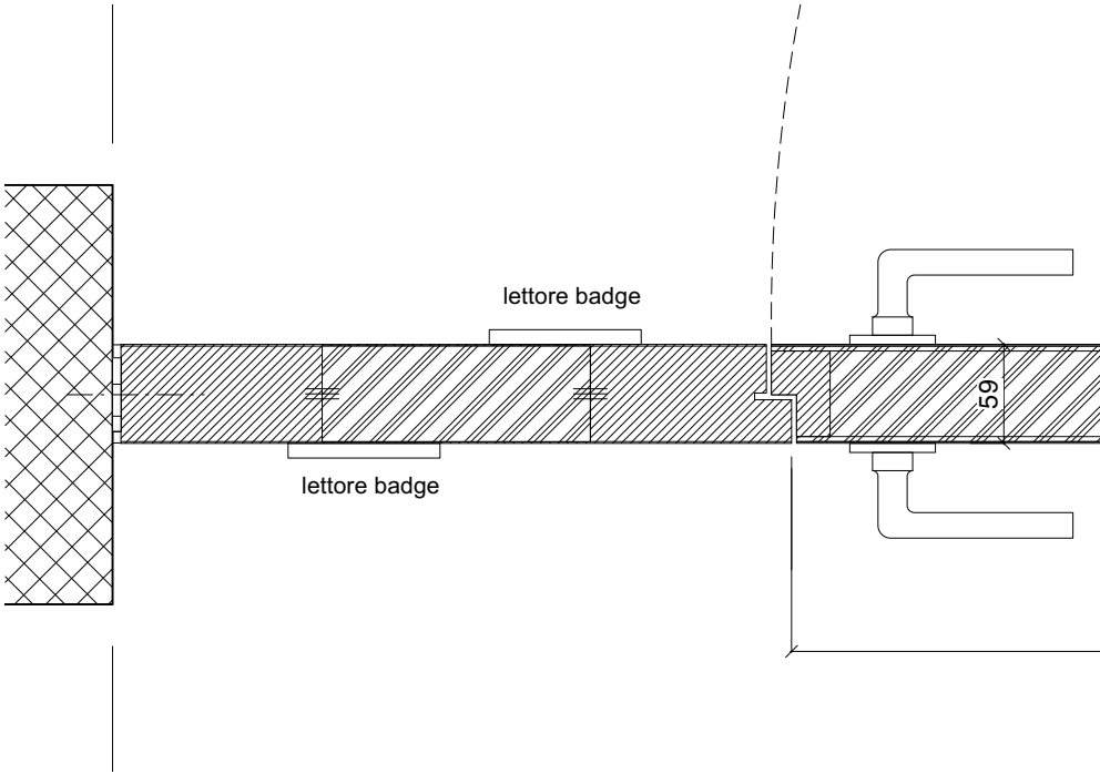
PIANTA DETTAGLIO 1:5
