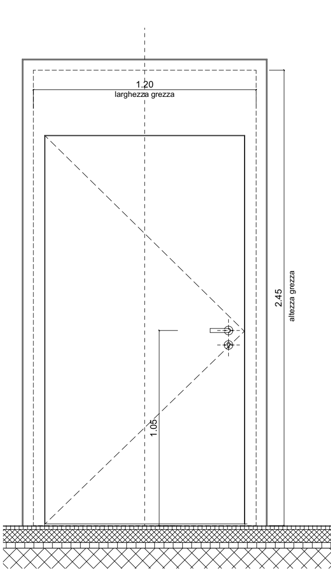
PROSPETTO INTERNO 1:20
