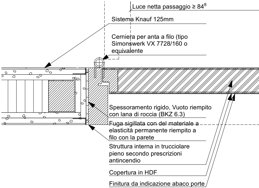
PIANTA DETTAGLIO 1:5
