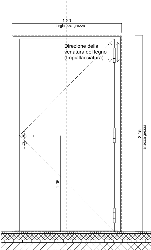
PROSPETTO ESTERNO 1:20
