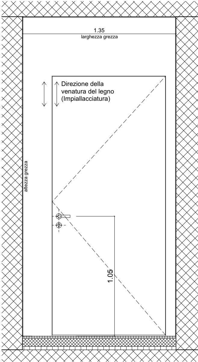
PROSPETTO INTERNO 1:20
