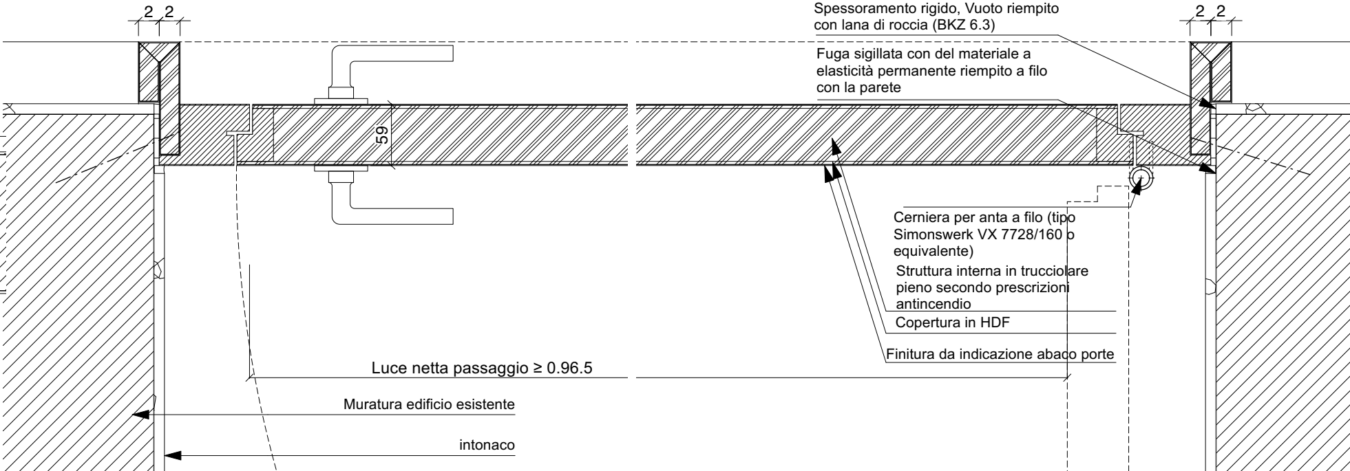
PIANTA DETTAGLIO 1:5
