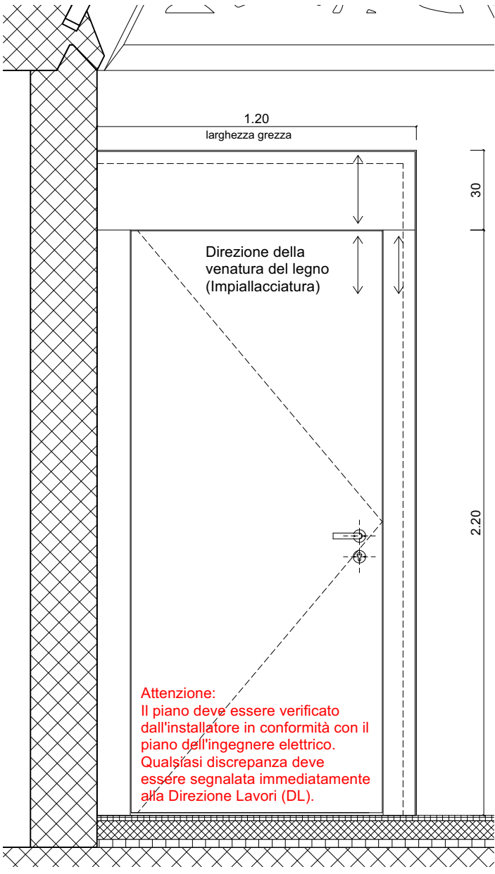
PROSPETTO ESTERNO 1:20
