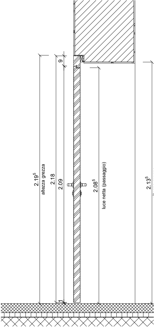
SEZIONE 1:20
