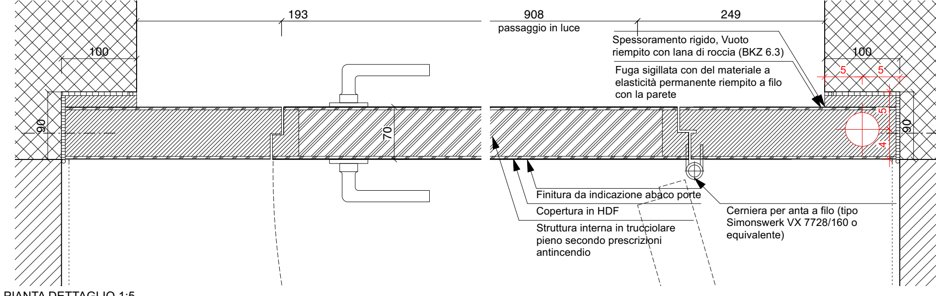
PIANTA DETTAGLIO 1:5
