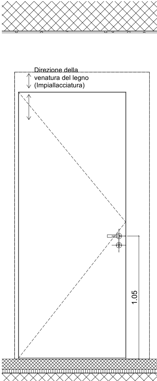
PROSPETTO ESTERNO 1:20
