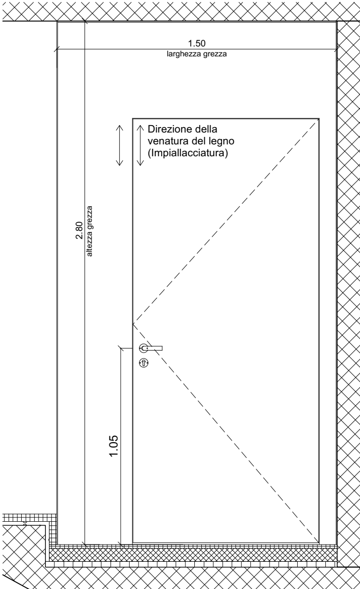
PROSPETTO INTERNO 1:20
