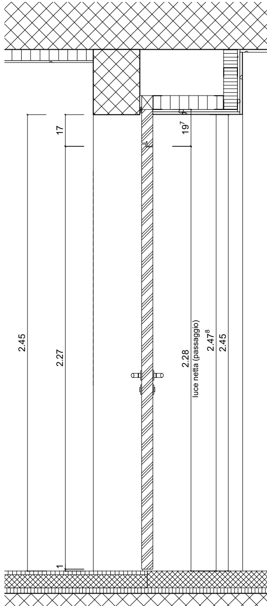
SEZIONE 1:20
