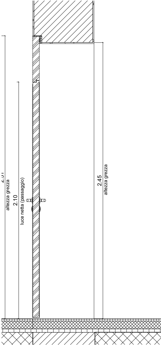
SEZIONE 1:20
