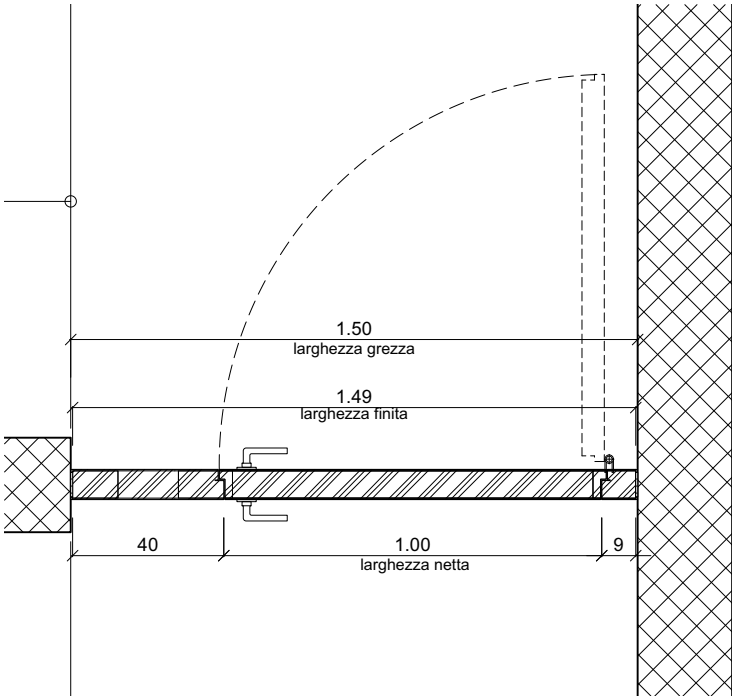
PIANTA 1:20
