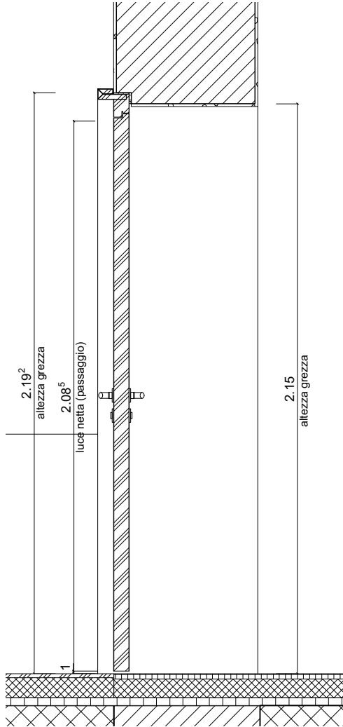
SEZIONE 1:20
