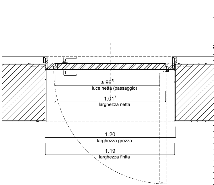
PIANTA 1:20
