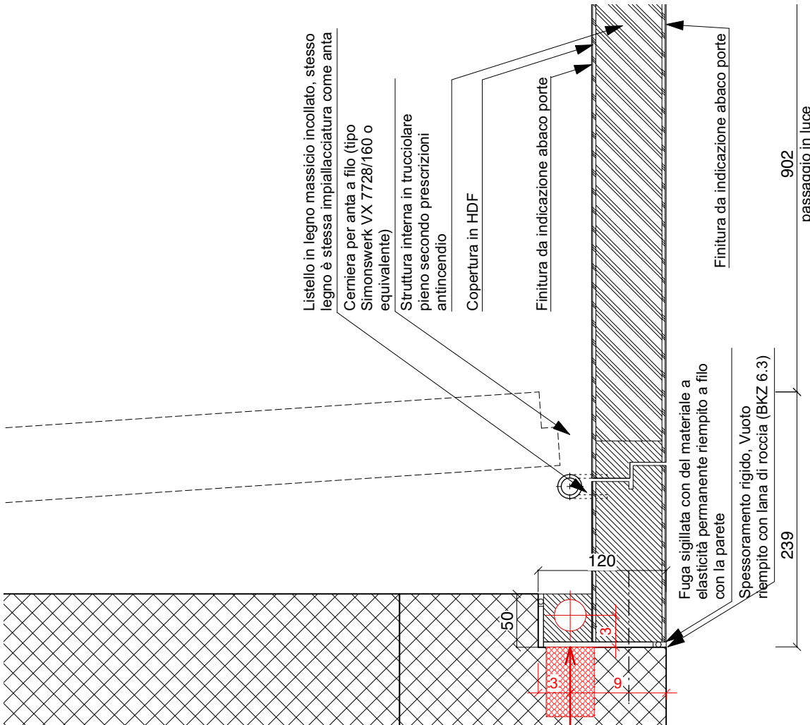
PIANTA DETTAGLIO 1:5
