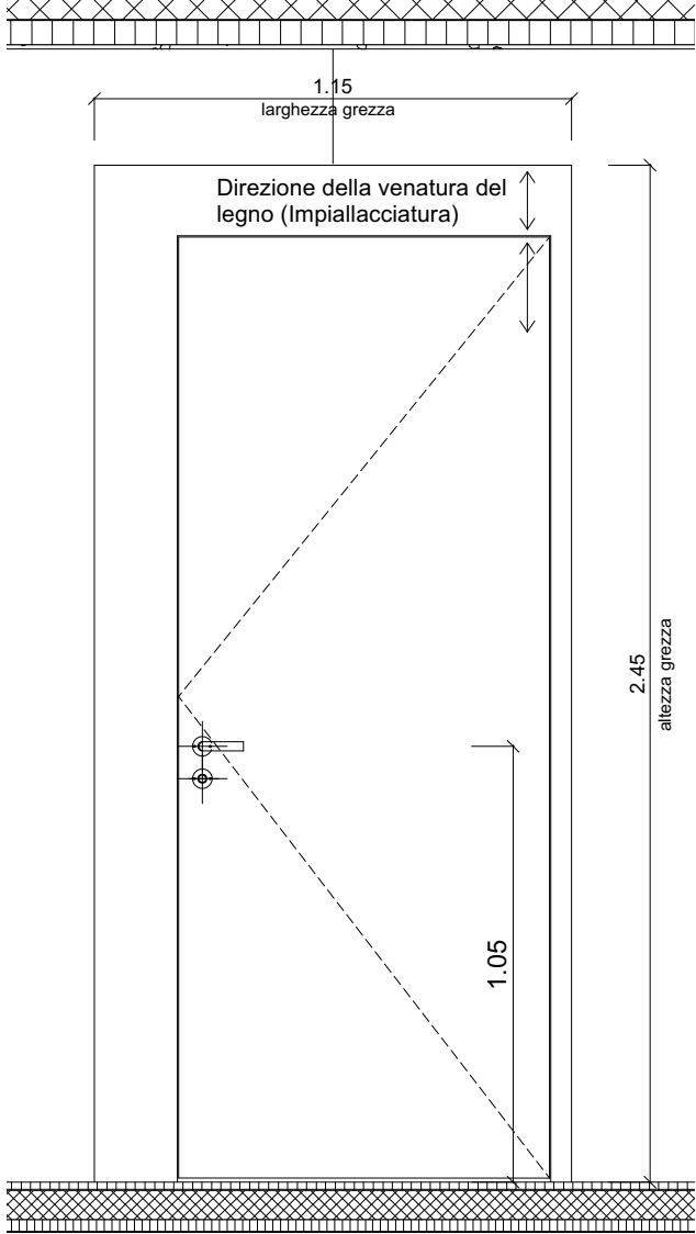
PROSPETTO INTERNO 1:20
