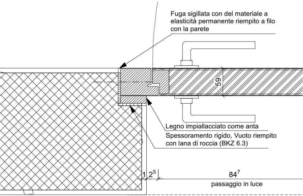
PIANTA DETTAGLIO 1:5
