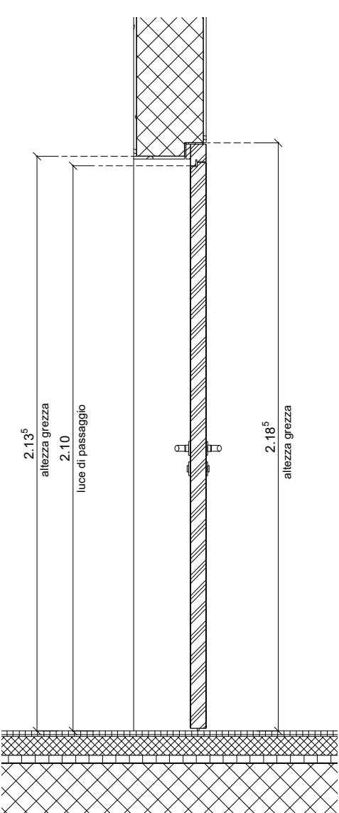
SEZIONE 1:20
