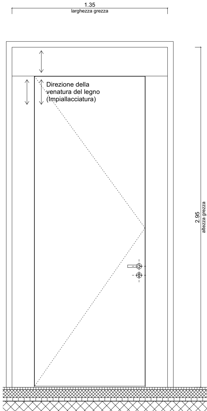
PROSPETTO ESTERNO 1:20
