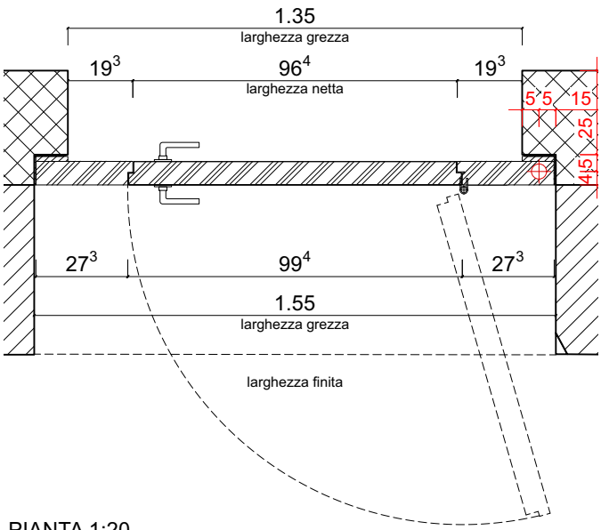
PIANTA 1:20
