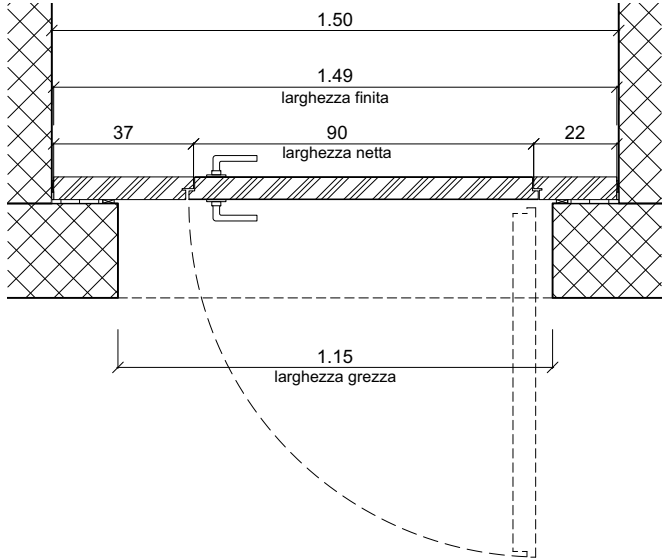
PIANTA 1:20
