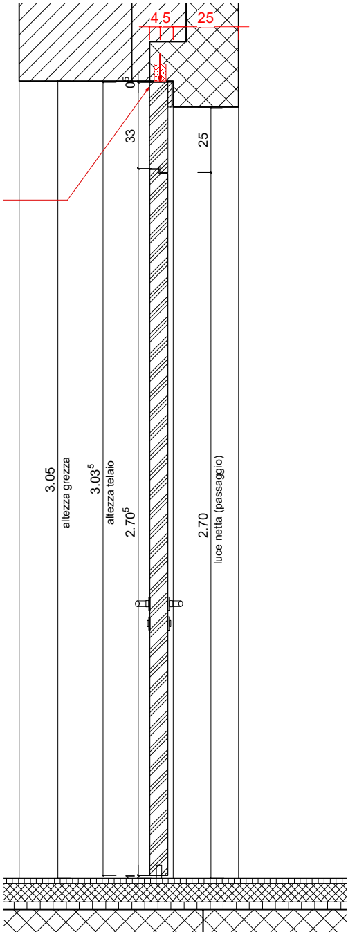
SEZIONE 1:20
