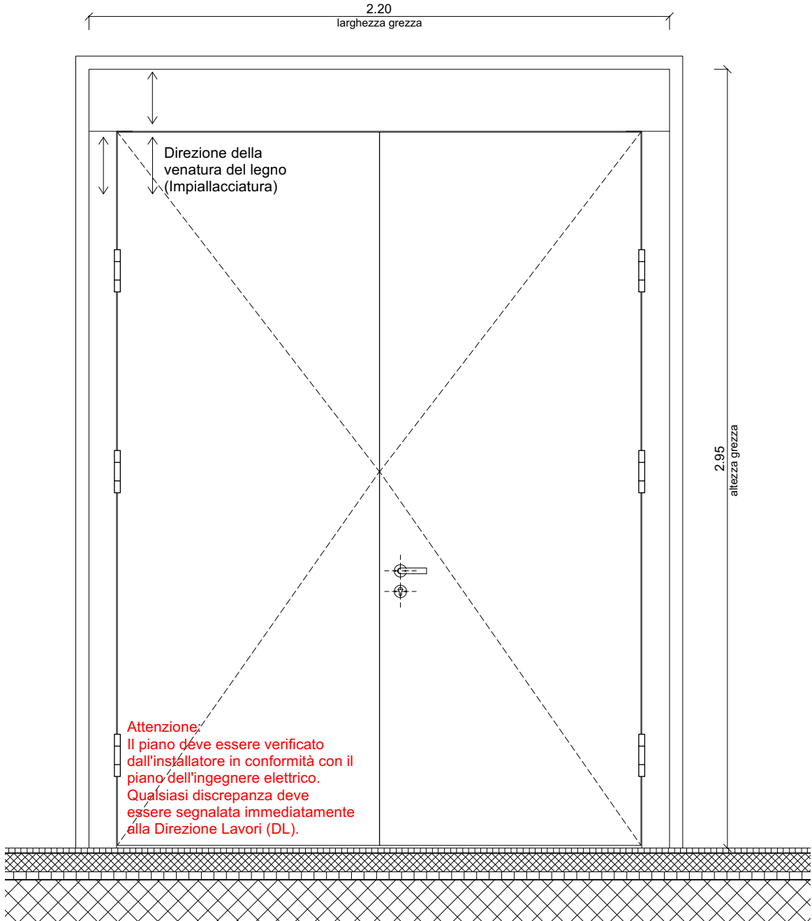
PROSPETTO INTERNO 1:20
