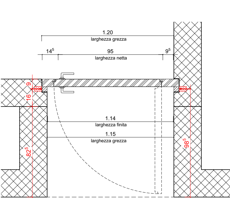
PIANTA 1:20
