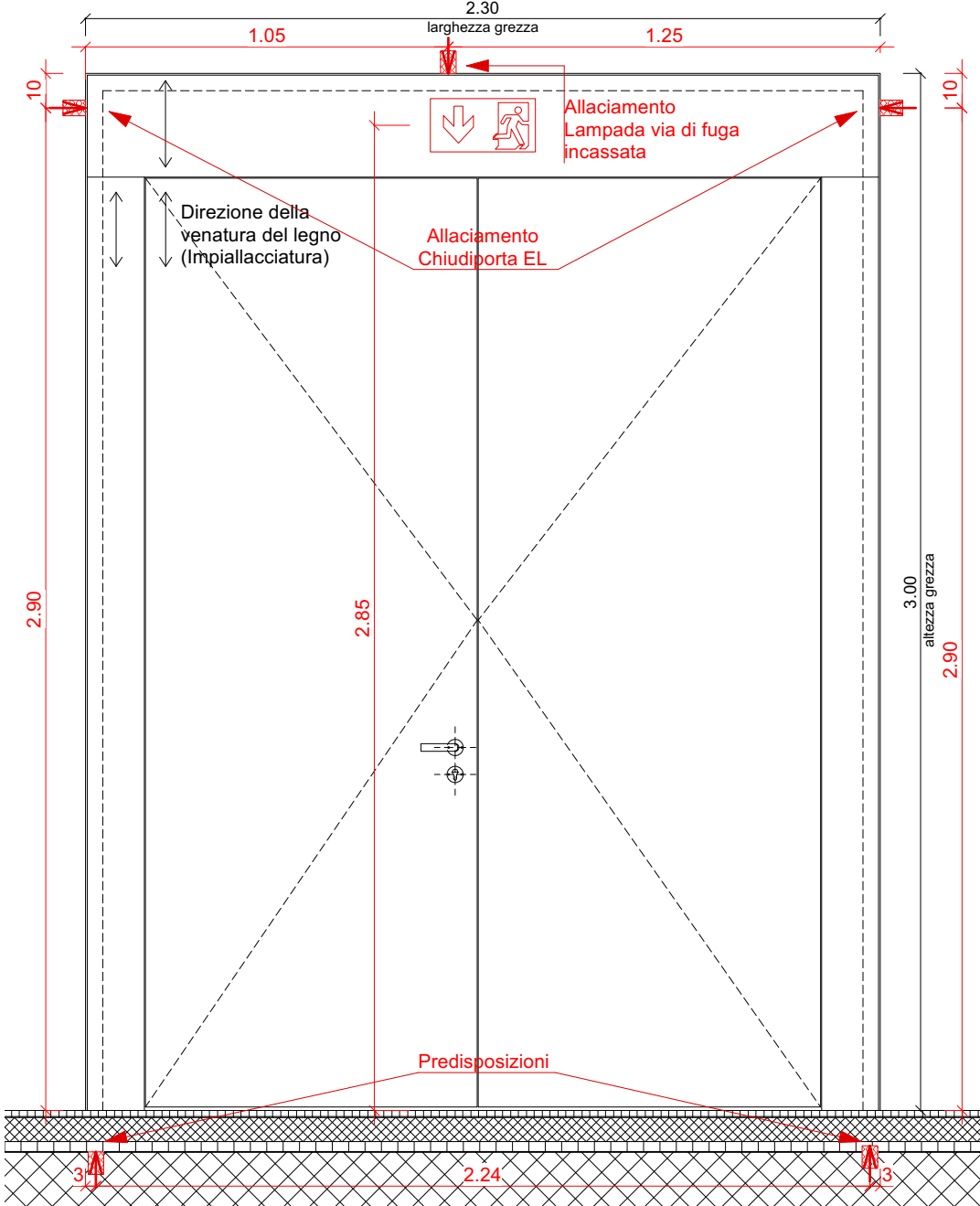
PROSPETTO ESTERNO 1:20
