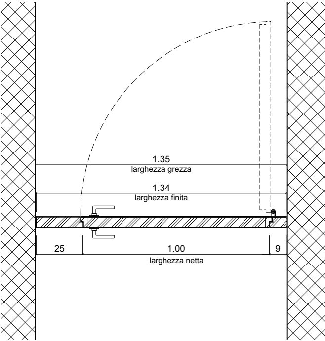
PIANTA 1:20
