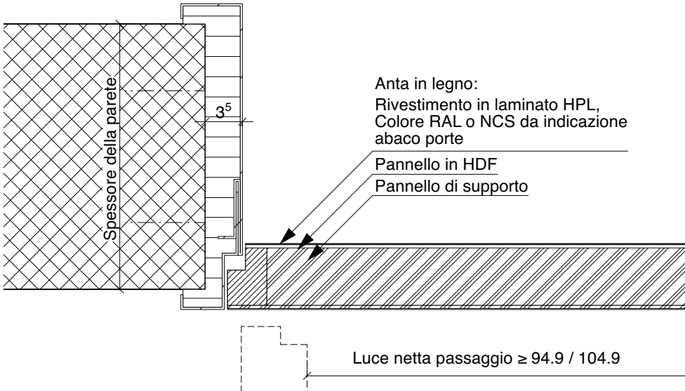
PIANTA DETTAGLIO 1:5
