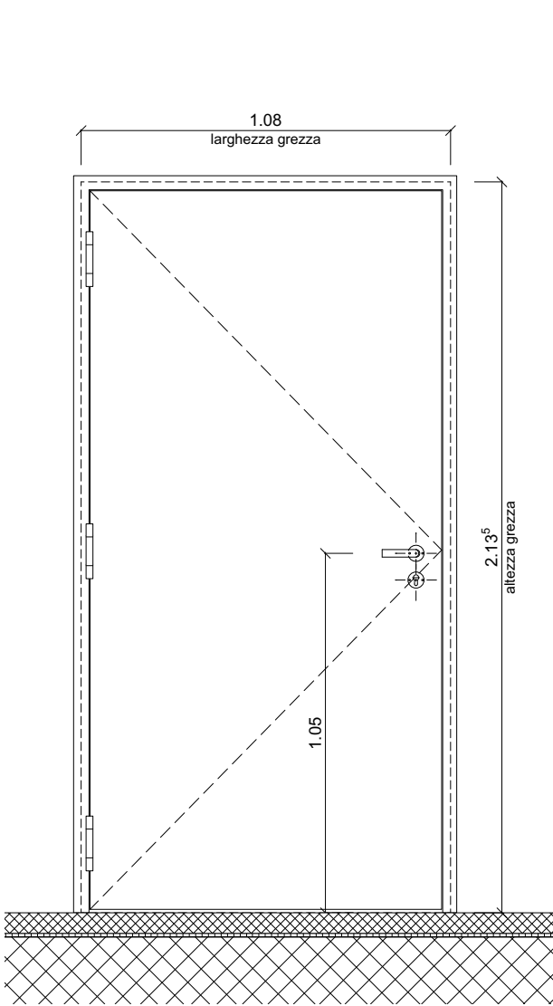
PROSPETTO ESTERNO 1:20
