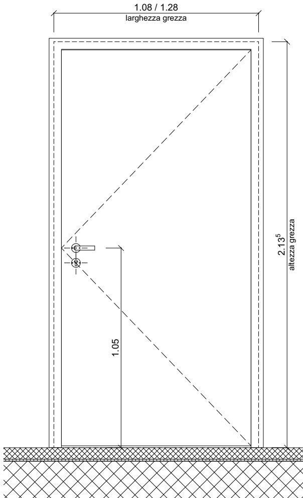
PROSPETTO INTERNO 1:20
