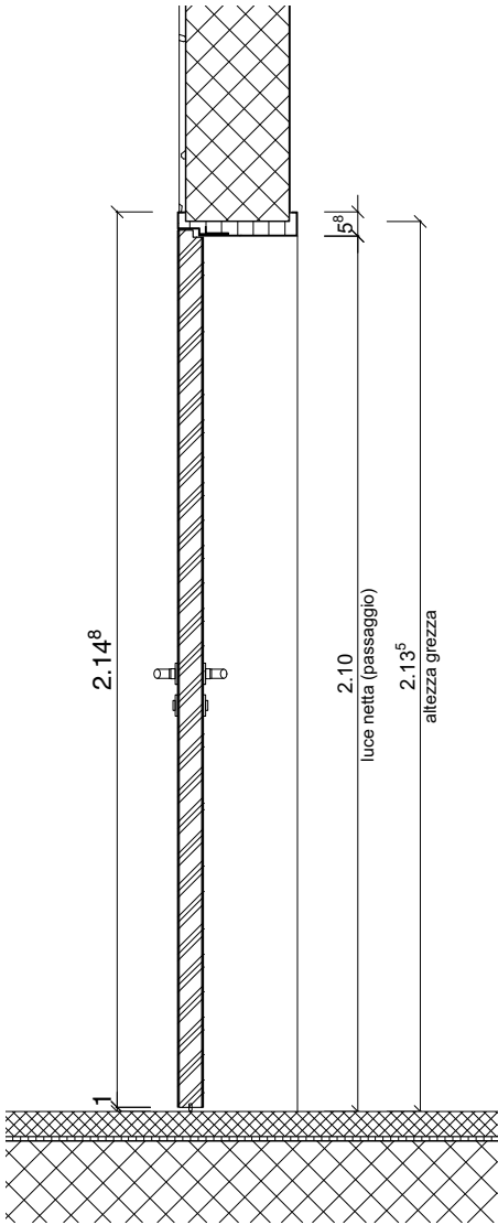
SEZIONE 1:20
