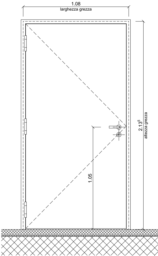
PROSPETTO ESTERNO 1:20
