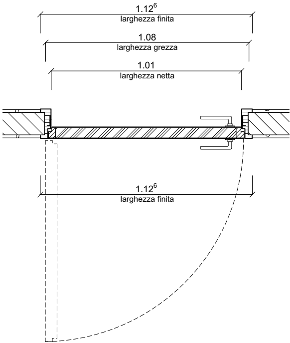
PIANTA 1:20
