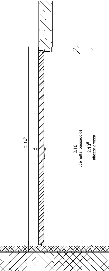
SEZIONE 1:20
