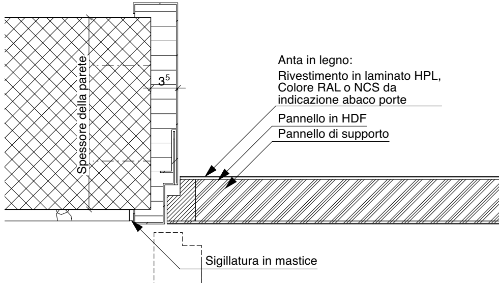
PIANTA DETTAGLIO 1:5
