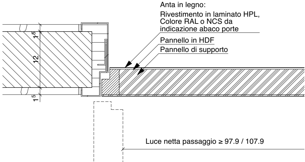
PIANTA DETTAGLIO 1:5
