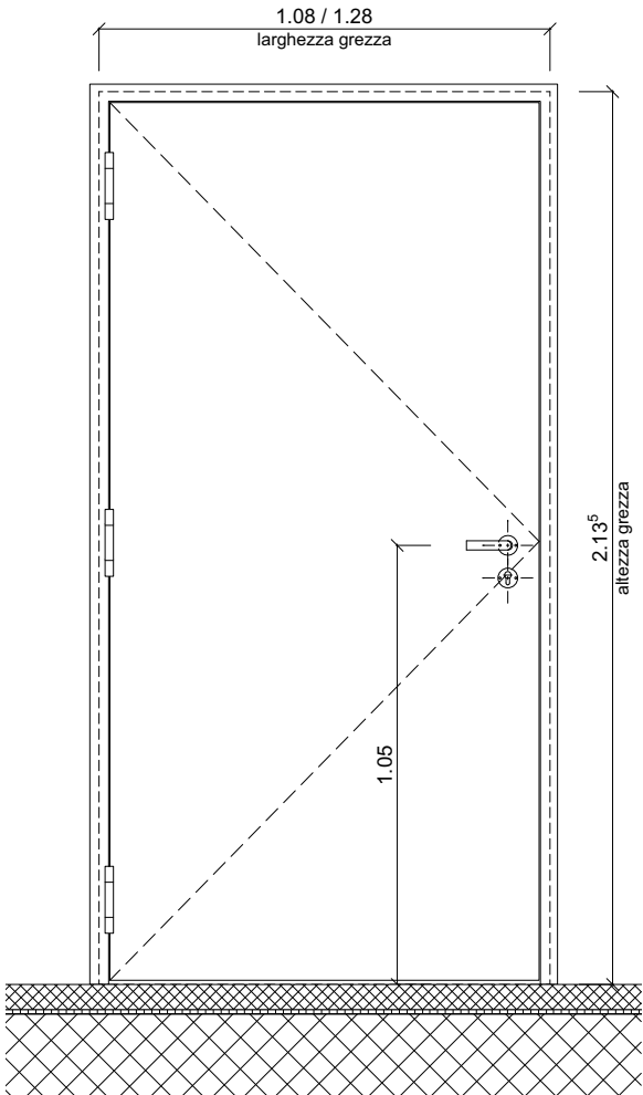
PROSPETTO ESTERNO 1:20
