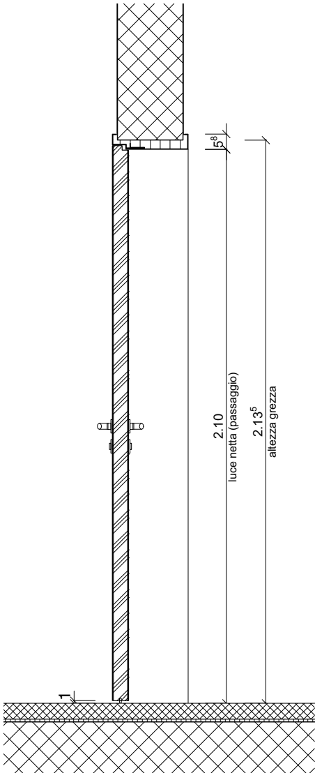
SEZIONE 1:20
