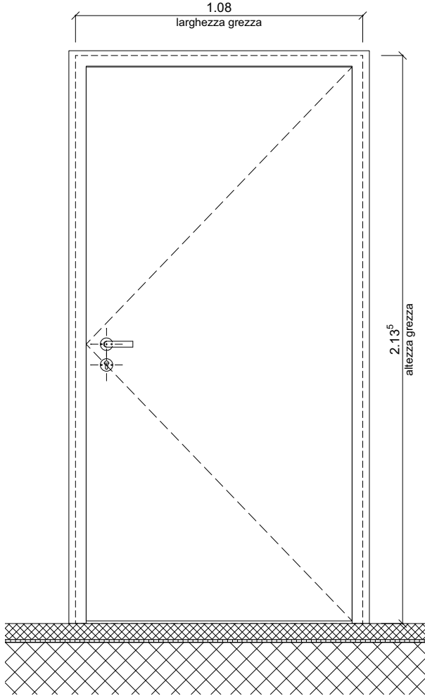
PROSPETTO INTERNO 1:20
