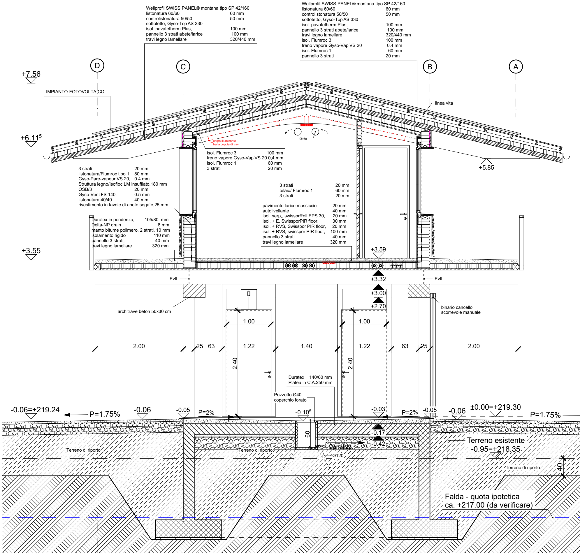
S-05, SEZIONE CORRIDOIO UFFICI
