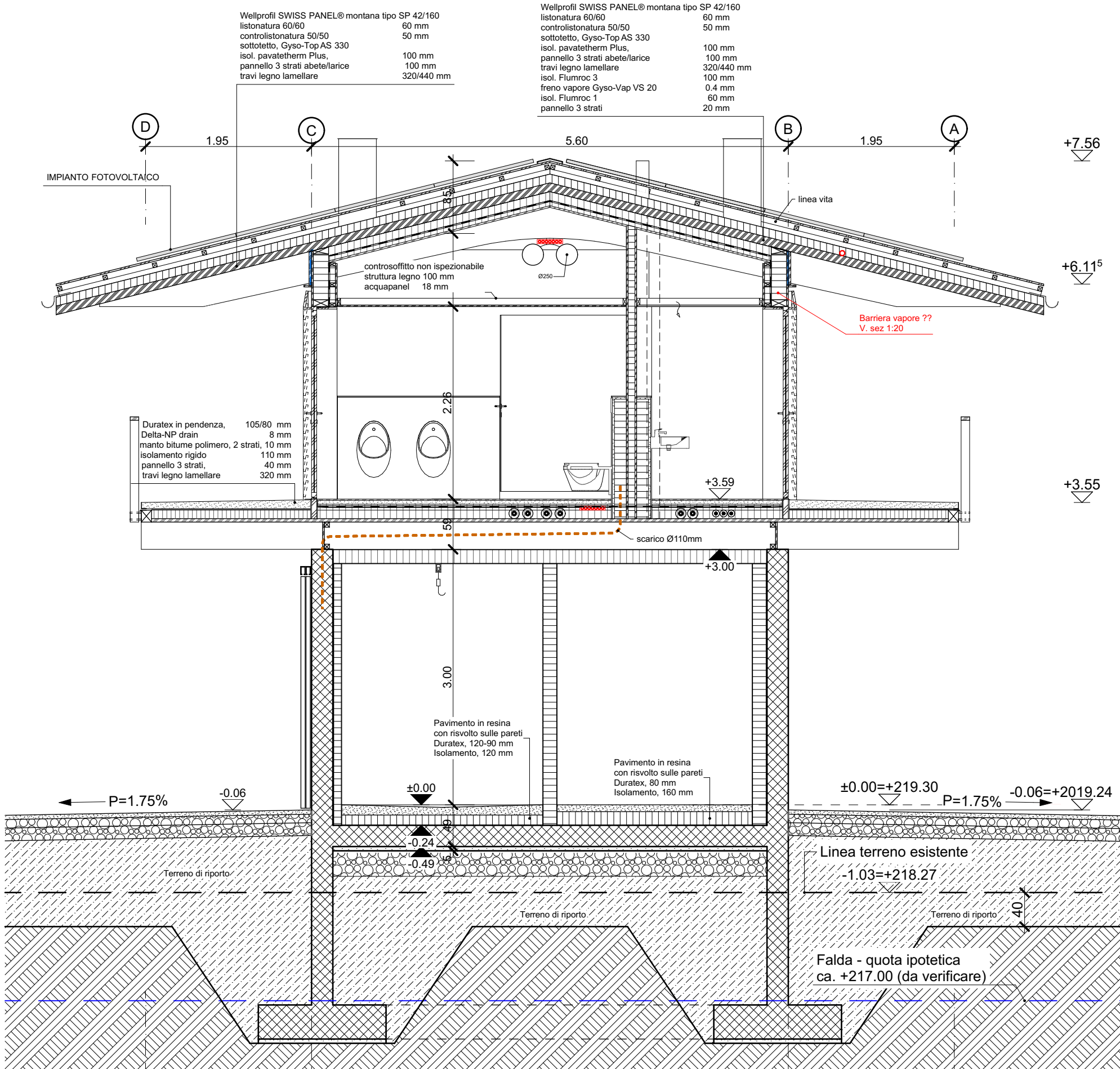
S-04, SEZIONE BAGNI / CELLE FRIGO
