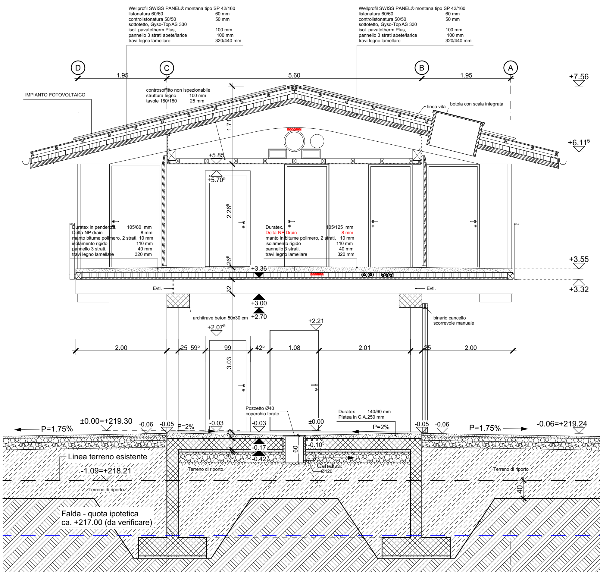
S-03, SEZIONE INGRESSO SALA
