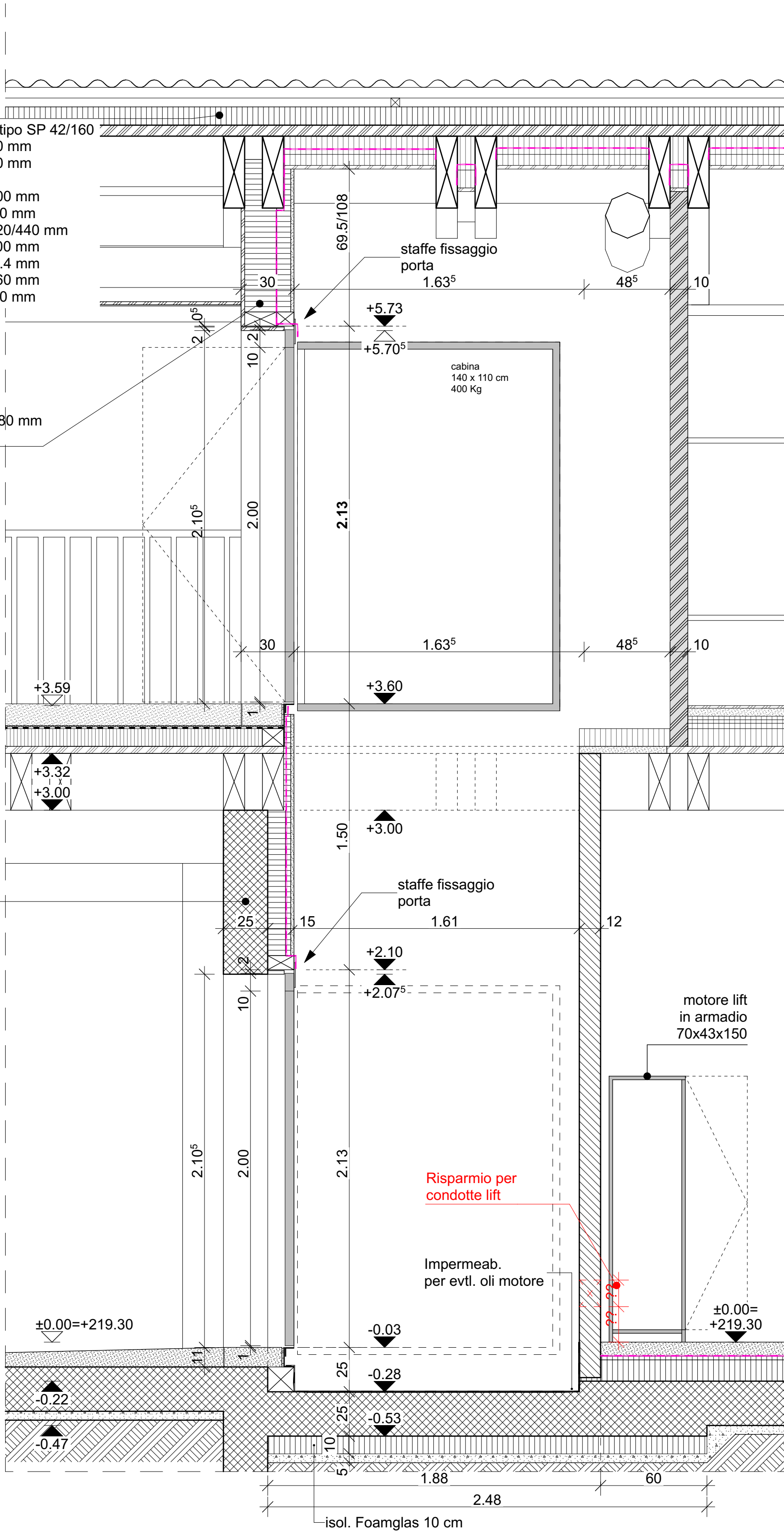
SEZIONE 2-2
