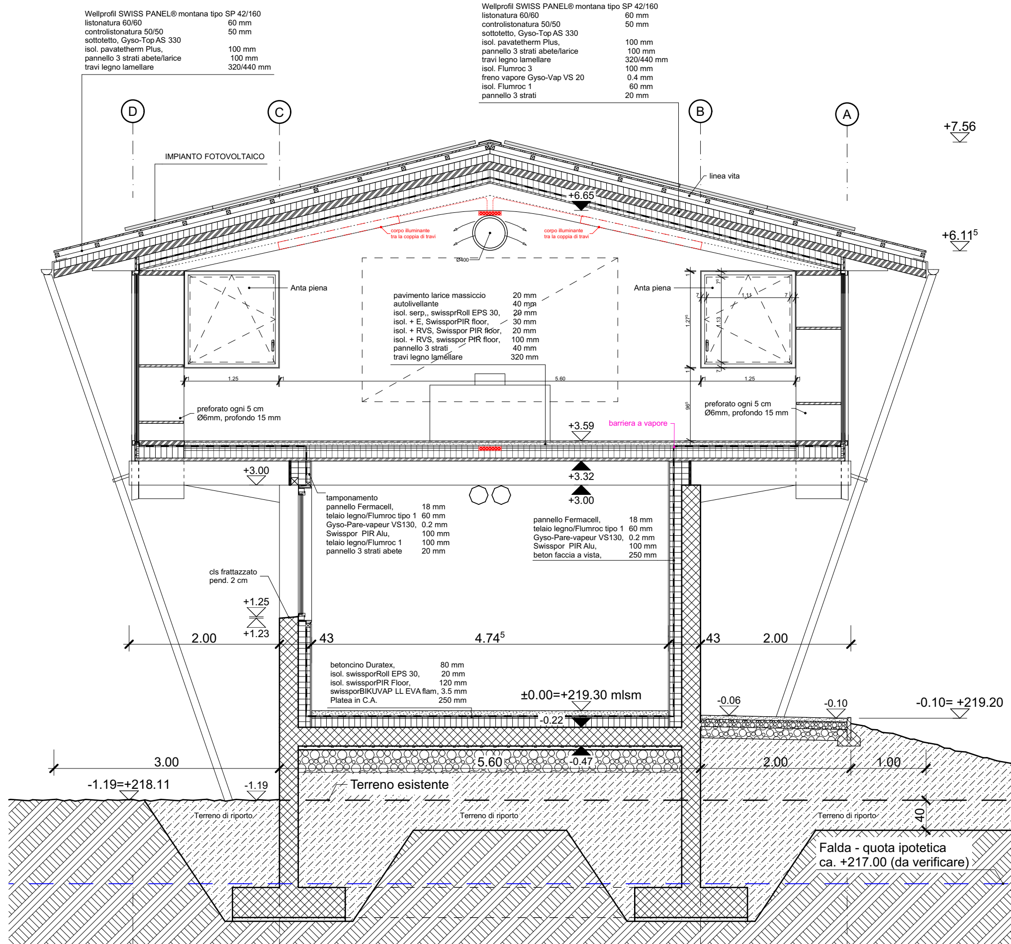
S-01, SEZIONE SALA
