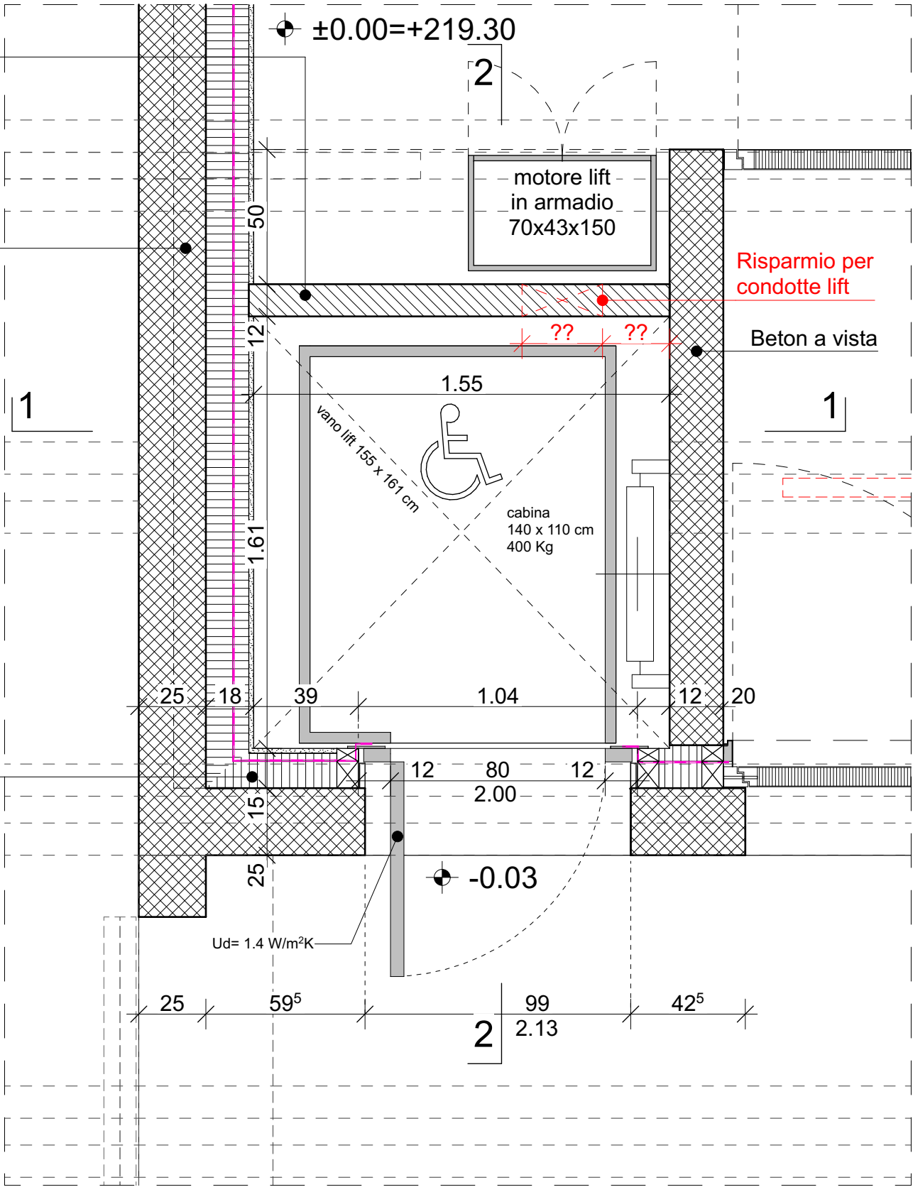
PIANTA PT
