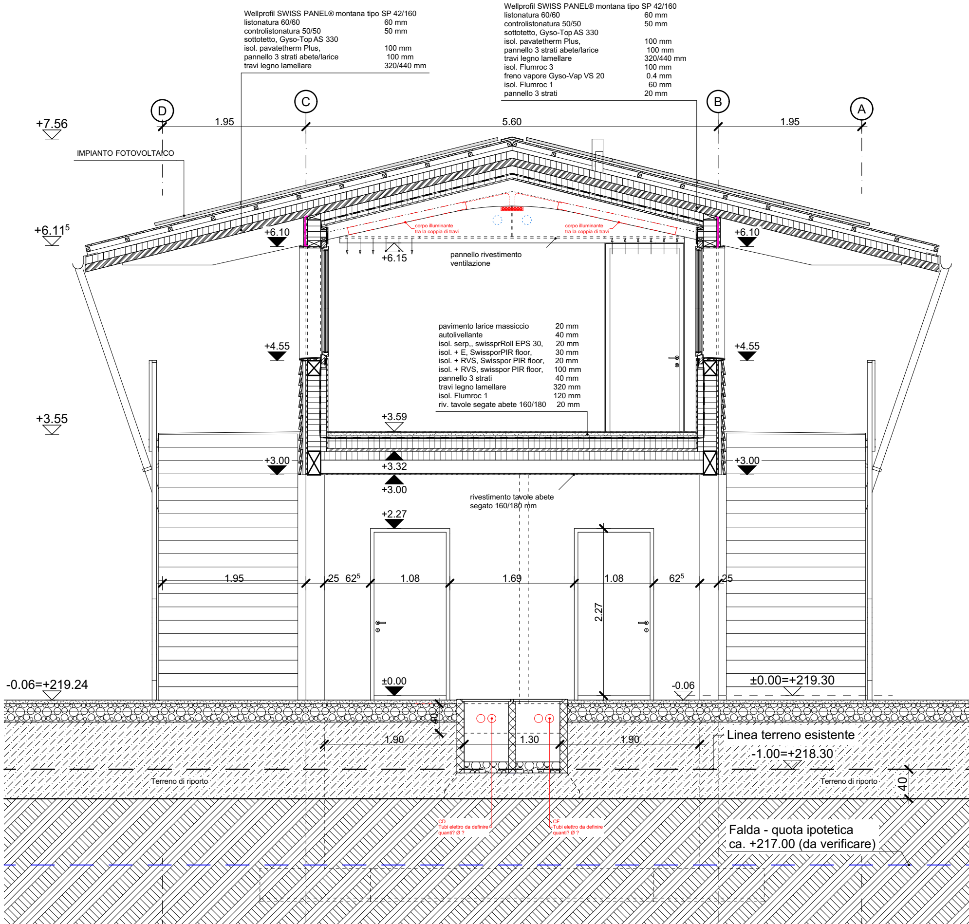
S-06, SEZIONE SBALZO
