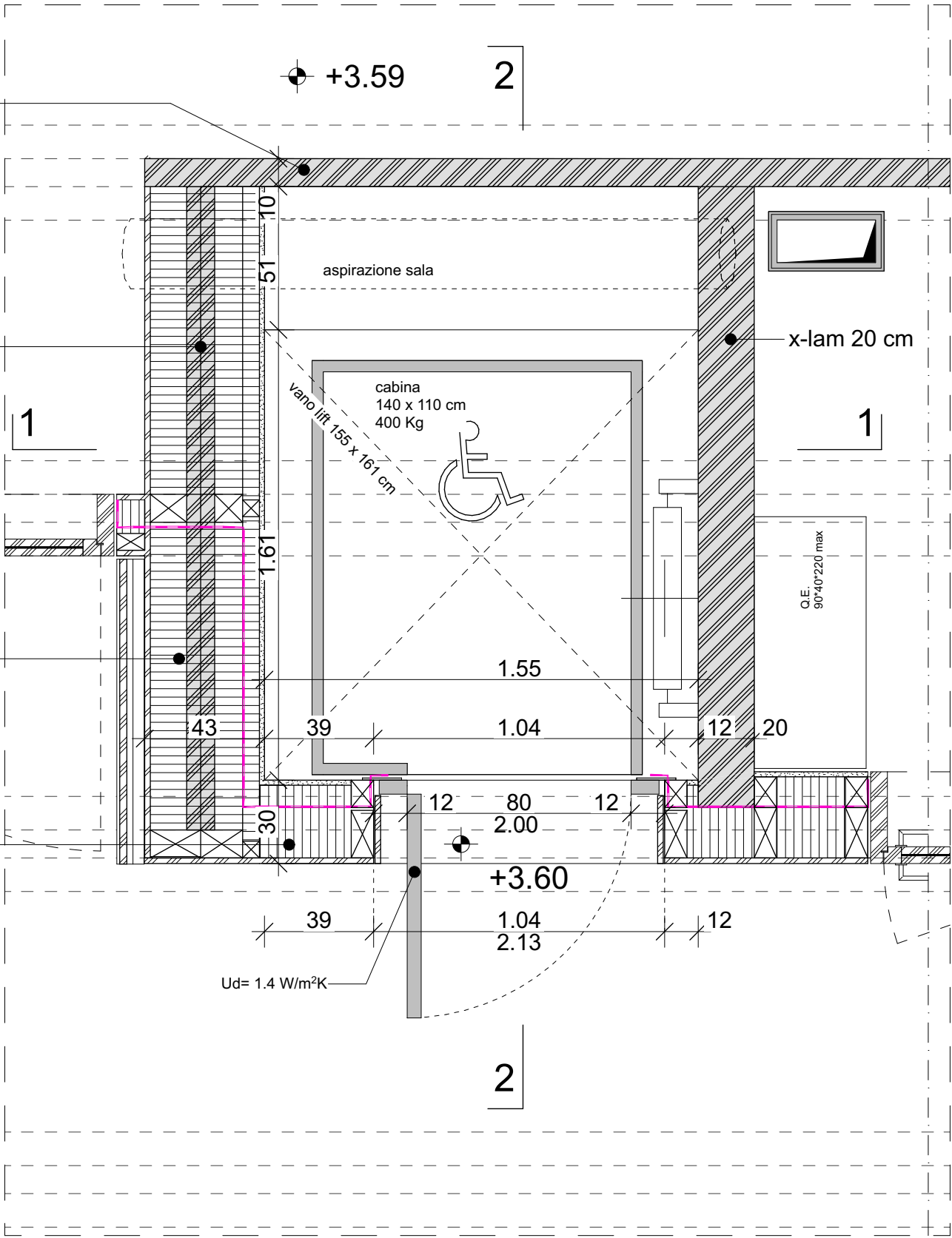
PIANTA 1°P
