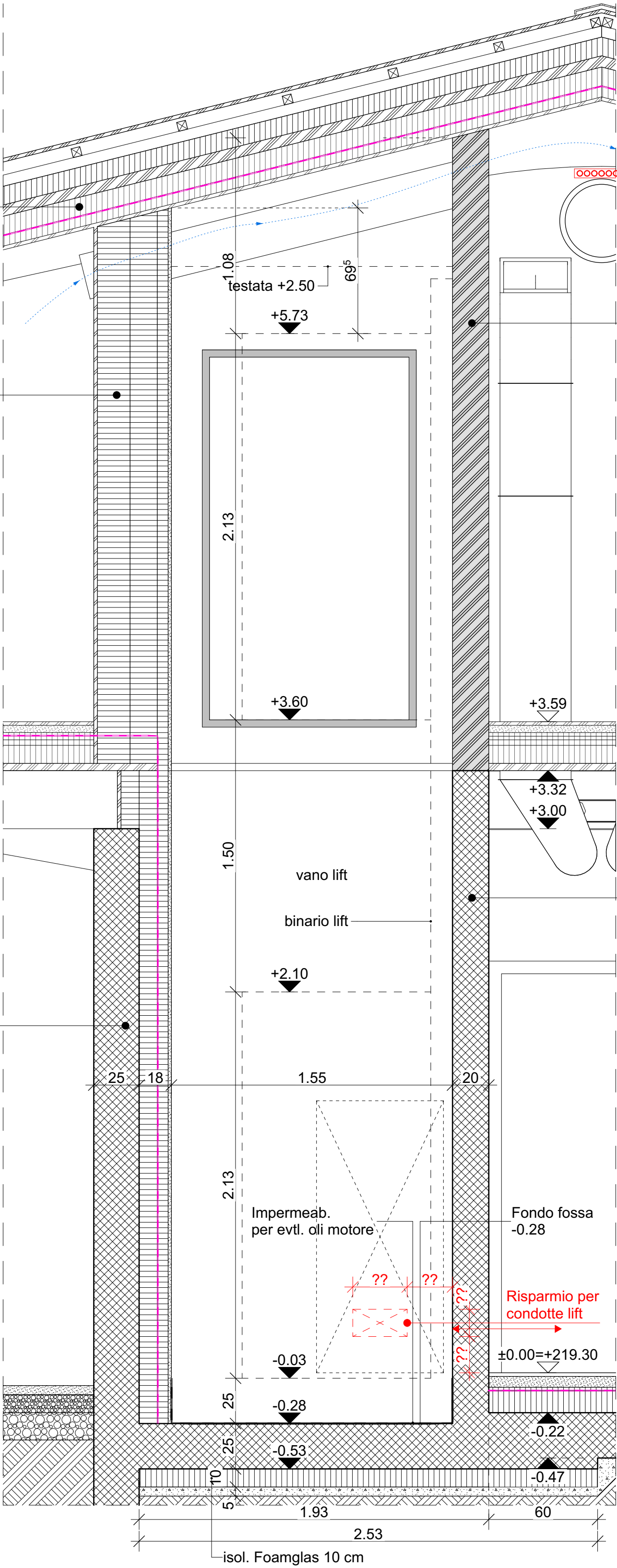
SEZIONE 1-1
