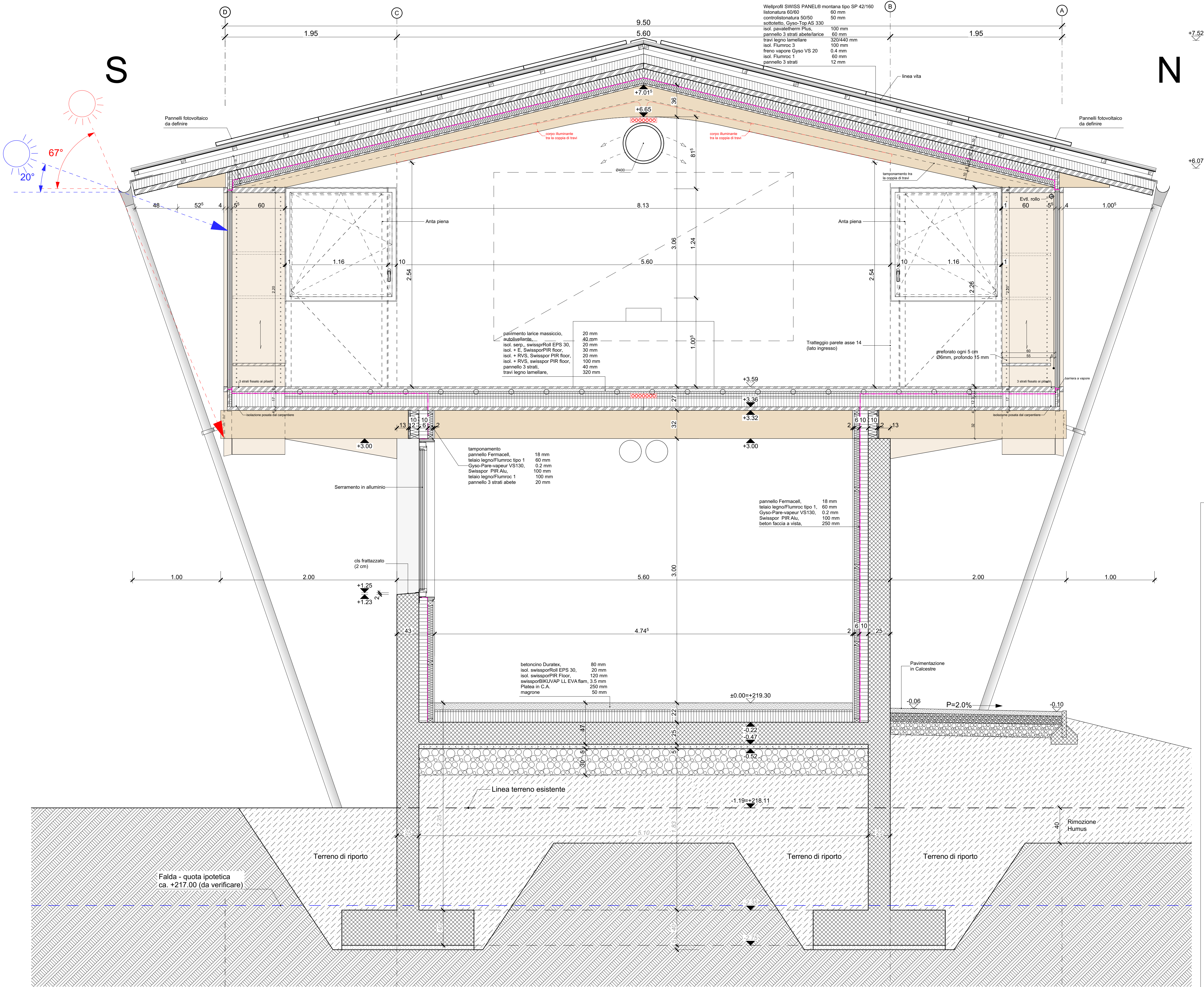
SEZIONE SALA
