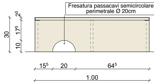
Vista Posteriore Cubo 4
