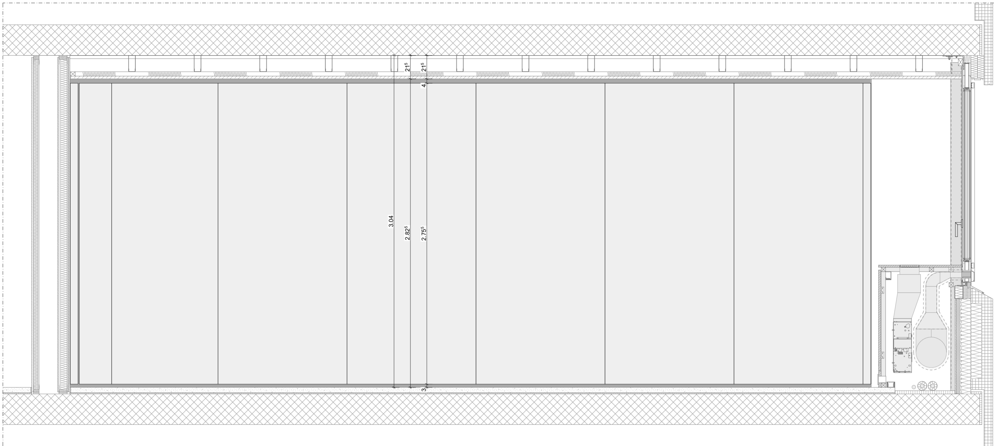
PROSPETTO, SCALA 1:20
