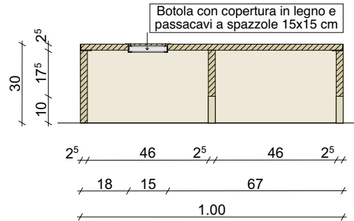
Sezione C-C Cubo 4
