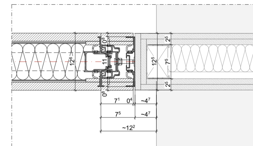
PIANTA, SCALA 1:5
