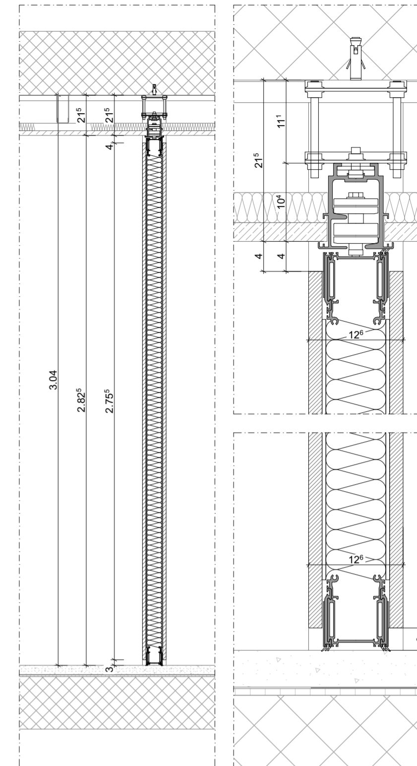
SEZIONE, SCALA 1:20
