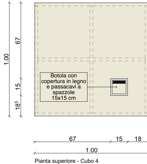
Pianta superiore - Cubo 4
