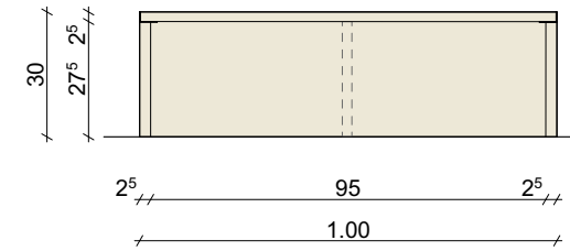
Vista laterale Cubo 4
