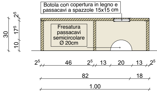
Sezione A-A Cubo 4
