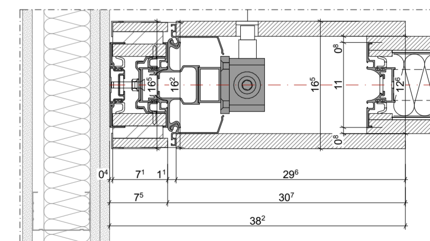
PIANTA, SCALA 1:5
