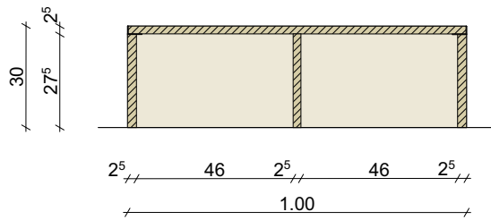
Sezione B-B Cubo 4
