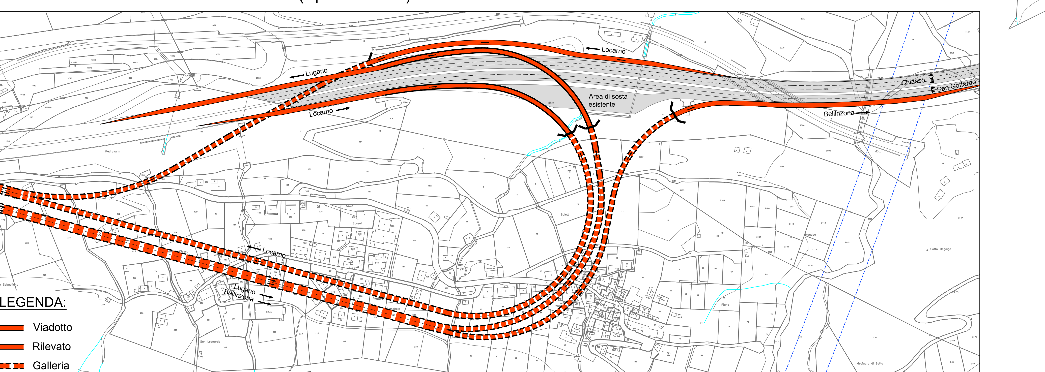
Diramazione A2-A13 in località al Motto (Vp = 60 Km/h) - 1:2000
