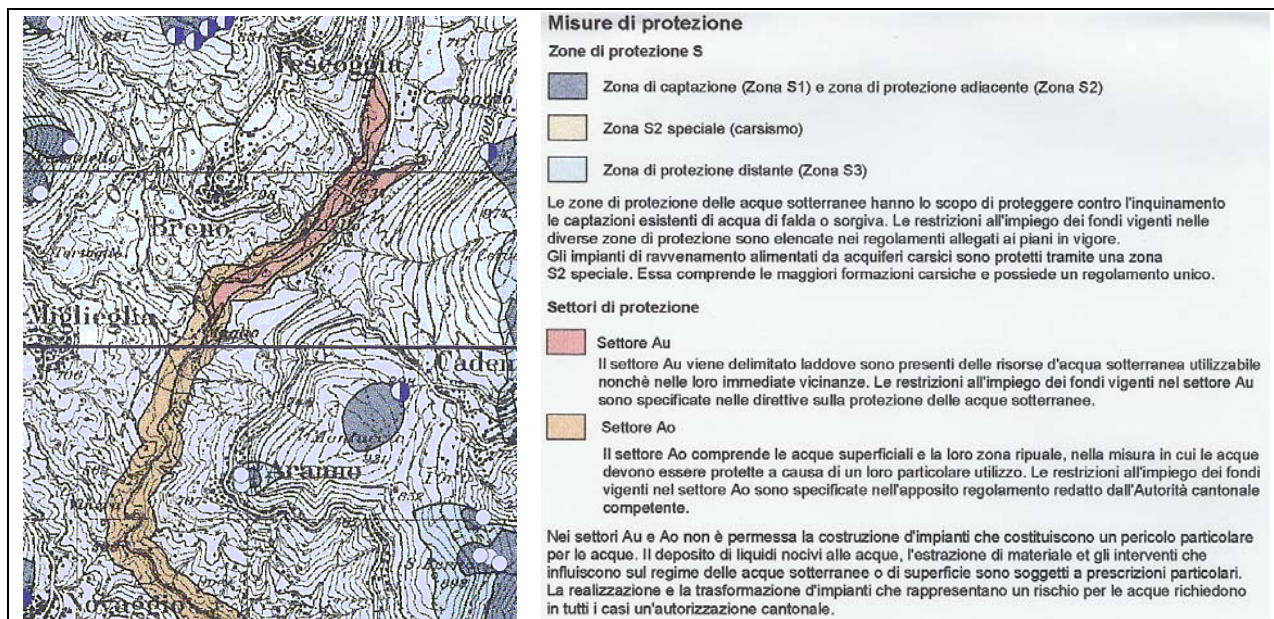
Figura 3: Settori e aree di protezione delle acque sotterranee e delle captazioni (IST 2003)
