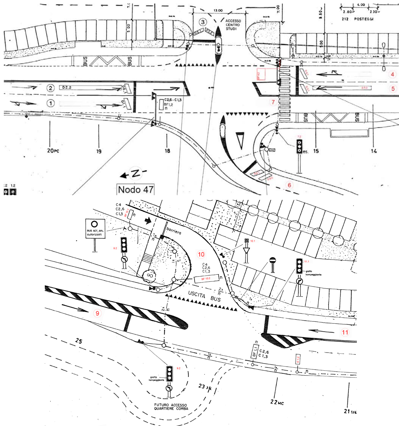
Figura 53: estratto del piano semaforico – nodo 47
