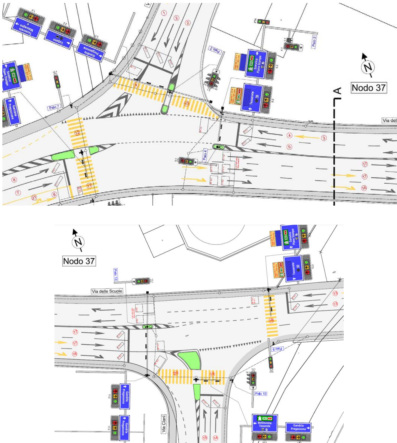
Figura 51: estratto del piano semaforico - nodo 37
