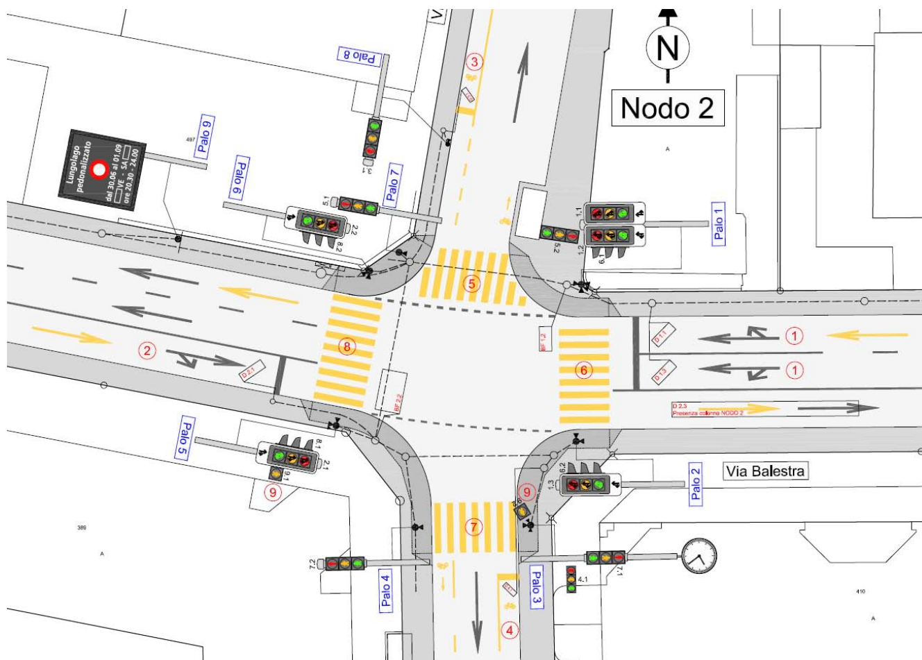
Figura 18: estratto del piano semaforico - nodo 2
