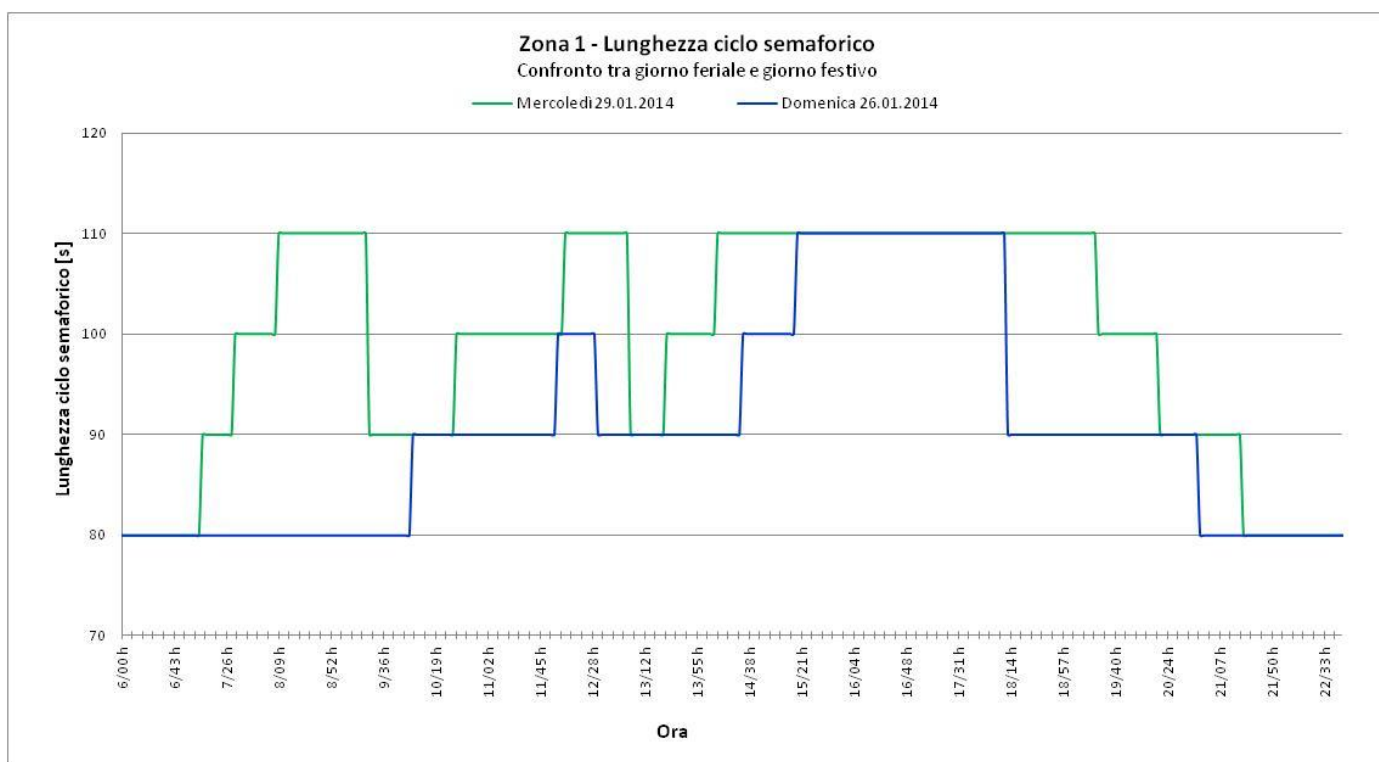
Figura 6: ZONA 1 – Confronto lunghezza ciclo semaforico – giorno feriale e giorno festivo
