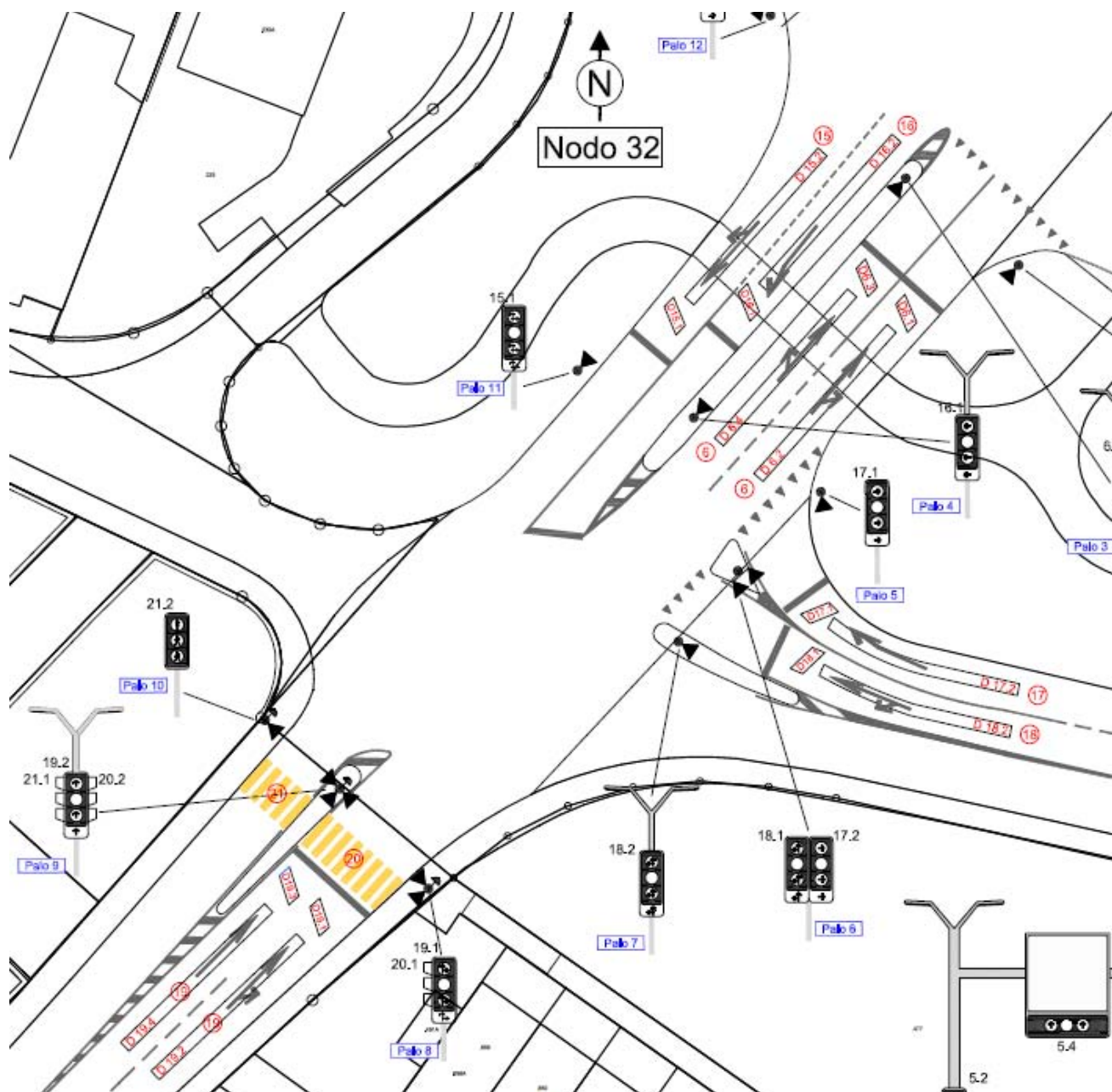
Figura 70: estratto del piano semaforico - nodo 32
