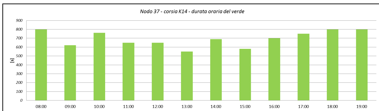
Figura 45: Nodo 37 – durata oraria del tempo di verde - corsia K14
