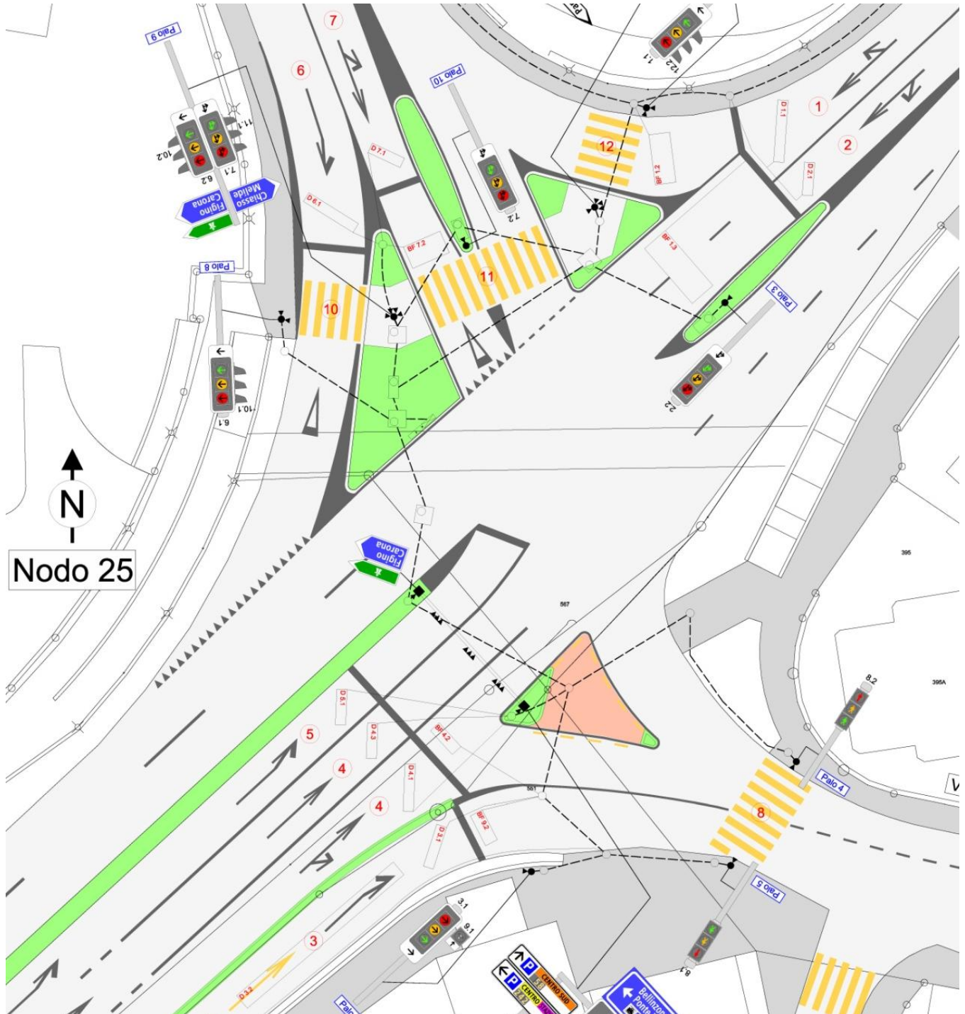
Figura 88: estratto del piano semaforico - nodo 25
