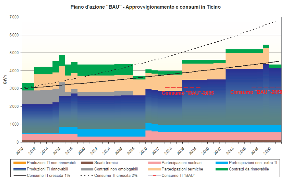
Figura 38 Approvvigionamento elettrico secondo il piano d'azione BAU. In rosso sono evidenziati i consumi previsti dal piano d'azione BAU al 2035 e al 2050. Quale ulteriore riferimento, in nero (linea continua e linea tratteggiata) sono riportate le stime di crescita tendenziale dei consumi (incremento 1%-2% anno).
