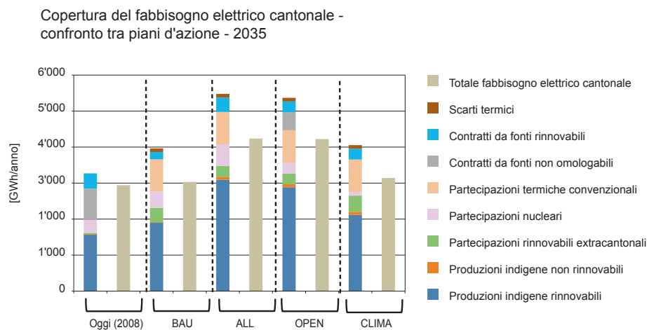
Figura 52 Copertura del fabbisogno elettrico cantonale secondo i quattro piani d'azione al 2035, a confronto con la situazione attuale (2008).
