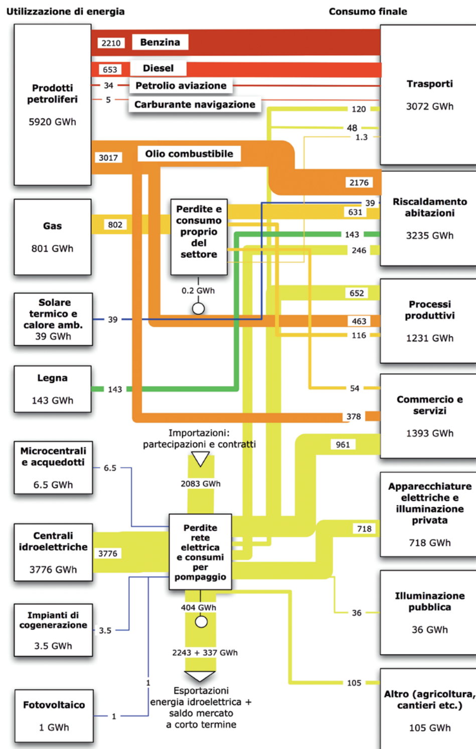
Figura 6 Il bilancio energetico cantonale (anno 2008).
