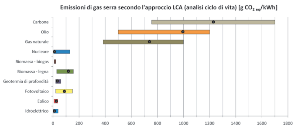
Figura 29 Stime di emissione di gas serra [gCO 2 eq/kWh] per le principali tecnologie di produzione di energia elettrica, desunte dall'analisi di rassegne internazionali
