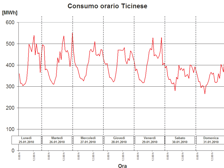
Figura 32 Esempio di curve di carico giornaliero per il Cantone Ticino su base oraria (consumo orario), registrata nella settimana dal 25 al 31 gennaio 2010 Fonte: AET.
