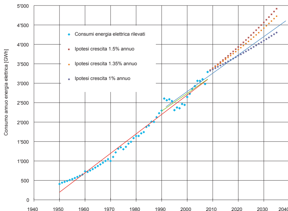
Figura 30 Previsioni d'evoluzione dei consumi di energia elettrica, in assenza di misure di politica energetica (evoluzione «spontanea» del sistema elettrico).
