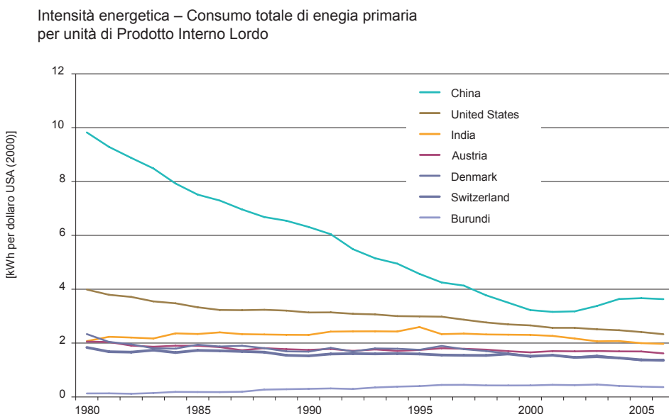
Figura 26 Andamento dell'intensità energetica (kWh per dollaro USA 2000) Fonte: US DOE/Energy Information Administration, International Energy Annual 2006.
