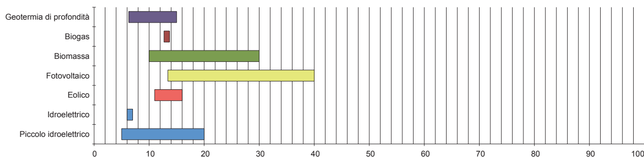
Stima del costo di produzione del kWh elettrico [cts CHF/kWh] - anni 2035/2050
