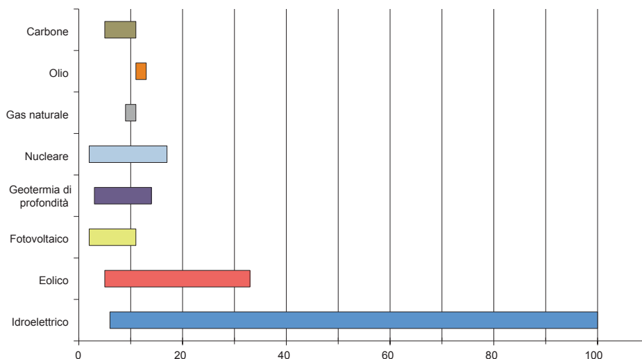
Figura 28 Stime dell'indice EROI per le principali tecnologie di produzione di energia elettrica, desunte dall'analisi di rassegne internazionali Fonti: Murphy et Hall, 2010, Kubiszewski et al., 2010.
