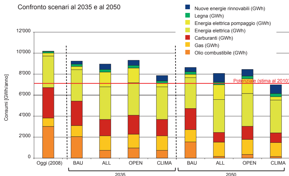
Figura 46 Consumi di energia, secondo gli scenari determinati dai quattro piani d'azione, a confronto con la situazione attuale (anno 2008).
