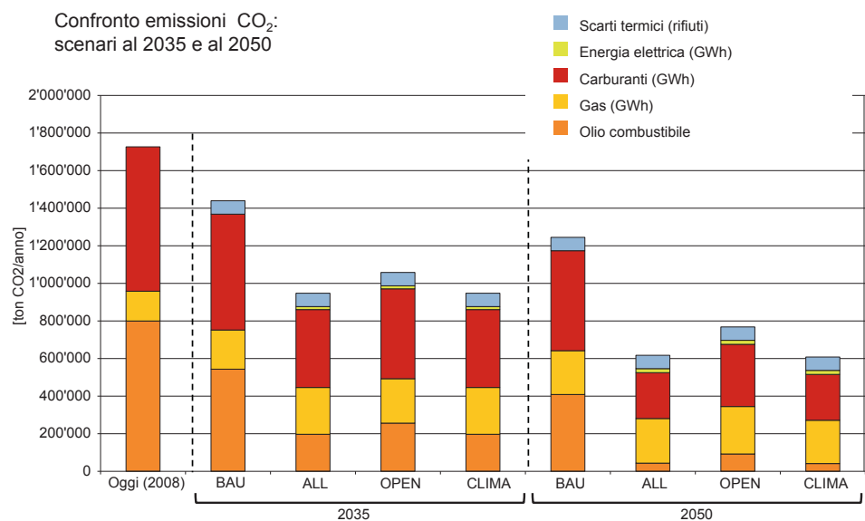
Figura 51 Emissioni di CO 2 prodotte sul territorio cantonale secondo gli scenari determinati dai quattro piani d'azione, a confronto con la situazione attuale (anno 2008).
