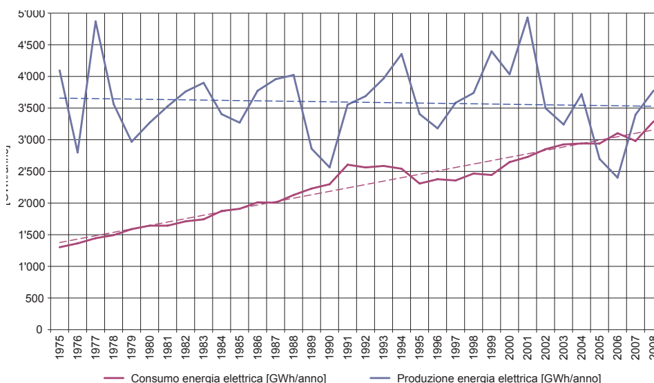
Figura 7 Confronto tra la produzione e il consumo di energia elettrica sul territorio cantonale. Sono tratteggiate le linee di tendenza sull'intero periodo 1975-2008.
