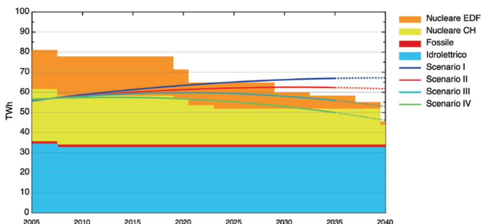
Figura 33 Produzione (superficie colorate) e consumo (curve colorate) di energia elettrica sul piano svizzero secondo quattro scenari di sviluppo [1 TWh = 1'000 GWh] Fonte: «Perspectives énergétiques 2035: Management Summary», Dipartimento federale dell'ambiente, dei trasporti, dell'energia e delle comunicazioni DATEC, 2007.
