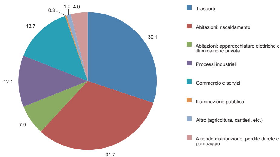
Consumi totali 2008, per settore [%]
