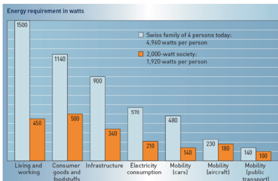
Figura 24 Articolazione del fabbisogno medio di energia primaria pro-capite nella Società 2000 watt. Fonte: «Smarter living», Novatantis, 2005.
