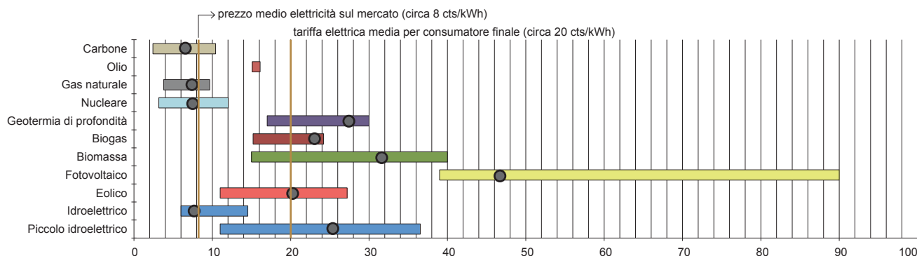
Stima del costo di produzione del kWh elettrico [cts CHF/kWh] - anni 2000/2008
