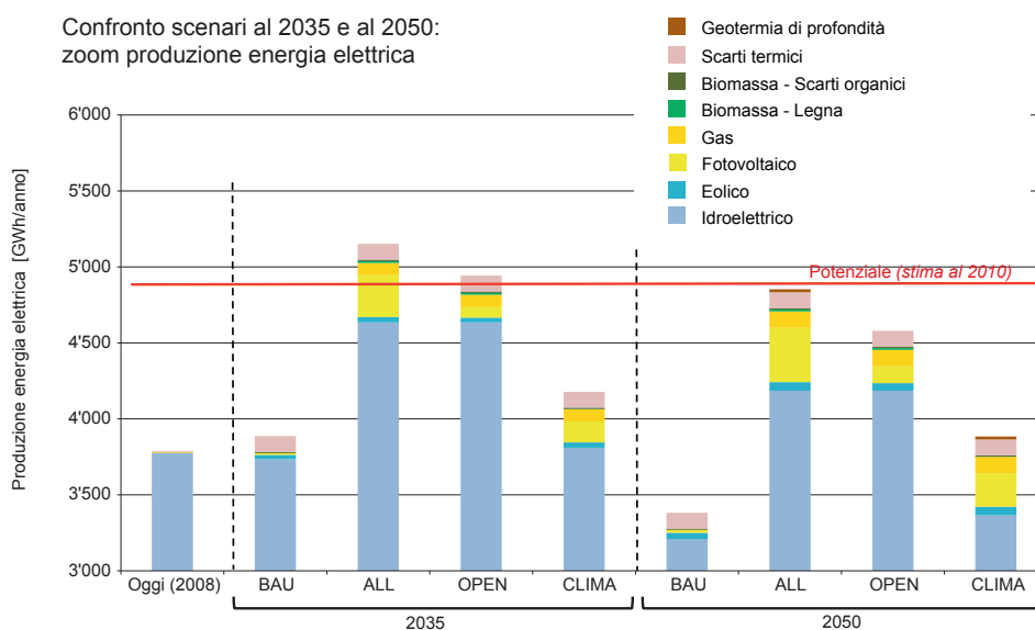
Figura 50 Produzione di energia elettrica sul territorio cantonale secondo gli scenari determinati dai quattro piani d'azione, a confronto con la situazione attuale (anno 2008). Zoom sui valori di produzione compresi tra 3'000 e 6'000 GWh/anno, volto ad evidenziare il contributo delle nuove fonti rinnovabili.
