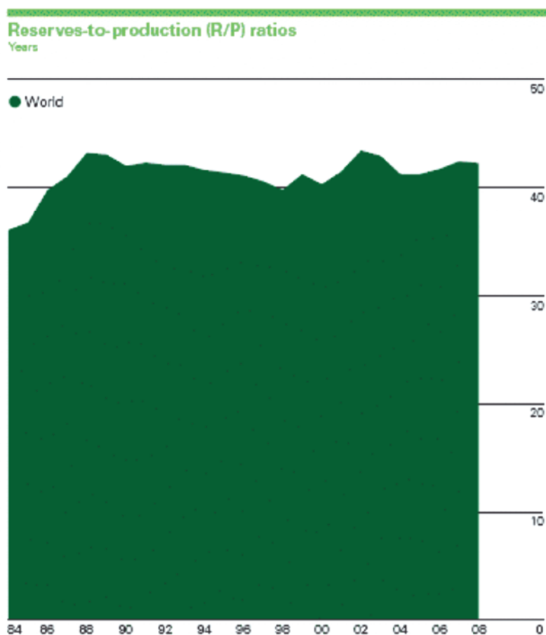
Figura 14 L'andamento del rapporto R/P (riserve/produzione) per il petrolio secondo la British Petroleum Fonte: BP Statistical review of world energy, 2009.
