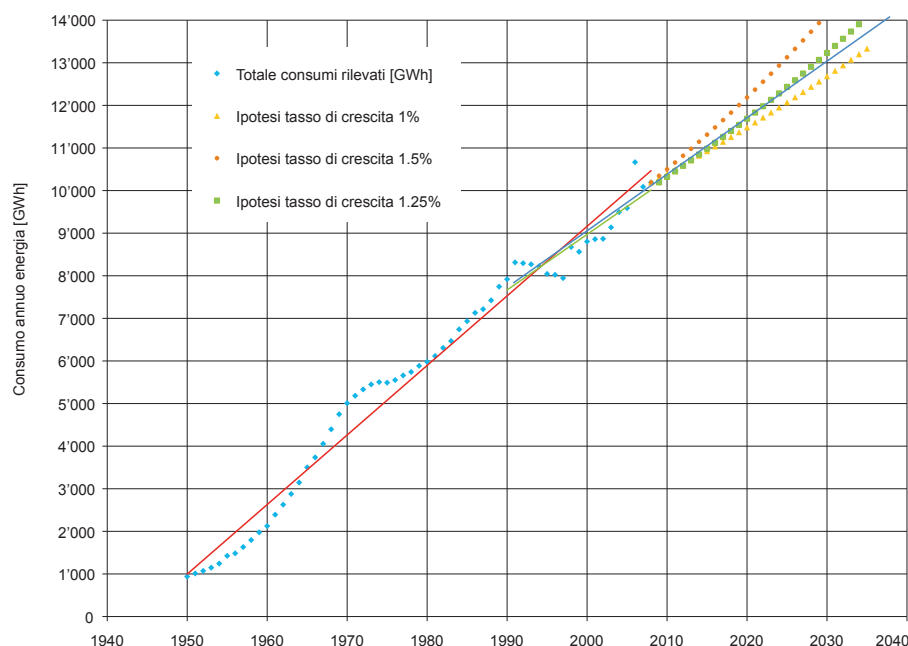
Figura 12 Previsioni d'evoluzione dei consumi energetici (evoluzione «spontanea» del sistema).
