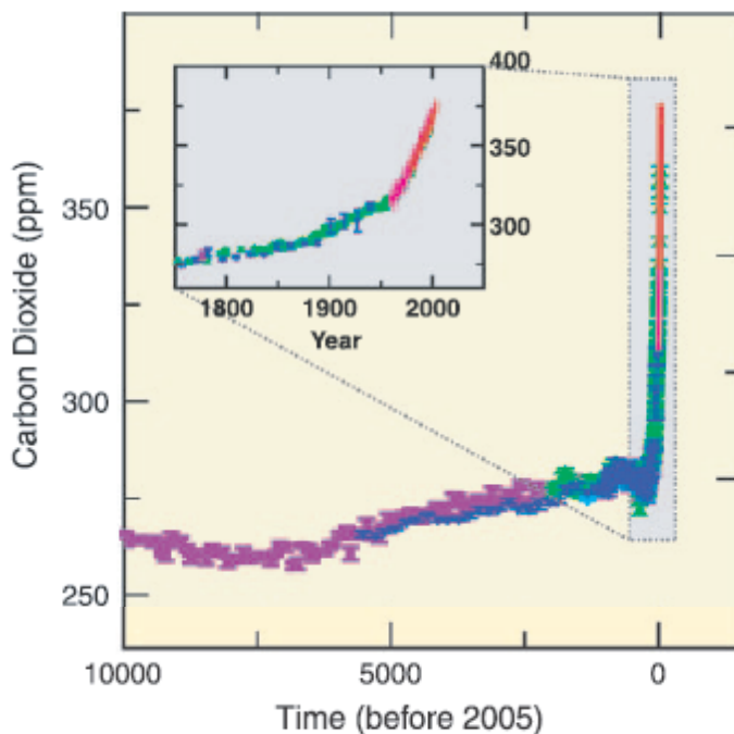
Figura 20 Concentrazione atmosferica di CO 2 registrata nel corso degli ultimi 10'000 anni. L'ingrandimento riporta l'andamento a partire dal 1750.
