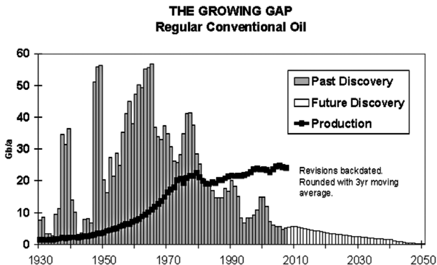
Figura 15 Confronto tra le riserve scoperte ogni anno («past discoveries») e la produzione annua di petrolio. Il grafico riporta anche una previsione delle scoperte annue per il futuro («future discoveries»). [Unità di misura Gb/a = milioni di barili all'anno] Fonte: ASPO Newsletter 100, 2009.
