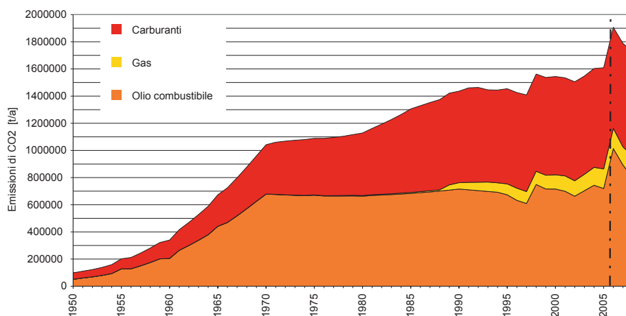
Figura 9 Andamento delle emissioni di CO 2 prodotte sul territorio cantonale, dal 1950. La retta tratteggiata indica l'anno (2006) a partire dal quale sono stati utilizzati modelli di calcolo dei consumi energetici differenti rispetto agli anni precedenti.
